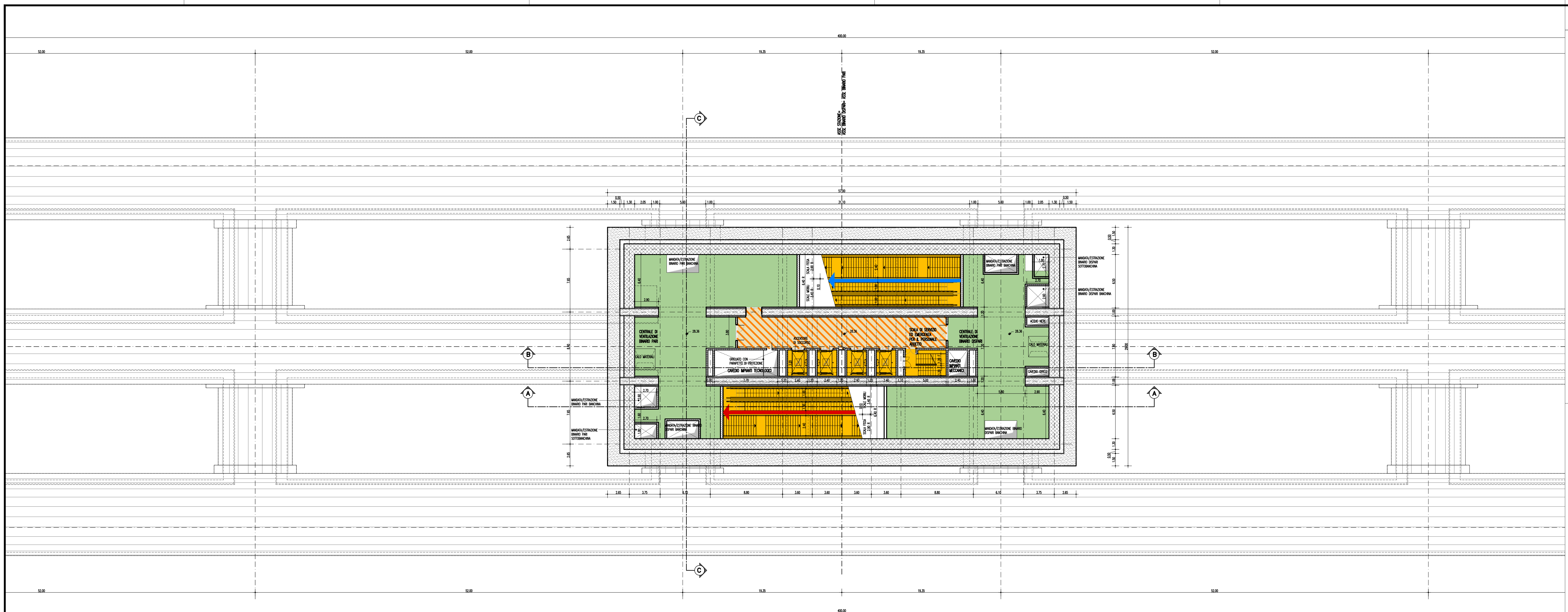
STAZIONE EUROPA – PIANTA PIANO PRIMO LIVELLO TECNICO
