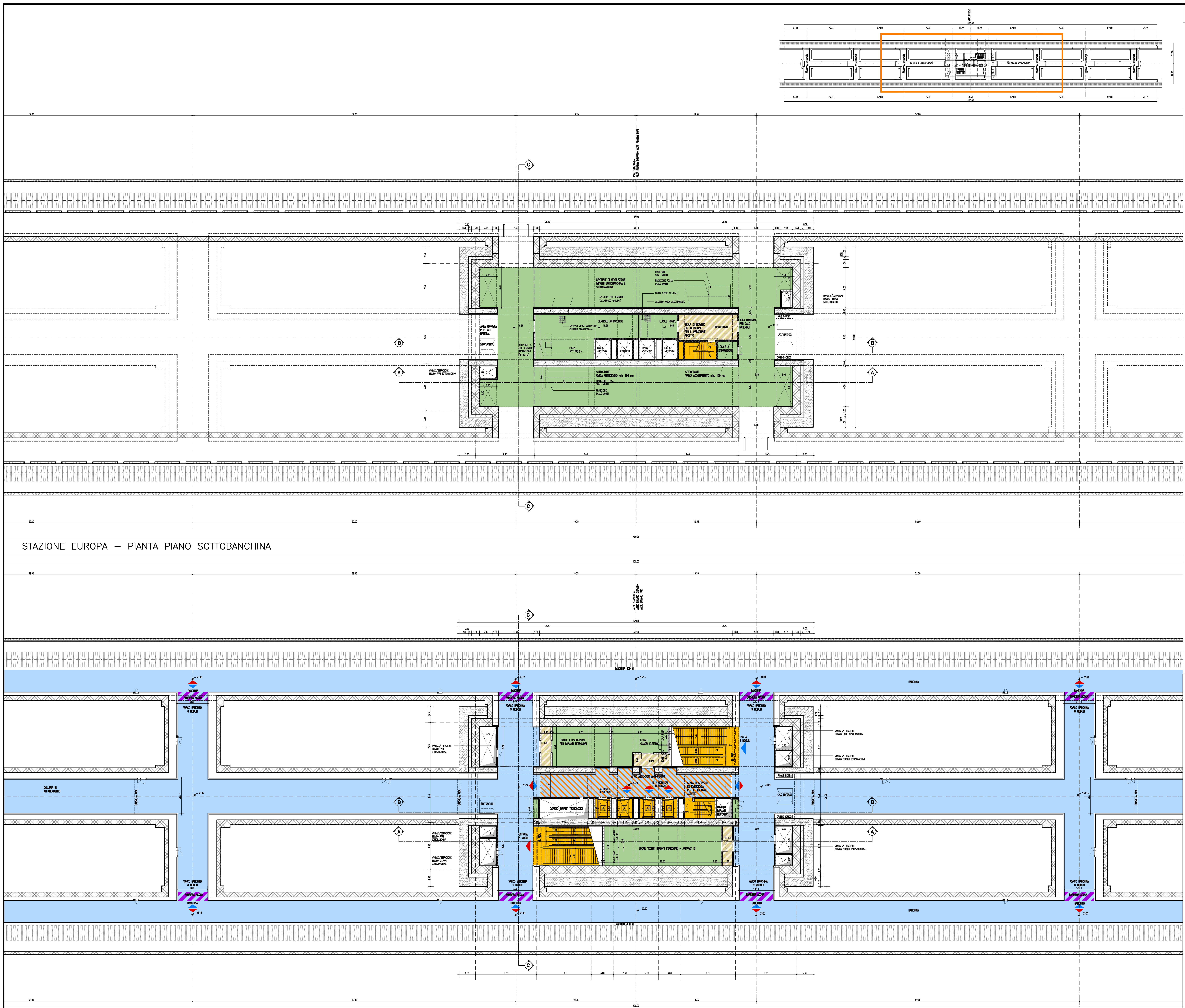
STAZIONE EUROPA – PIANTA PIANO BANCHINA
