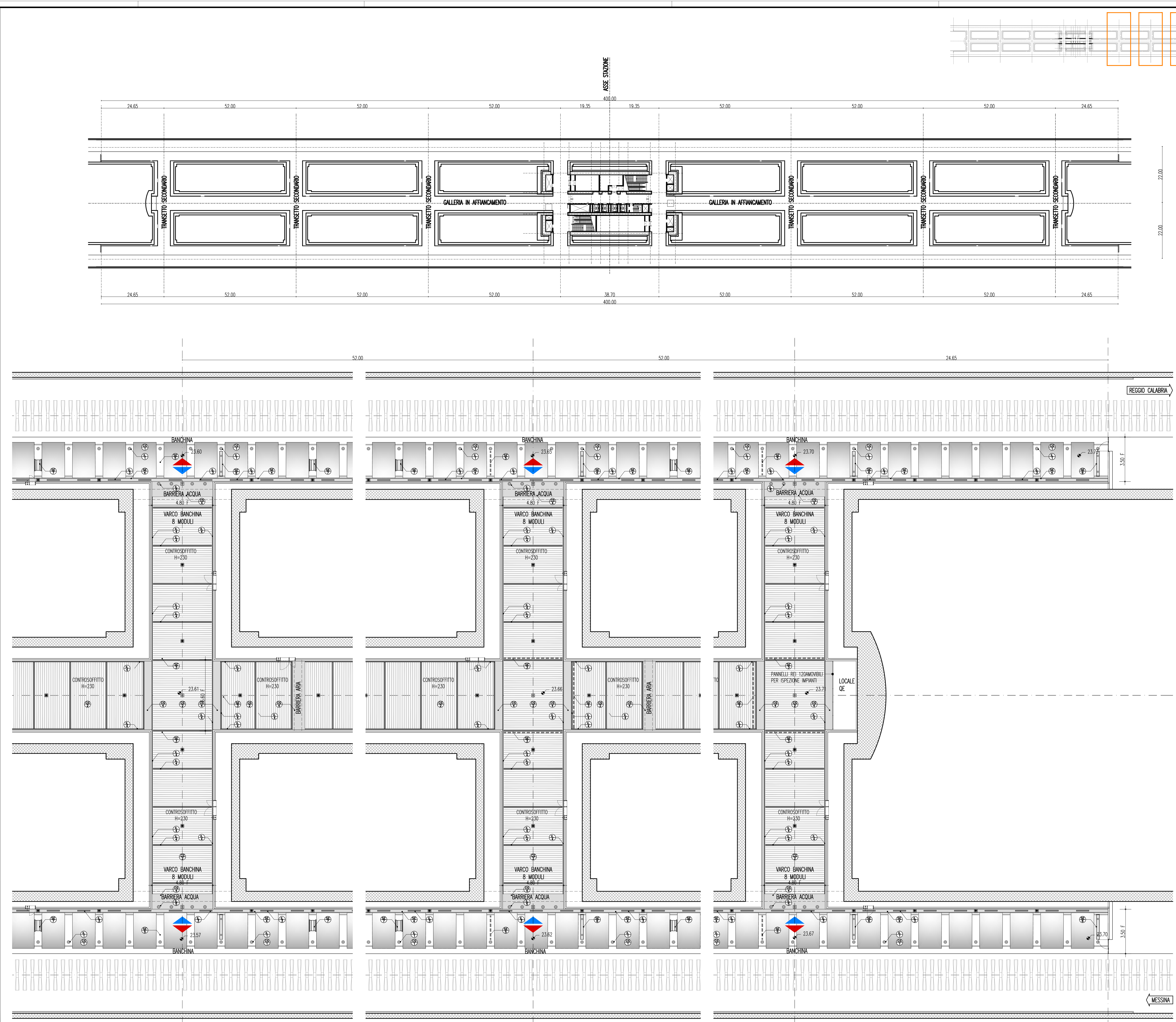
STAZIONE EUROPA - PIANTA CONTROSOFFITTI PIANO BANCHINA - LATO REGGIO CALABRIA
