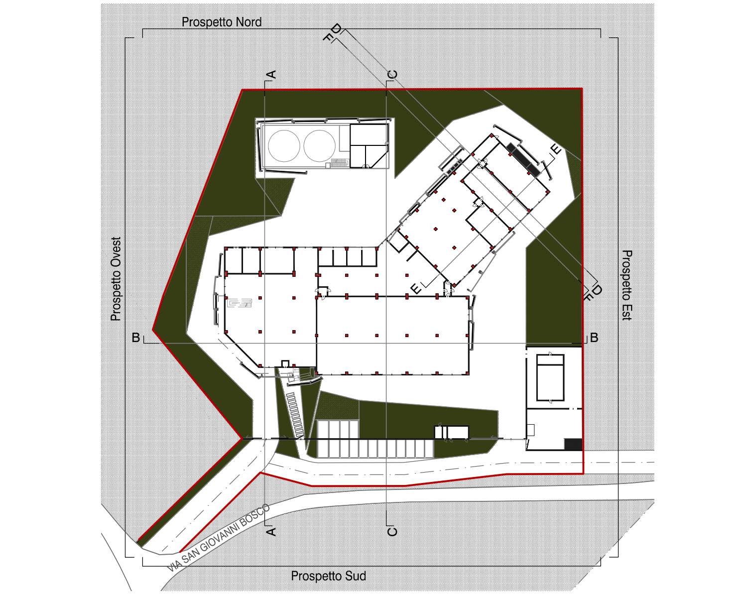
Pianta piano terra, scala 1:1000 Key plan
