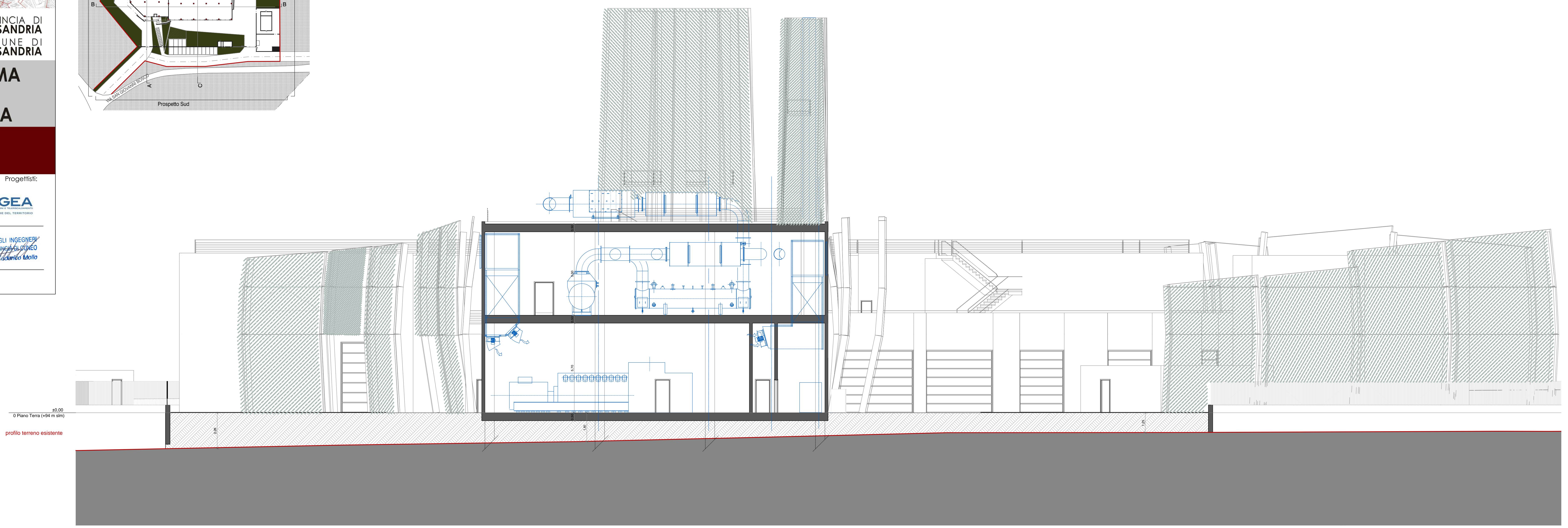
Sezione D, scala 1:100
