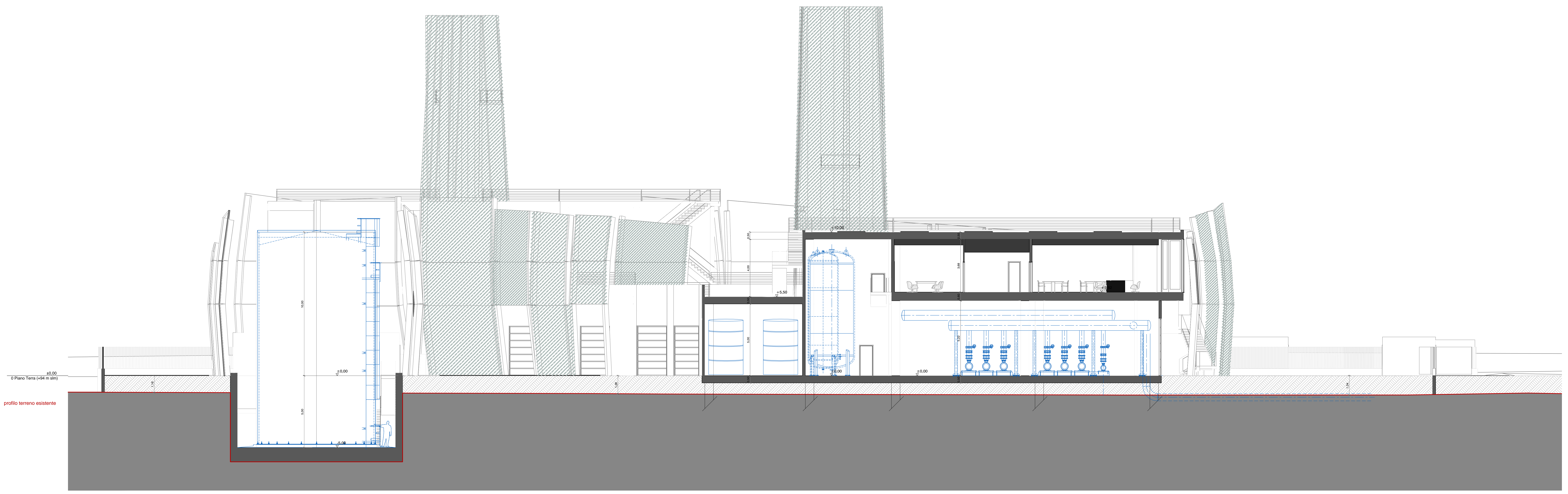
Sezione A, scala 1:100
