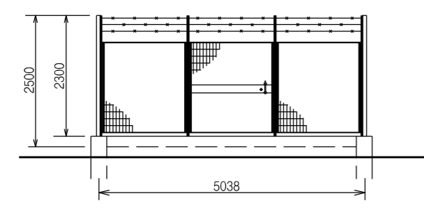
PROSPETTO A – Scala 1:100
