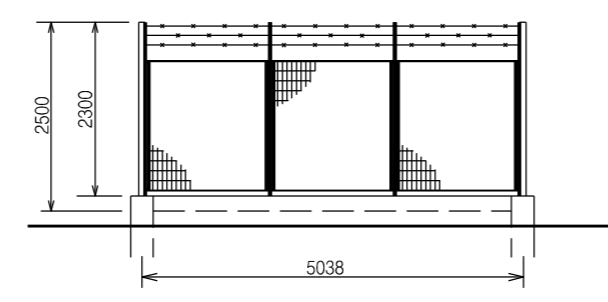
PROSPETTO B – Scala 1:100
