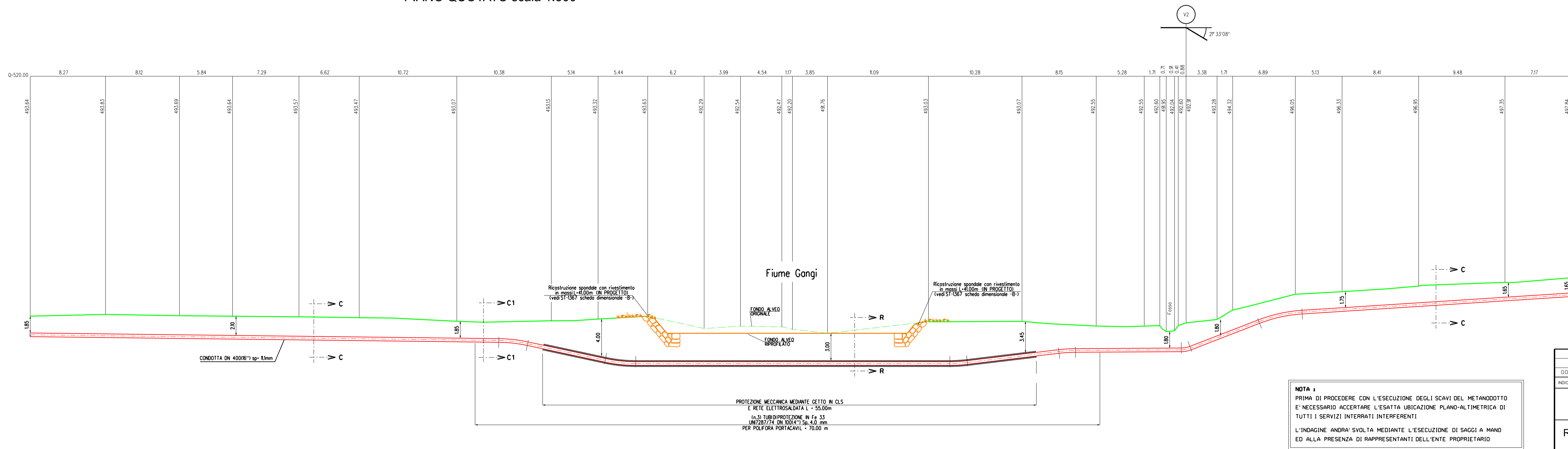
SEZIONE A - B scala 1:200
