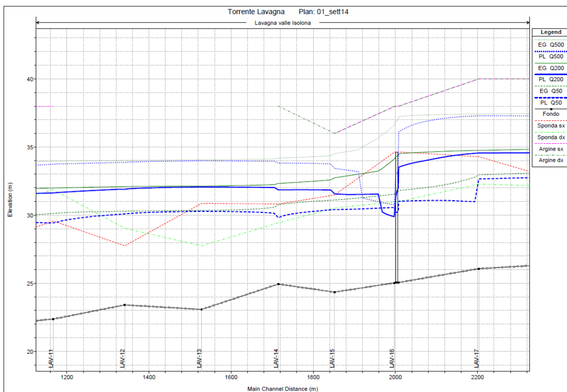
Fig. 6.3/C: Torrente Lavagna, profili di corrente per le portate di piena nel tratto interessato dall'attraversamento #1, in prossimità della sezione LAV14
