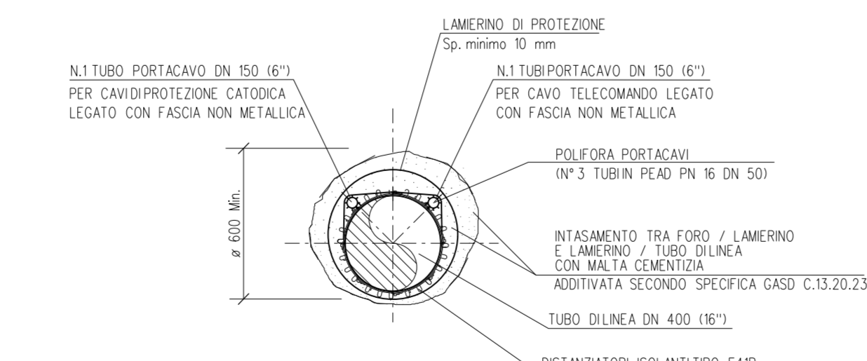
SEZIONE C-C RAISE-BORER
