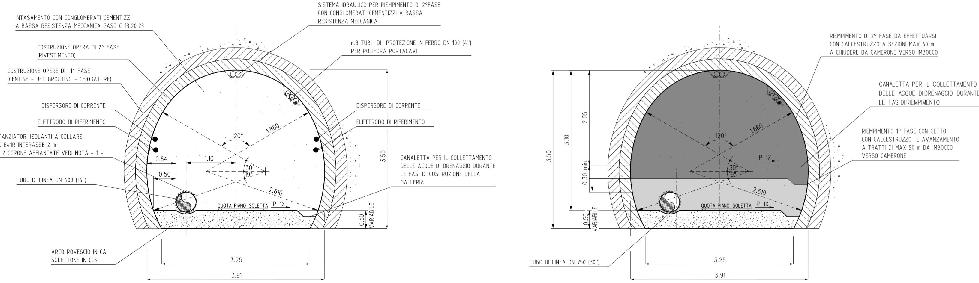
SEZIONE A-A POLICENTRICA CON FASI DI INTASAMENTO
