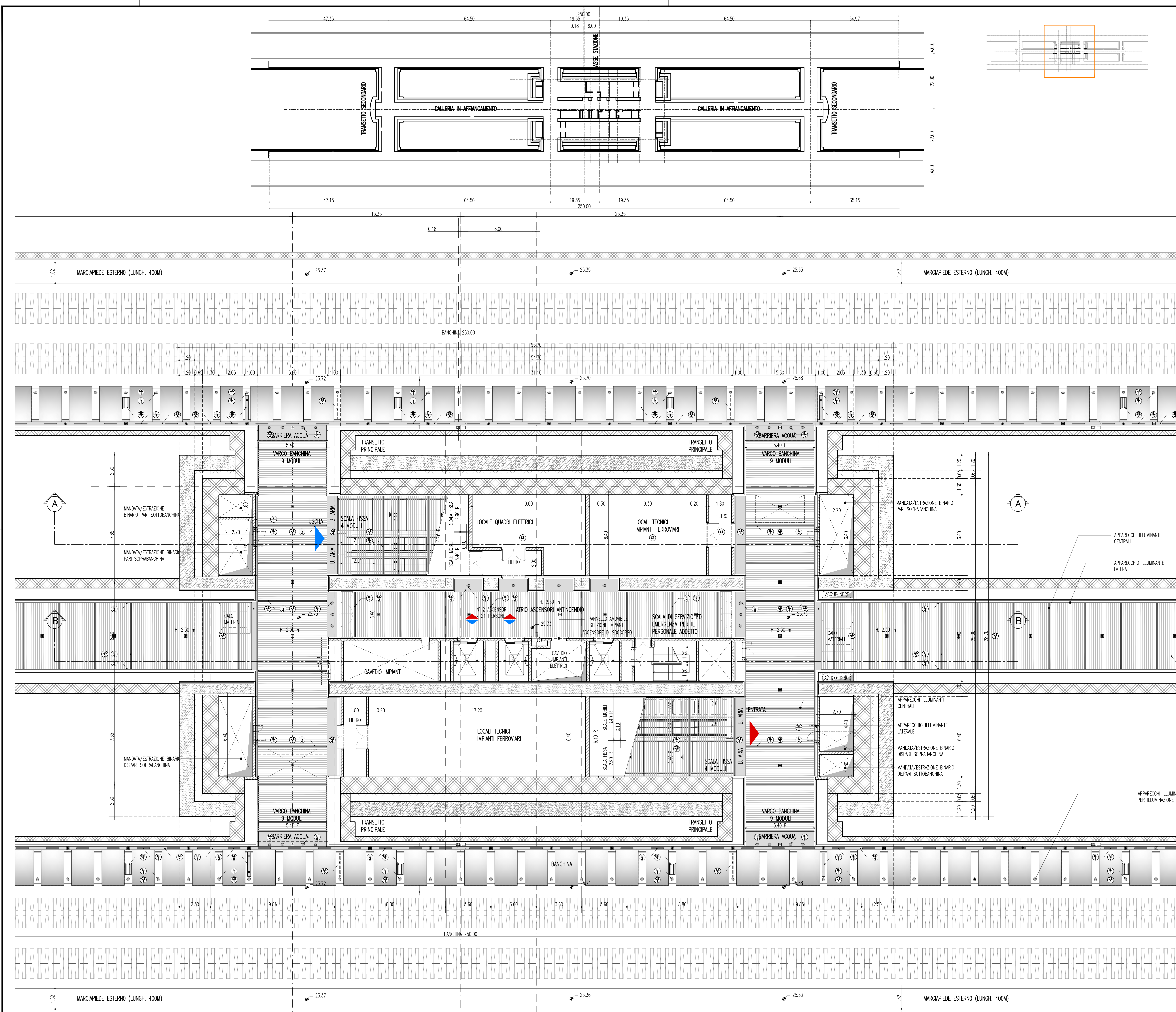
STAZIONE PAPARDO - PIANTA CONTROSOFFITTI PIANO BANCHINA
