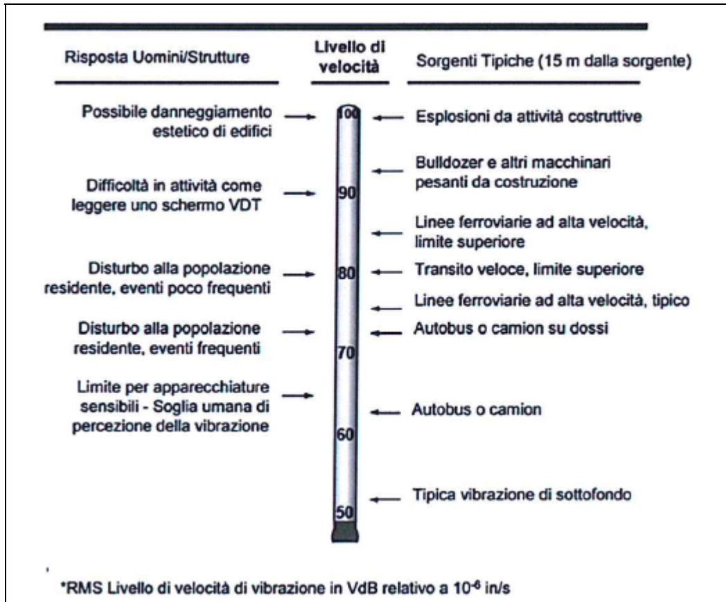
Fig. 7.8.A: Livelli tipici di vibrazione derivanti da attività umane (si evidenzia che la scala delle velocità è in dB pertanto l'ampiezza raddoppia ogni 3 dB)
