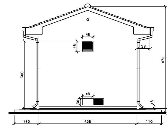
PROSPETTO B
