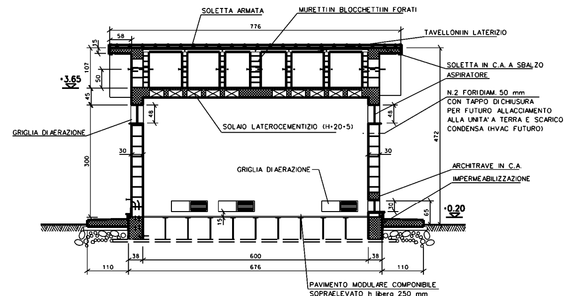
SEZIONE A-A
