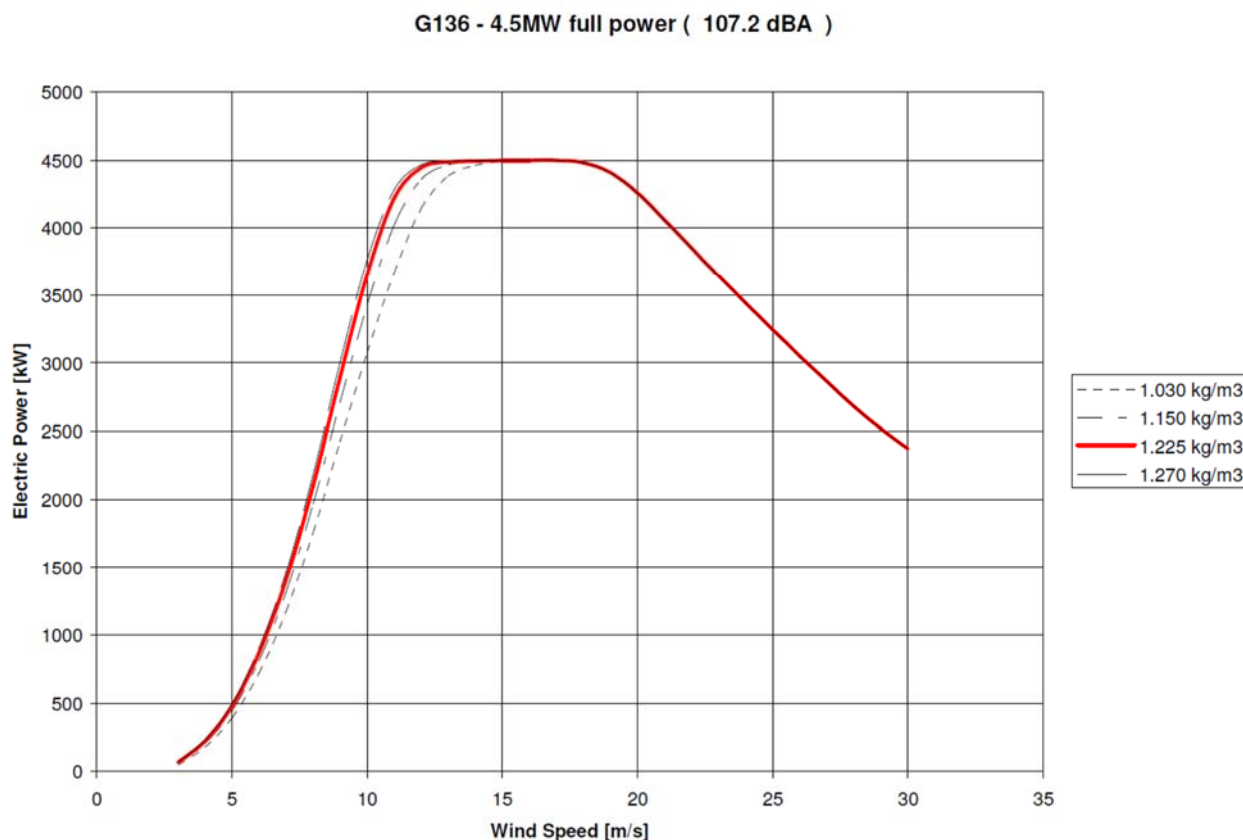
Fig.3.3: Curva di Potenza dell'aerogeneratore
