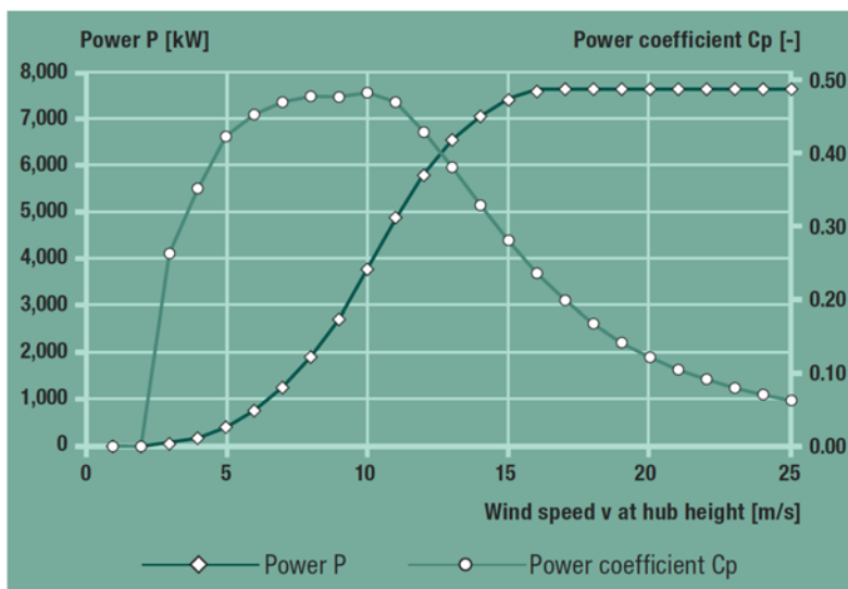
Fig.2.2: Curva di Potenza dell'aerogeneratore
