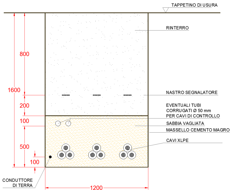
Figura 1: Posa del cavidotto AT
