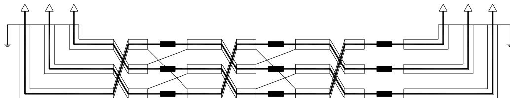
Schema di connessione delle guaine metalliche
