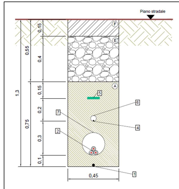
Sezione tipo su strada brecciata
