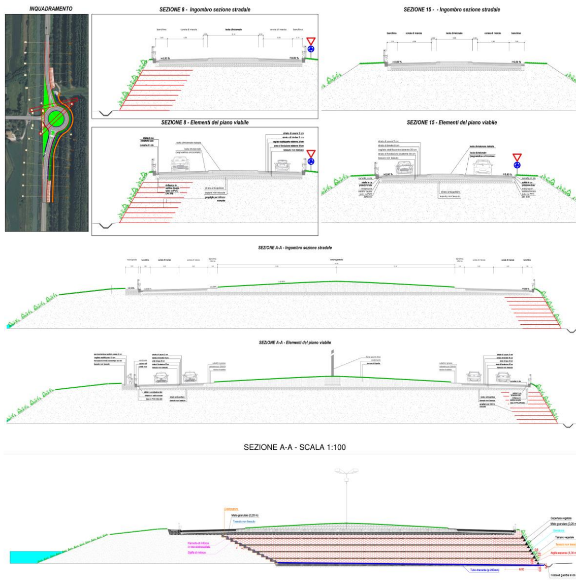
Figura 3 - Sezioni tipo della rotatoria in rilevato e della strada.
