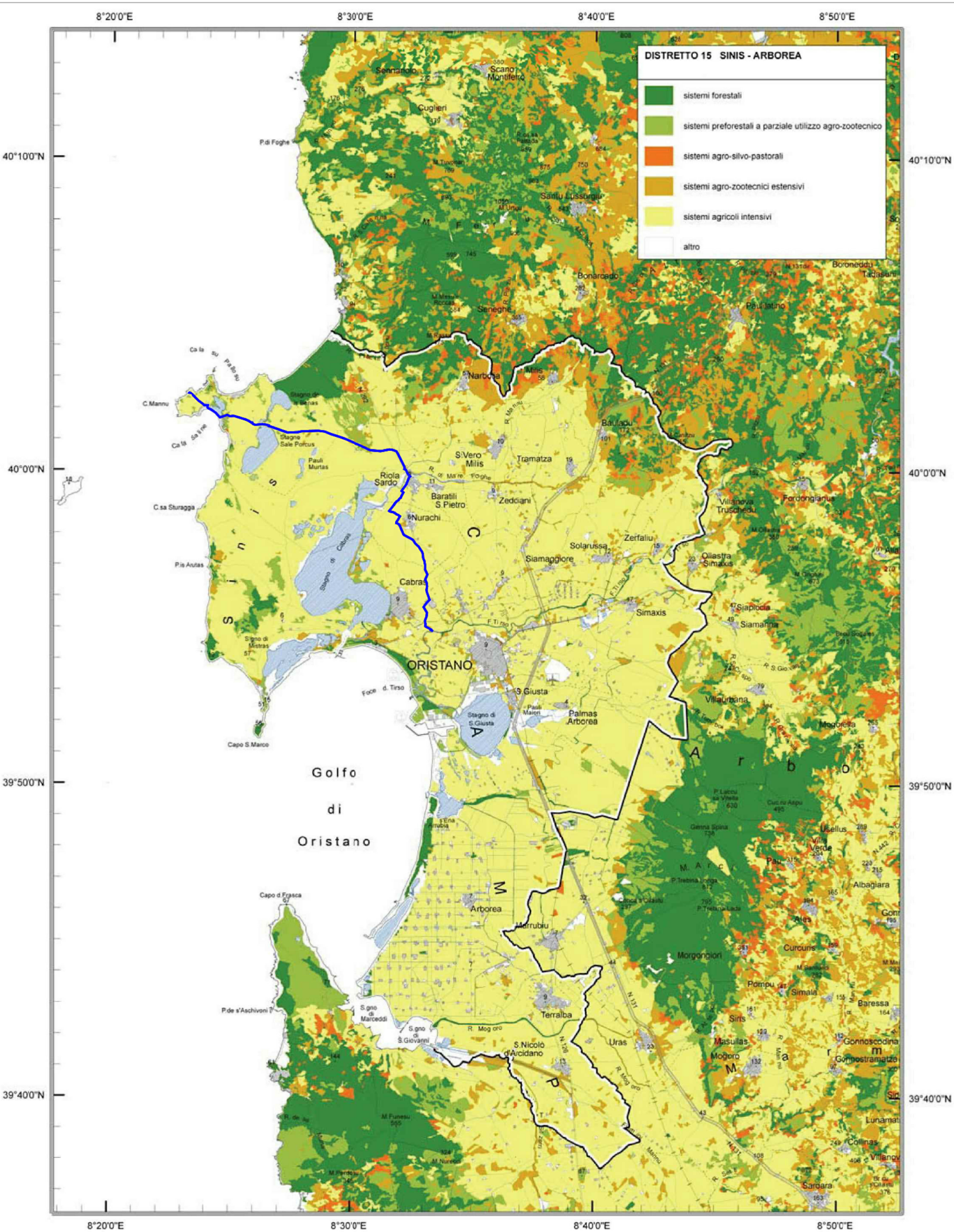
Uso del Suolo (fonte: Piano Forestale Ambientale Regionale, R.A.S., 2007)
