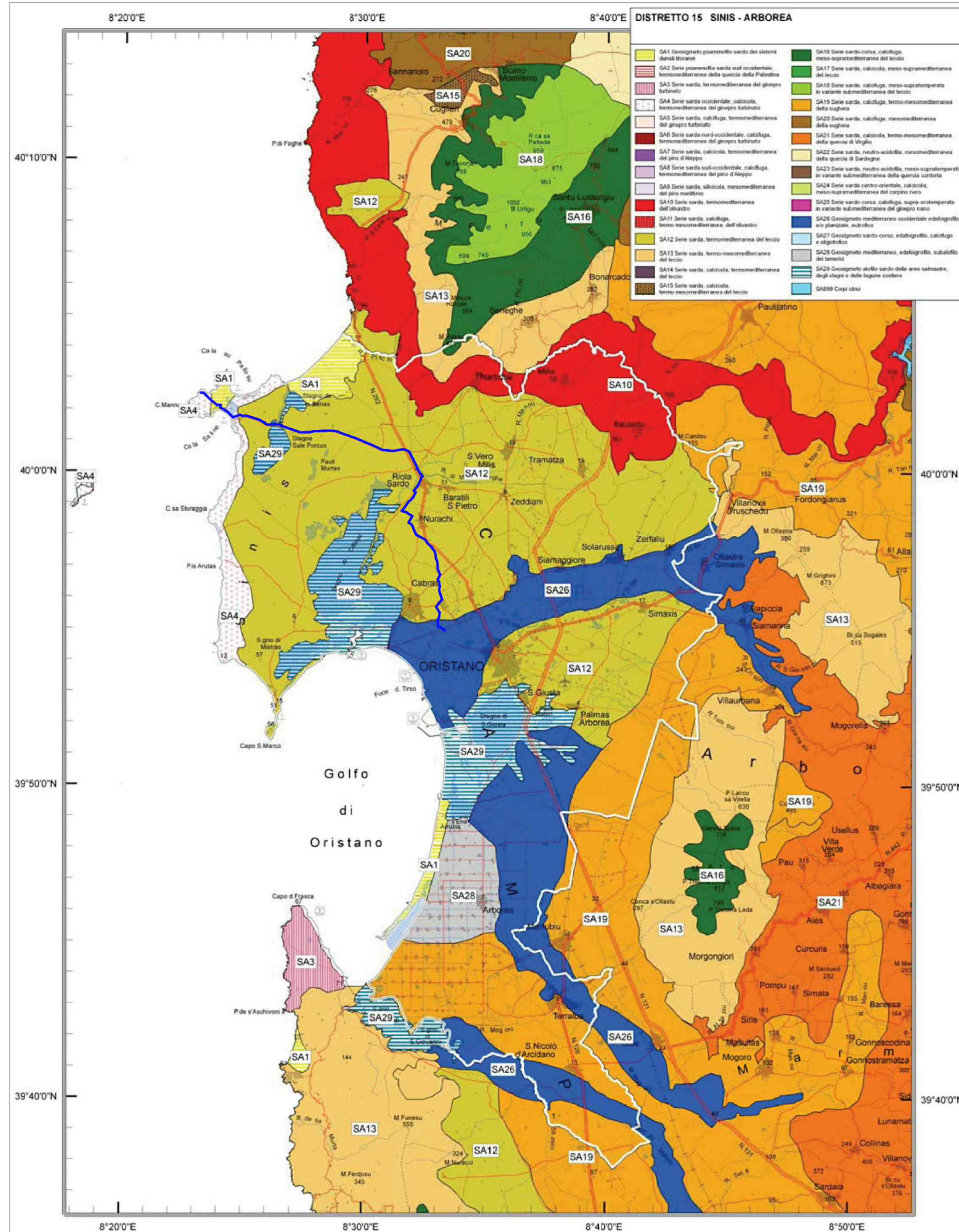
Serie di Vegetazione (fonte: Piano Forestale Ambientale Regionale, R.A.S., 2007)
