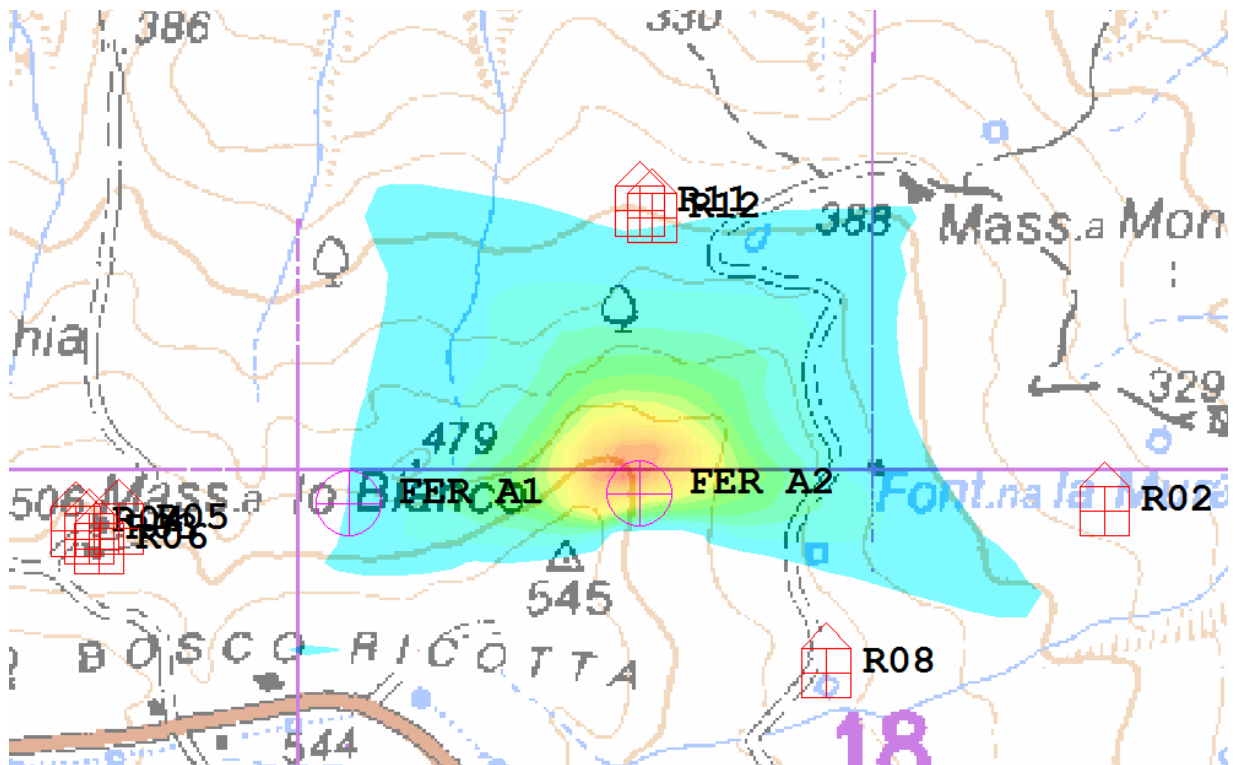
Figura 4: mappa di impatto potenziale per l'aerogeneratore 2
