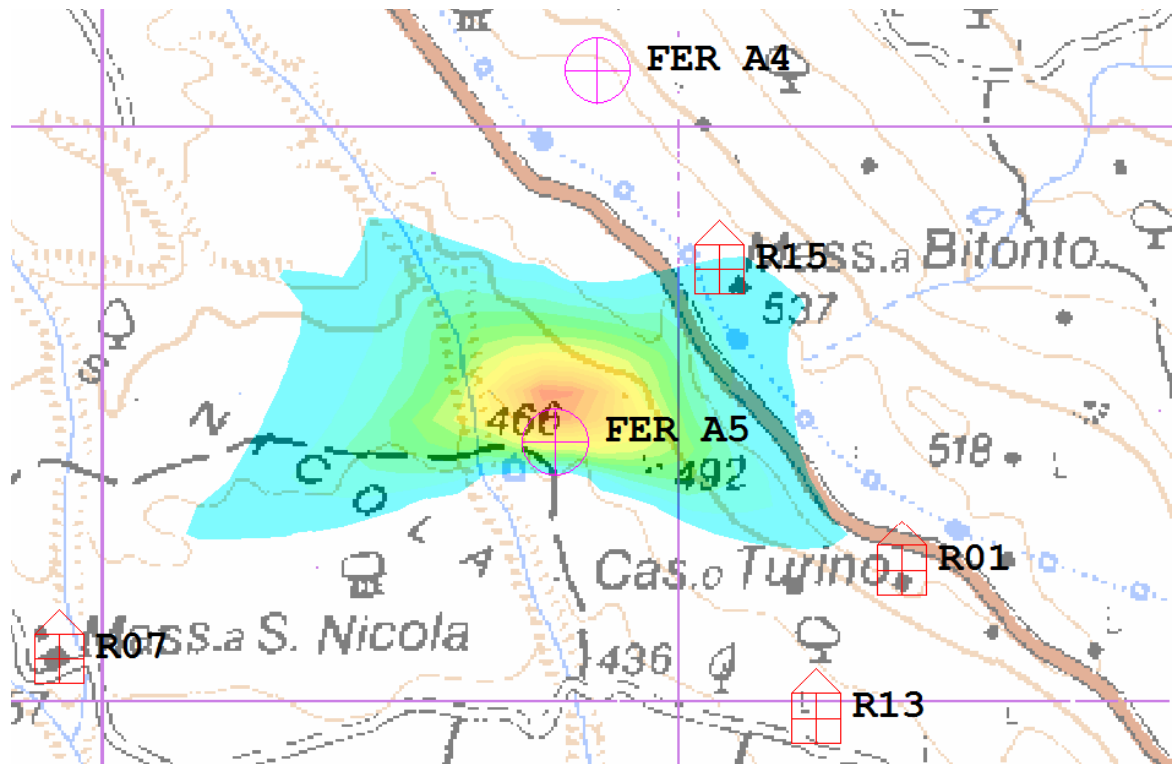
Figura 7: mappa di impatto potenziale per l'aerogeneratore 5
