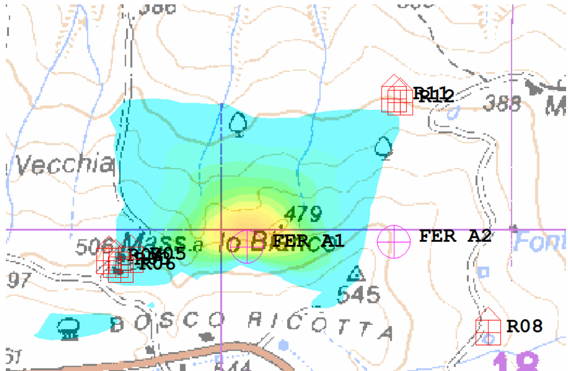
Figura 3: mappa di impatto potenziale per l'aerogeneratore 1
