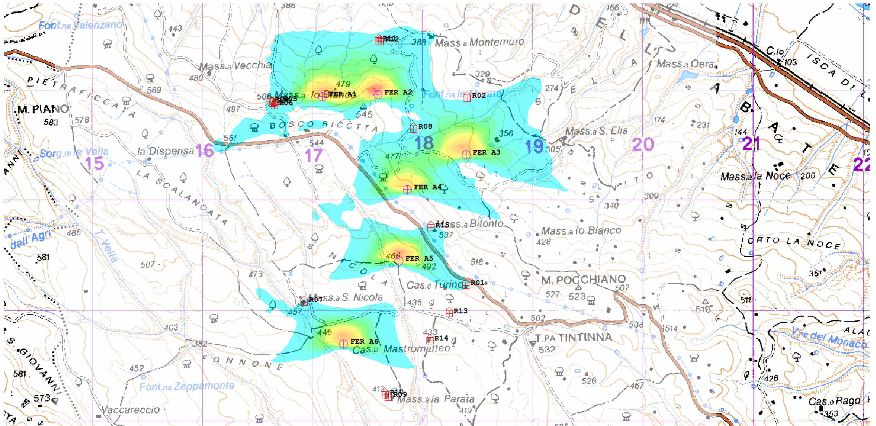
Figura 9: mappa di shadow flickering su base IGM
