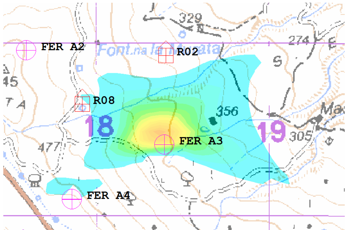
Figura 5: mappa di impatto potenziale per l'aerogeneratore 3
