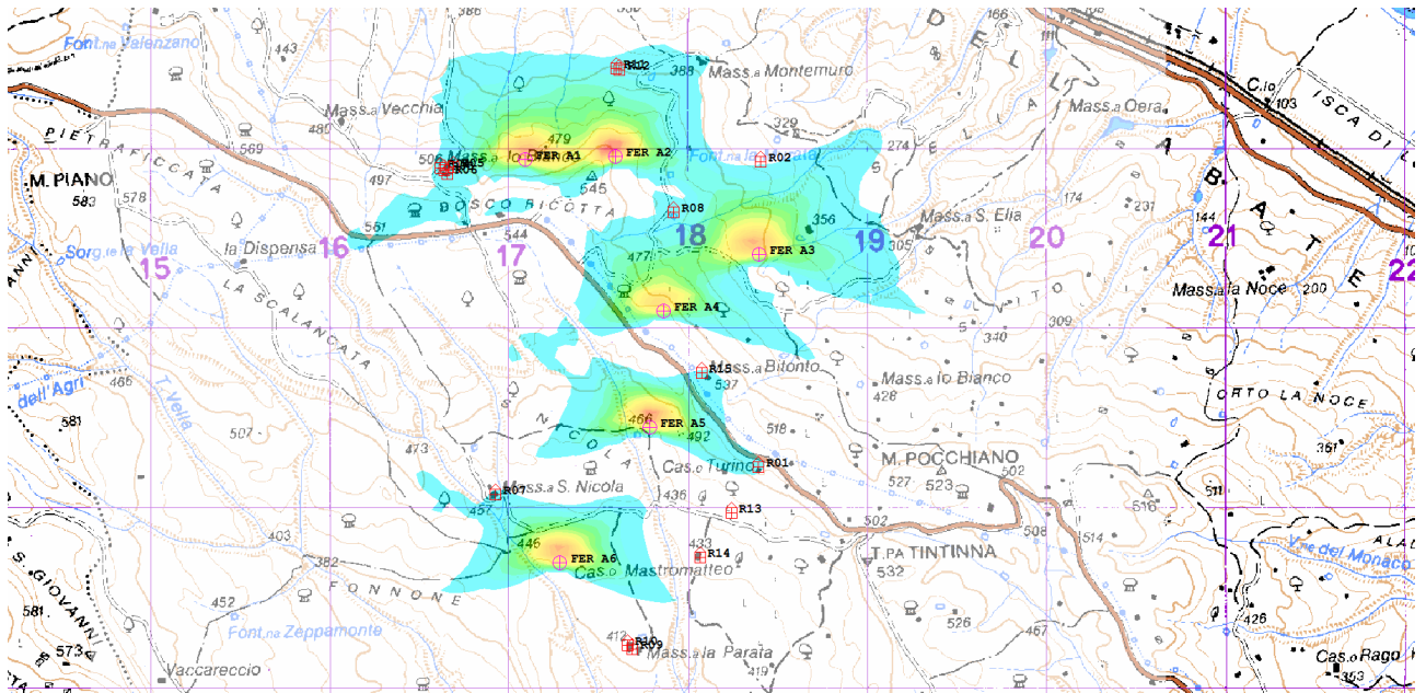
Figura 2: mappa di impatto potenziale (stralcio) da shadow flickering per il campo eolico in esame
