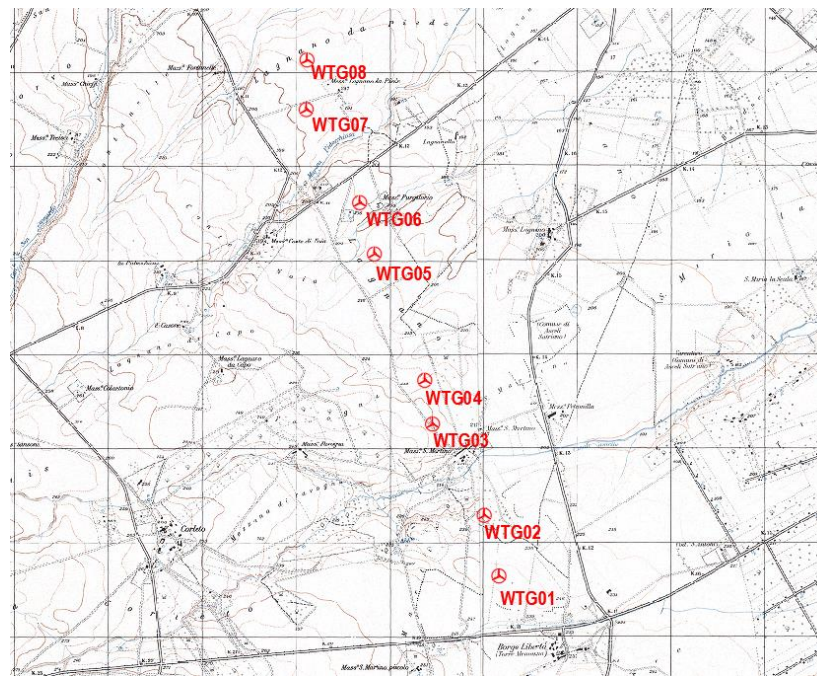
Figura 3 – Layout Alternativa 1 Schema layout a 8 WTG su unica fila
