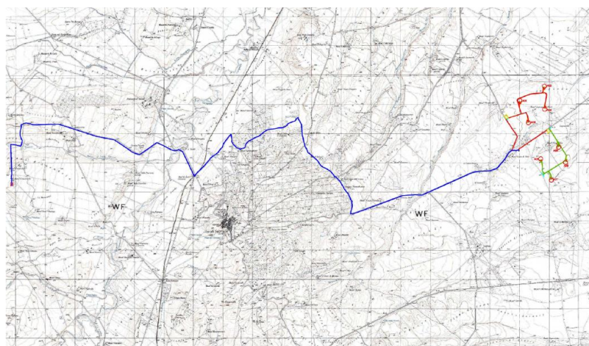
Figura 4 – layout d'impianto
