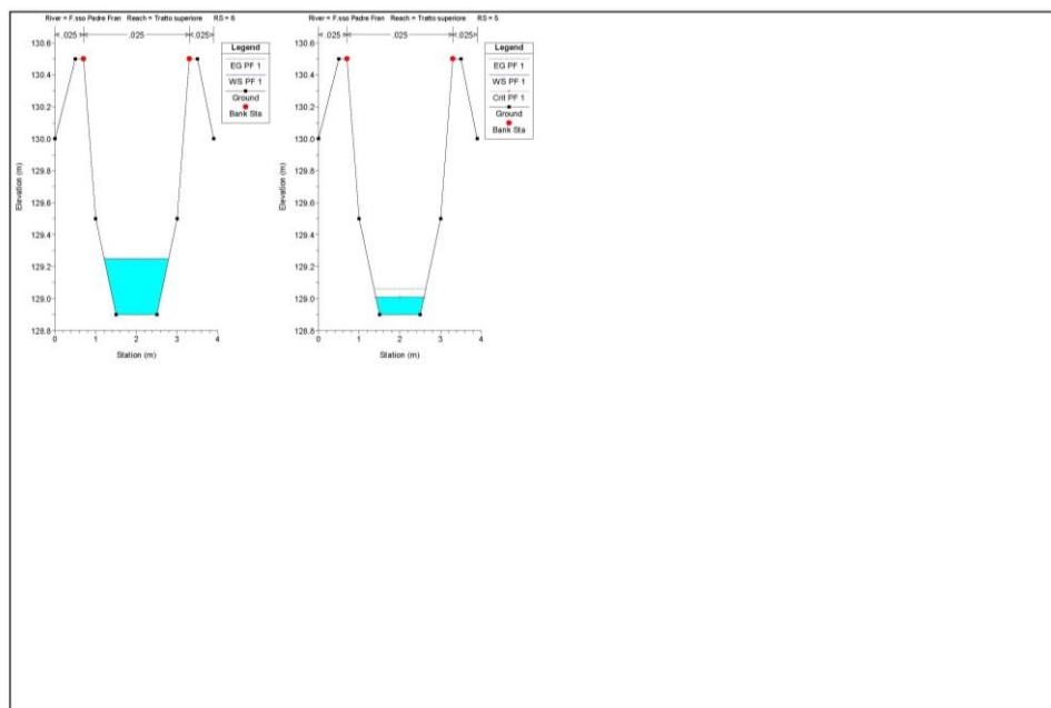
Figura 14: Bacino 2 – F.sso Padre Francesco- Tratto superiore - individuazione sezioni significative.
