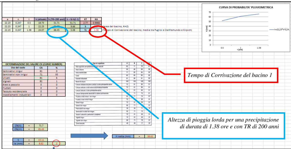
Figura 4: sviluppo dell'equazione proposta dal Va. Pi. per la Zona 2, rappresentazione della CPP e definizione della pioggia netta con il metodo del Curve Number per il bacino 1.
