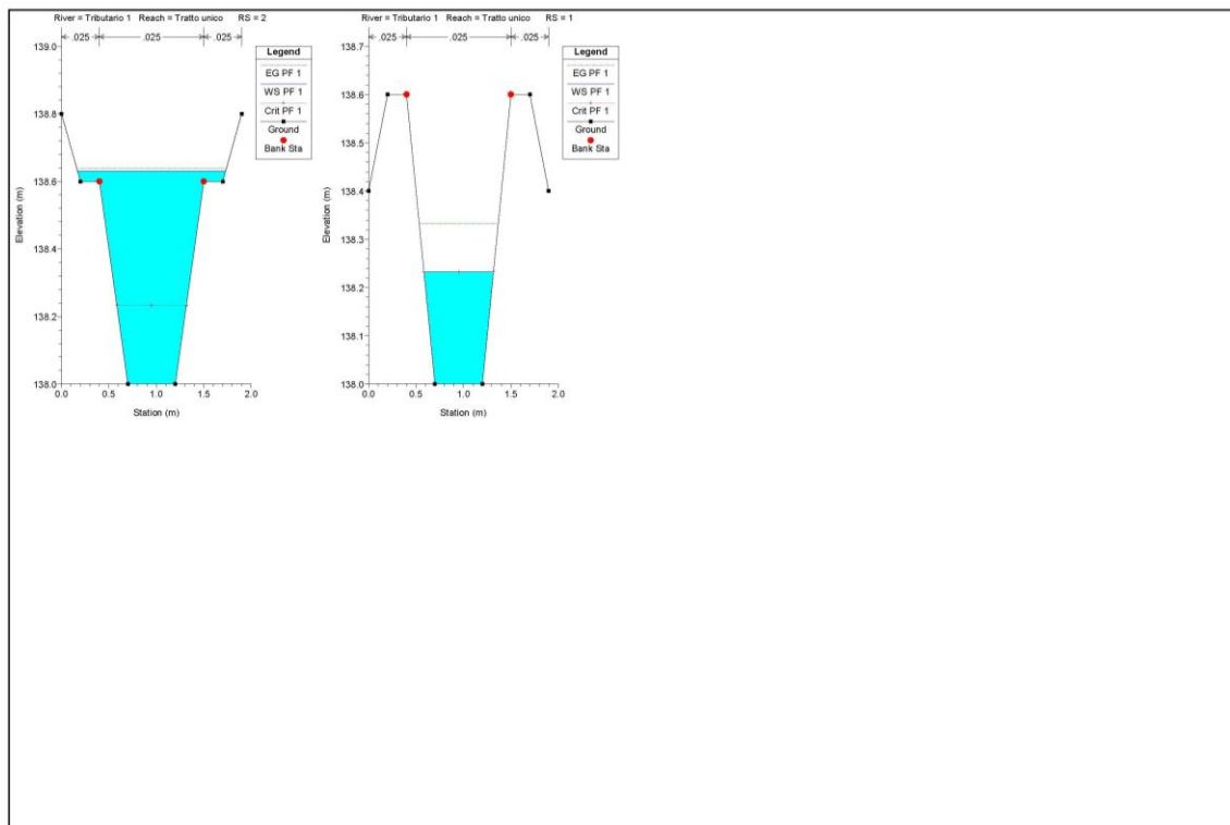
Figura 18: Bacino 4 - Tributario 1 - Tratto unico - individuazione sezioni significative.
