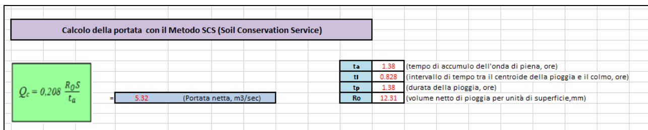
Figura 5: calcolo della portata "Q" con il metodo del Curve Number.
