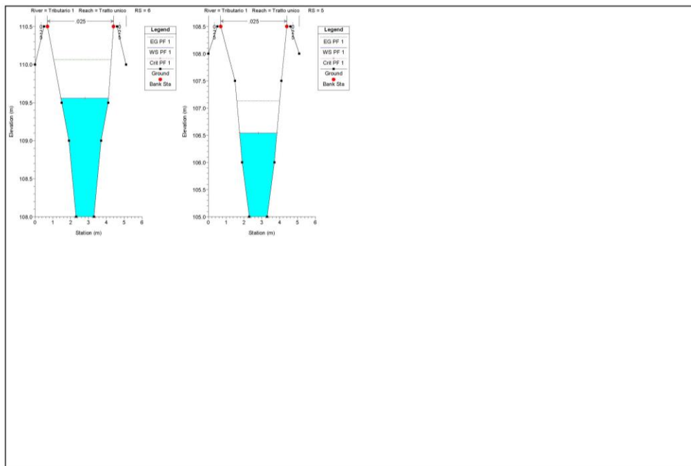
Figura 24: Bacino 9 - Tributario 1 - individuazione sezioni significative.
