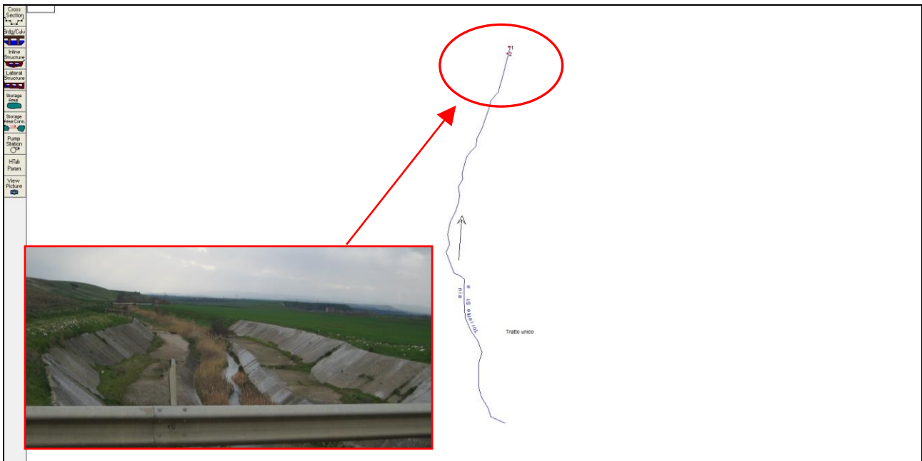
Figura 34: Bacino 19 – Torrente Staina - individuazione sezioni significative e reportage fotografico.
