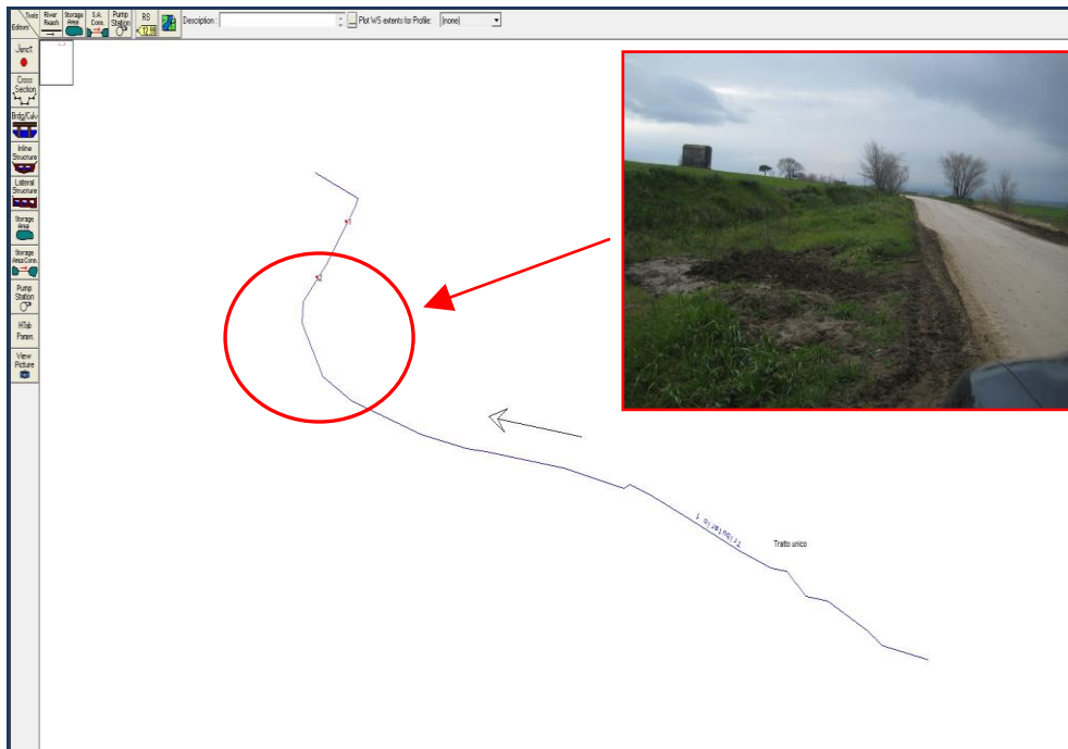
Figura 28: Bacino 13 - Tributario 1 - individuazione sezioni significative e reportage fotografico.
