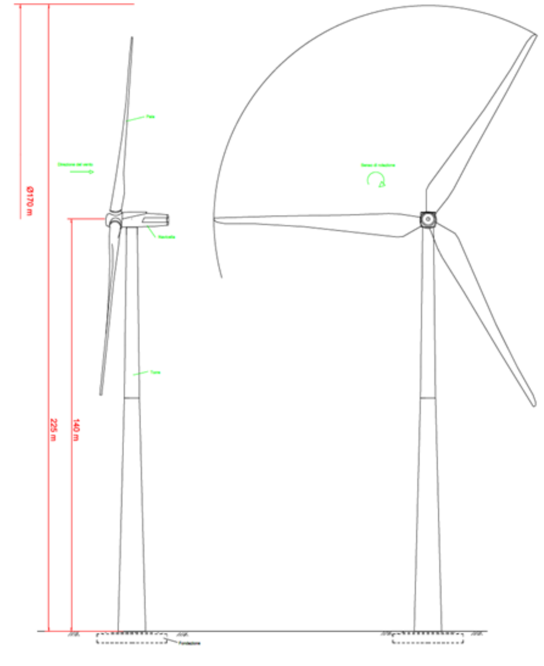
-Aerogeneratore Tipo-
