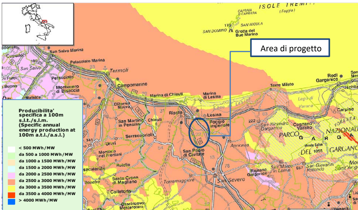
Figura 4: Area d'intervento su atlante eolico interattivo con producibilità specifica a 100m - C.E.S.I.
