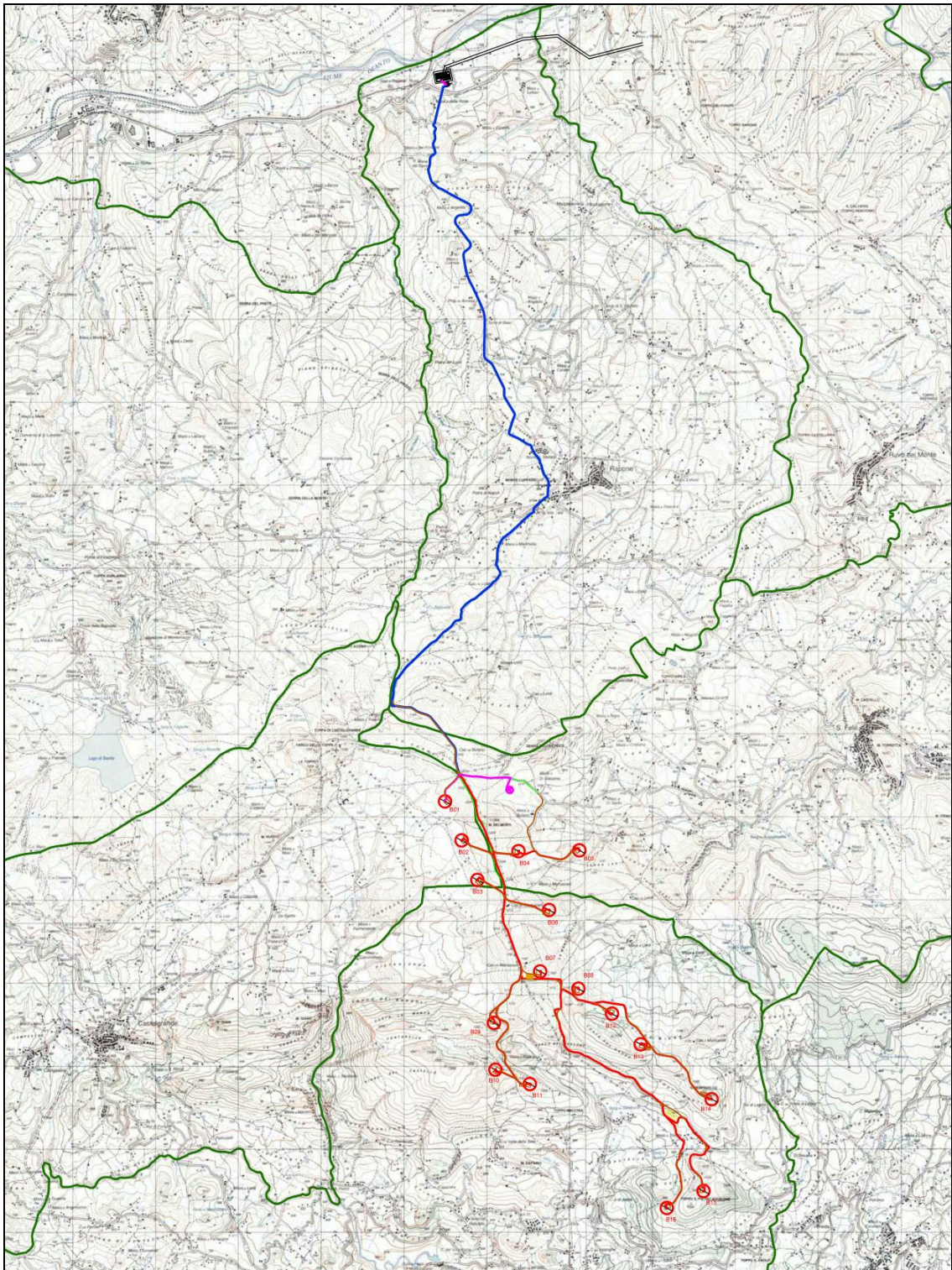
Fig. 1 – Planimetria generale dell'impianto eolico su IGM 25000
