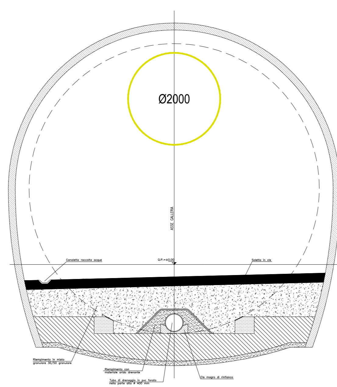
TRATTA IN TRADIZIONALE SEZIONE TRASVERSALE da pk 0+117.60 a pk 0+198.00
