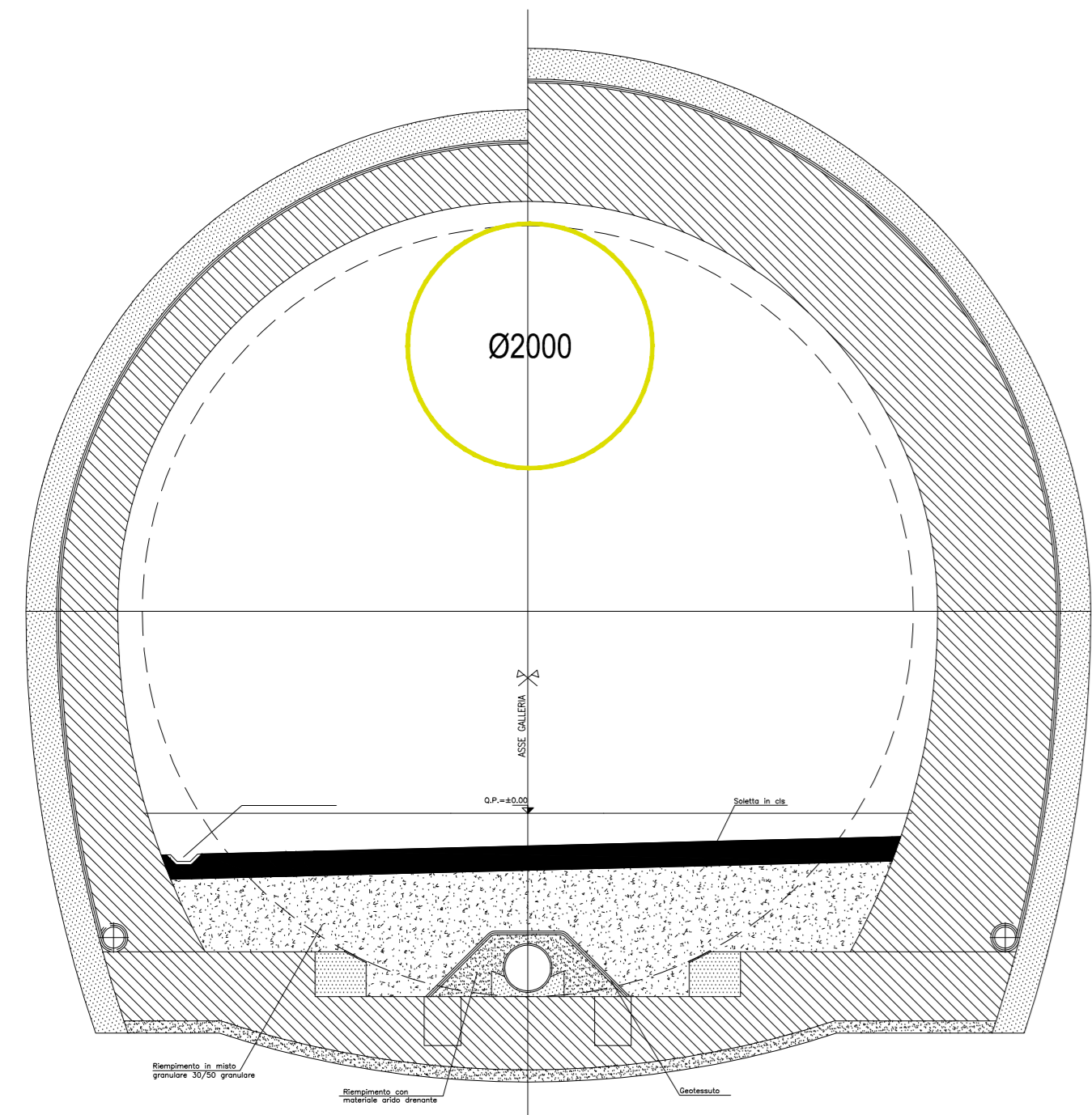
TRATTA IN TRADIZIONALE SEZIONE TRASVERSALE da pk 0+000 a pk 0+117.60
