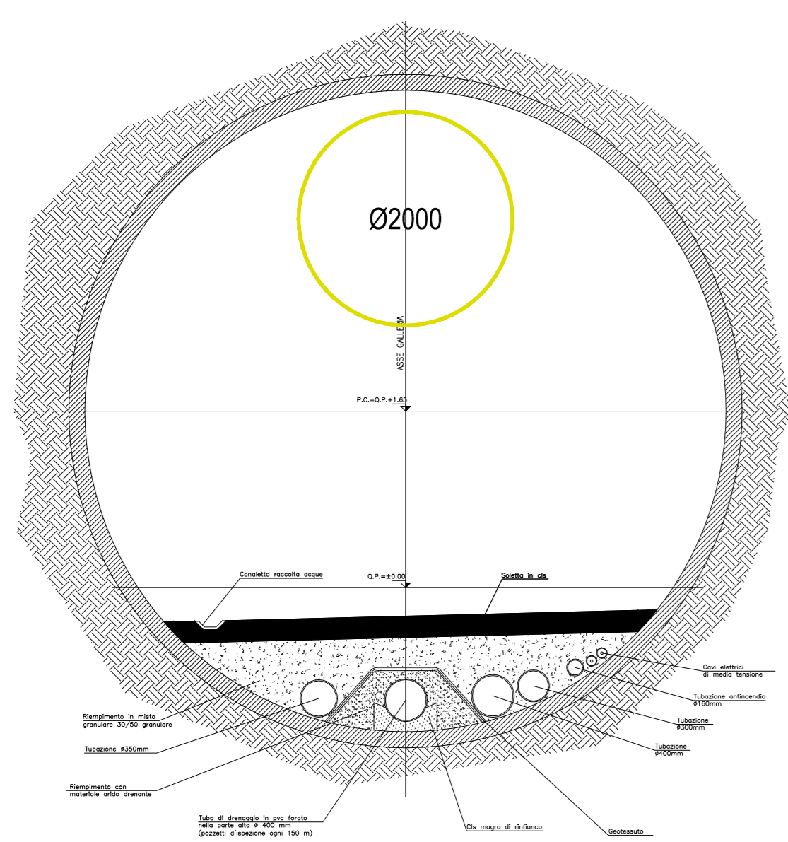
TRATTA IN MECCANIZZATO SEZIONE TRASVERSALE da pk 0+198.00 a pk 4+130.00 ca. IN PRESENZA DI CENTINA
