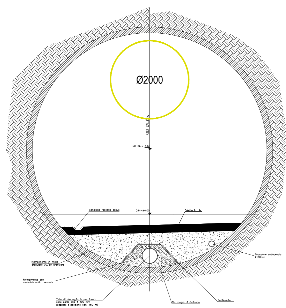
TRATTA IN MECCANIZZATO SEZIONE TRASVERSALE da pk 4+130.00 ca. a pk 7+020.00 IN PRESENZA DI CENTINA
