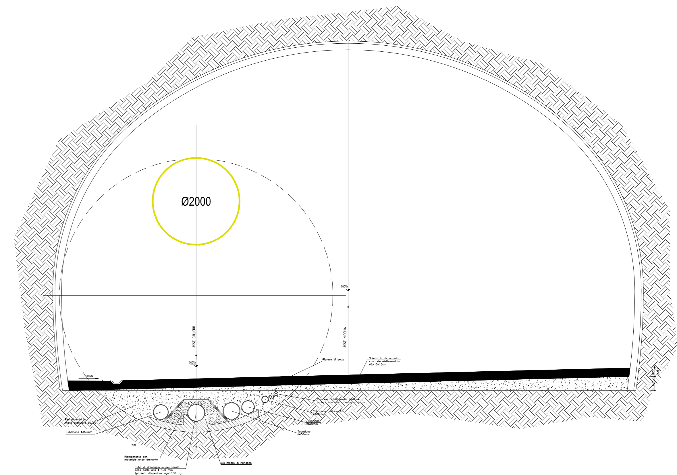
TRATTA IN MECCANIZZATO SEZIONE TRASVERSALE NICCHIA CORRENTE
