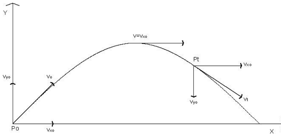
Figura 19 Traiettoria di un grave in caduta
