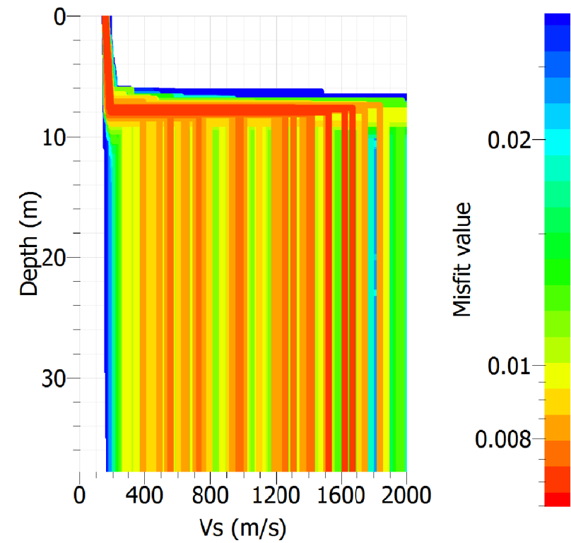
Risultati inversione Rayleigh wave (profilo modelli Vs)
