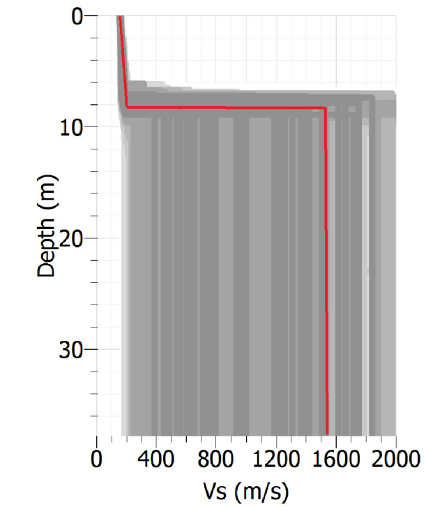
Profilo Vs Fortezza (BZ)
