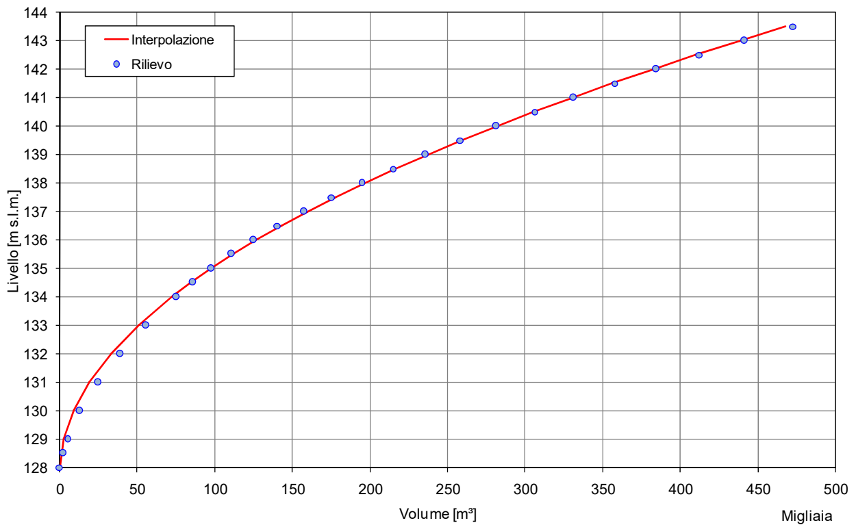
Figura 4-2 – Curva di invaso di progetto.
