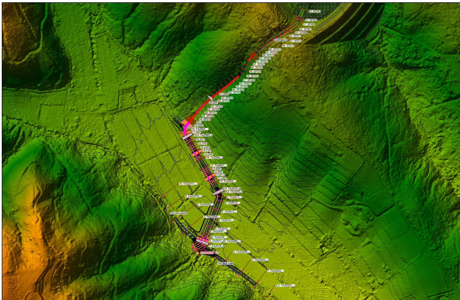
Figura 2-1 – Modello idraulico.
