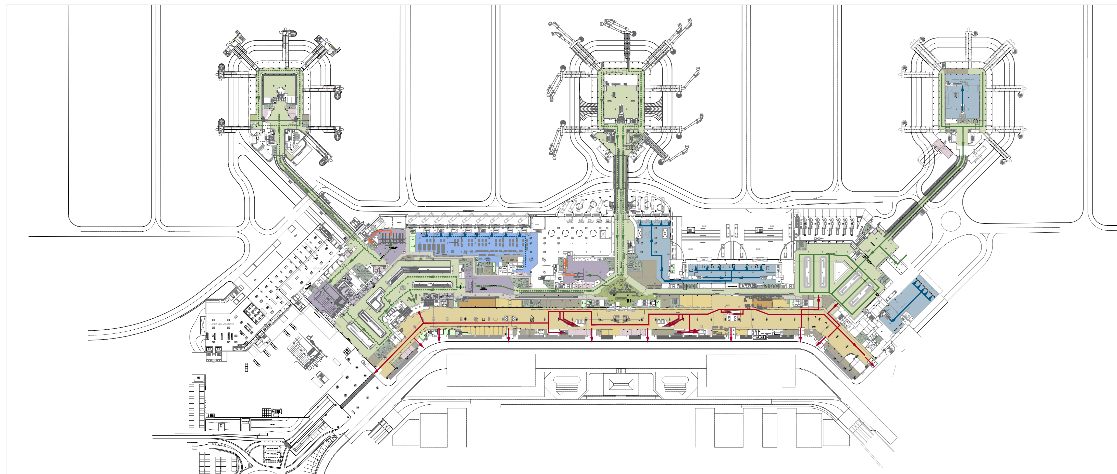
01 Terminal 1 - Pianta piano terra +1.50 Stato di fatto
