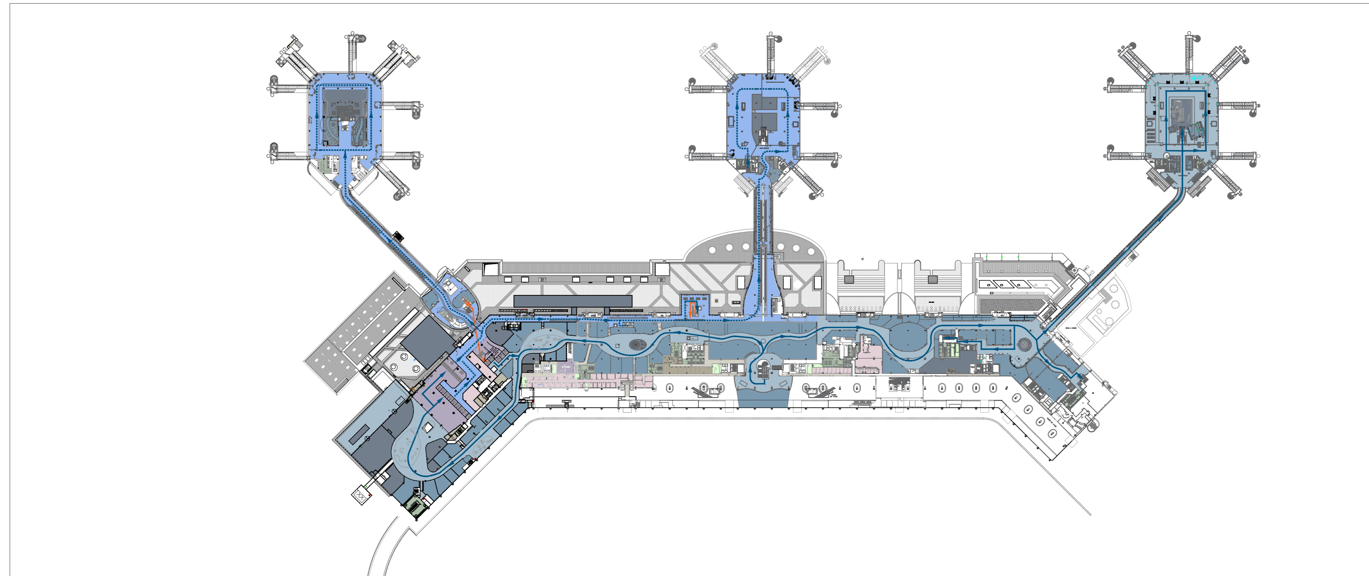
05 Terminal 1 - Pianta piano primo +7.90 Fase 1
