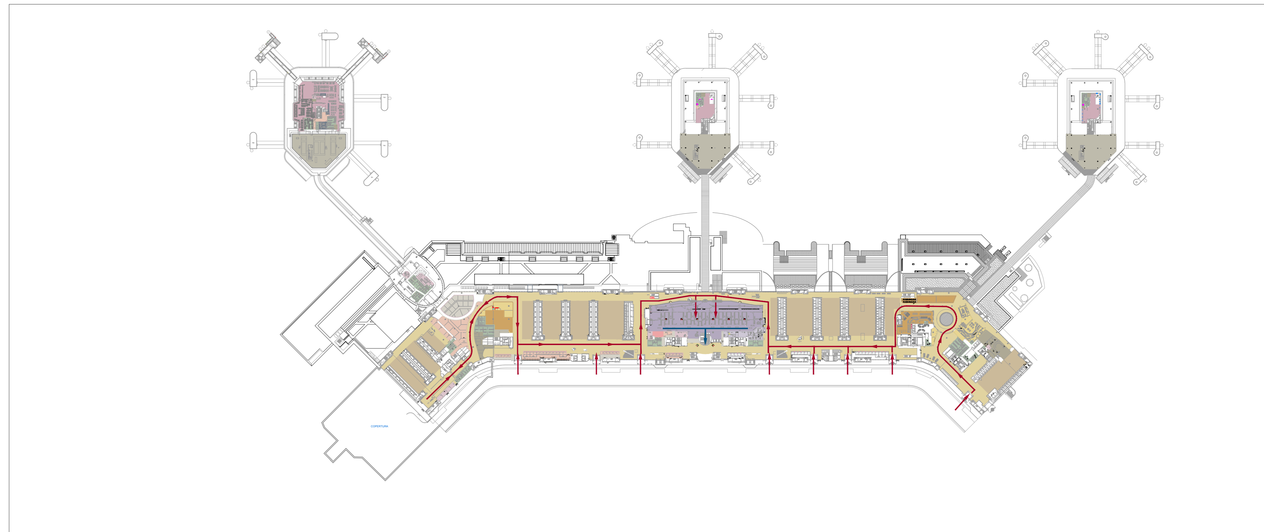
06 Terminal 1 - Pianta piano secondo +14.30 Fase 1
