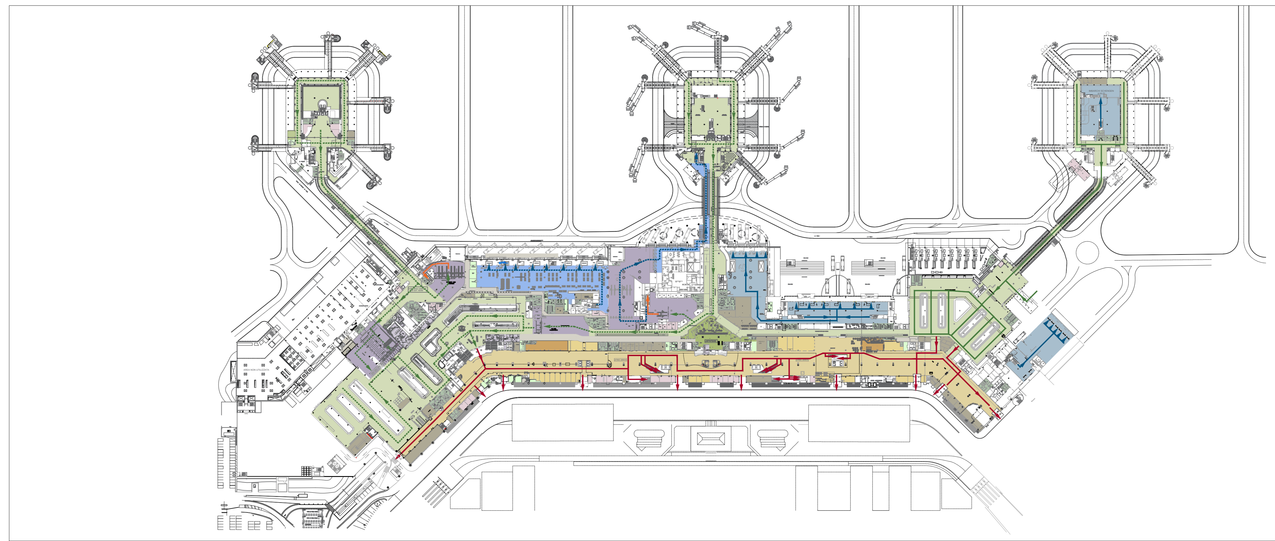
04 Terminal 1 - Pianta piano terra +1.50 Fase 1
