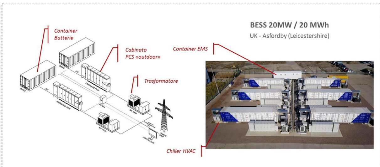
Figura 5 – Tipico "2": PCS esterno
