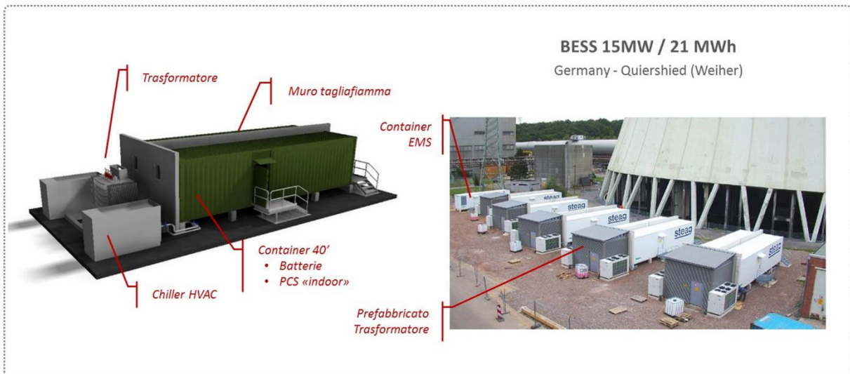
Figura 4 – Tipico "1": PCS interno al container ESS
