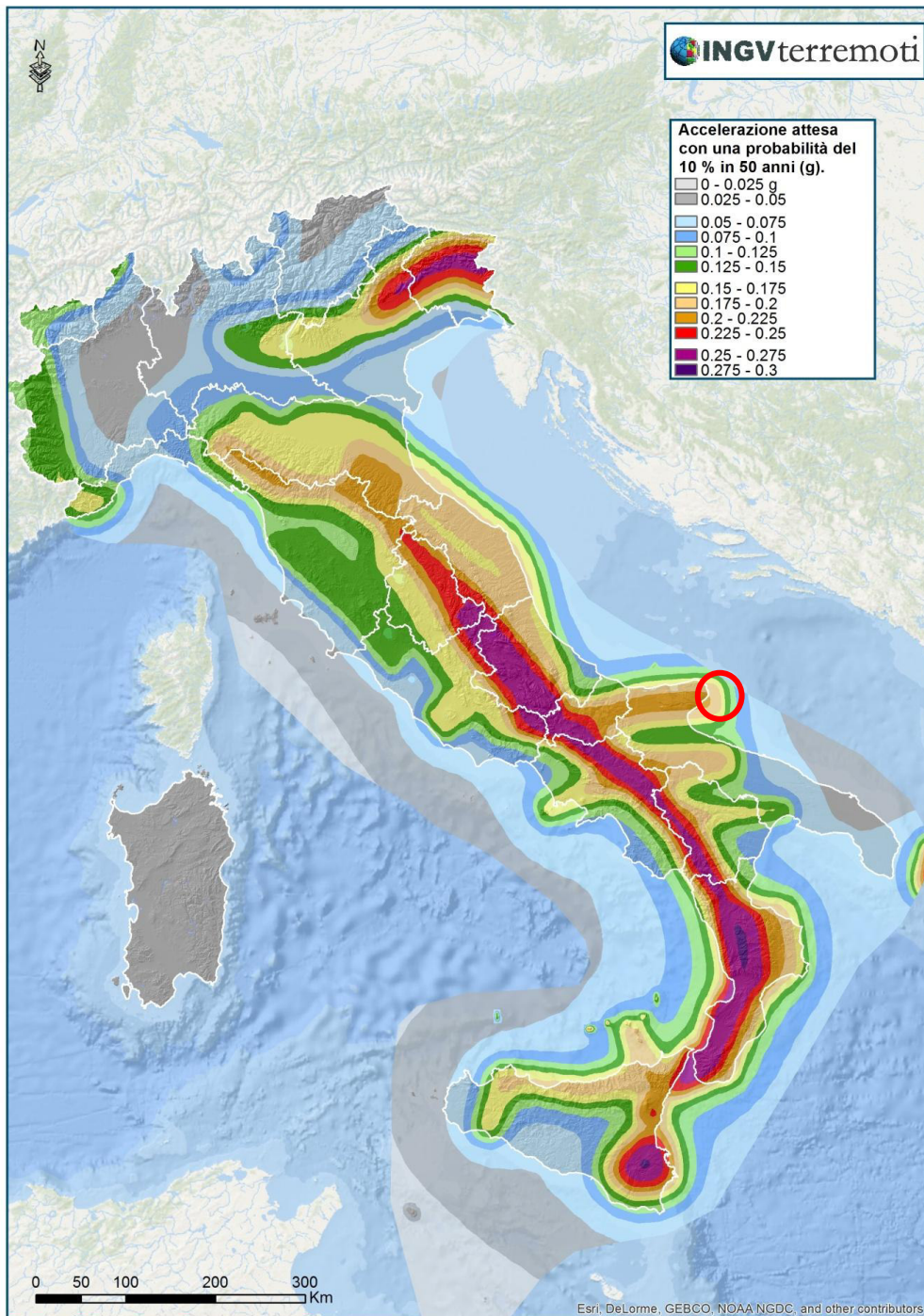
Figura 60: Accelerazione sismica
