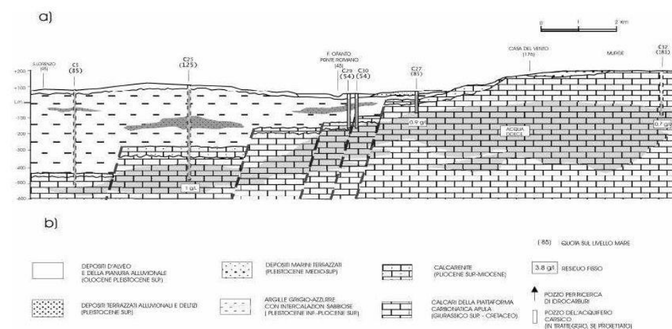
Figura 61: Sezione idrogeologica schematica (da Maggiore et Al., 2004)
