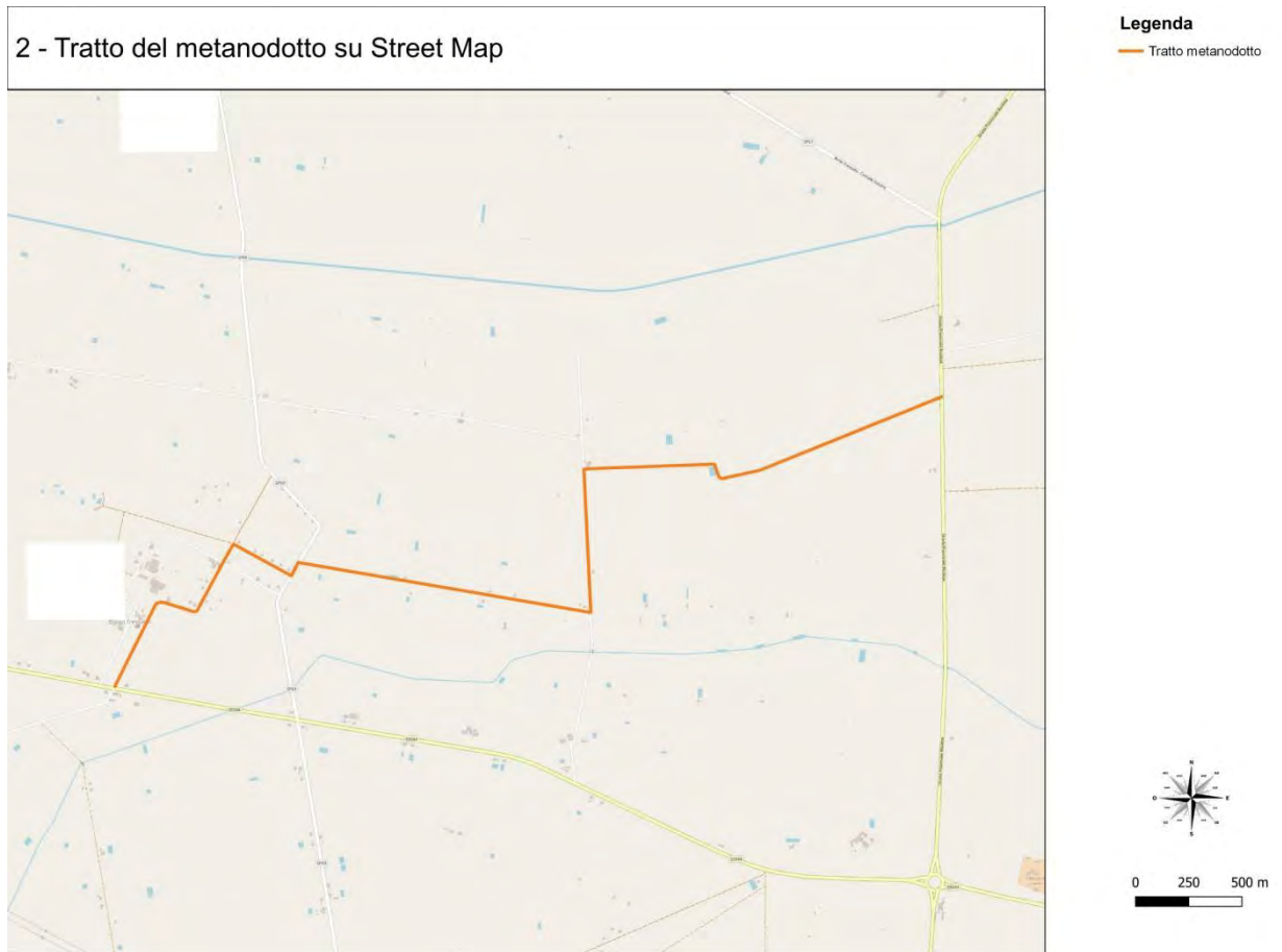
Figure 2- Tratto del metanodotto su Street Map
