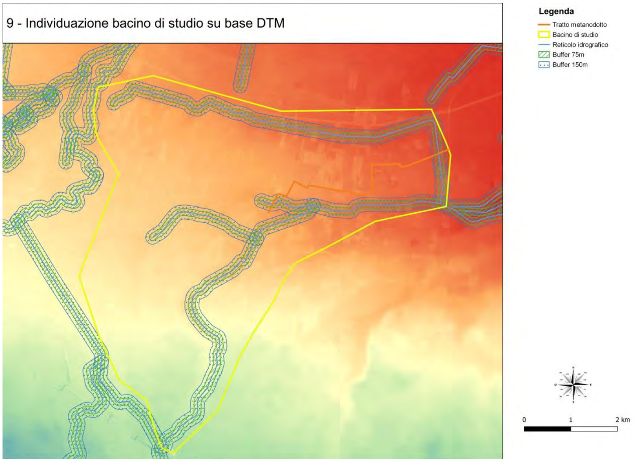
Figure 9 - Individuazione bacino di studio su base DTM
