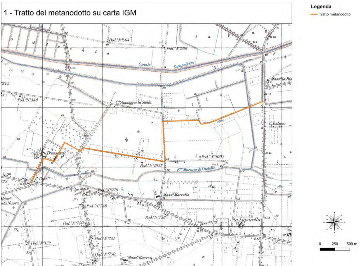
Figure 1- Tratto del metanodotto su Carta I.G.M.
