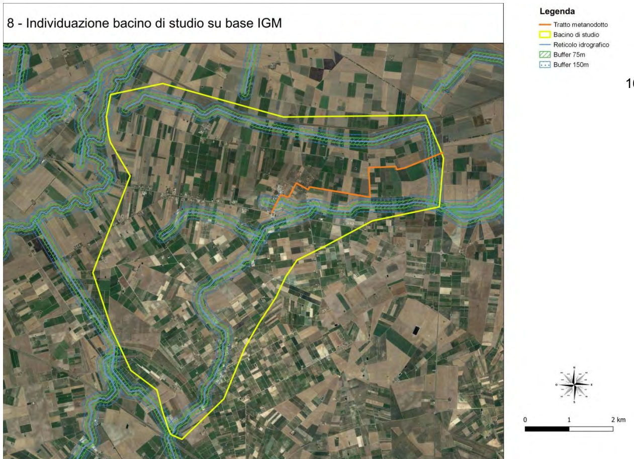
Figure 8 - Individuazione bacino di studio su base IGM
