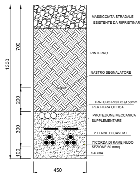
SEZIONE F-F CAVIDOTTO MT INTERRATO - 2 TERNE DI CAVI PERCORSO IN MASSICCIATA scala 1:20
