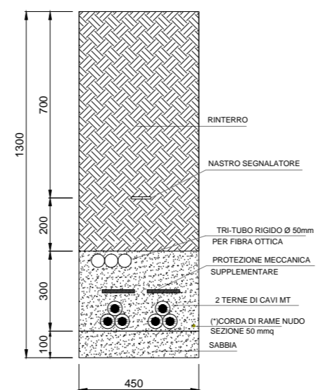
SEZIONE G-G CAVIDOTTO MT INTERRATO - 2 TERNE DI CAVI PERCORSO IN TERRENO scala 1:20
