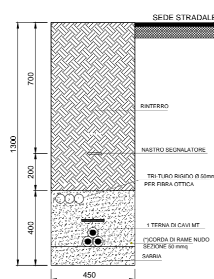
SEZIONE C-C CAVIDOTTO MT INTERRATO - 1 TERNA DI CAVI PERCORSO IN BANCHINA STRADA PROVINCIALE
