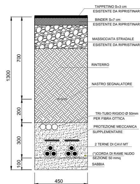
SEZIONE E-E CAVIDOTTO MT INTERRATO - 2 TERNE DI CAVI PERCORSO IN ASFALTO scala 1:20
