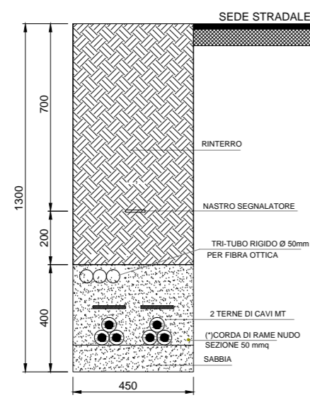
SEZIONE D-D CAVIDOTTO MT INTERRATO - 2 TERNE DI CAVI PERCORSO IN BANCHINA STRADA PROVINCIALE
