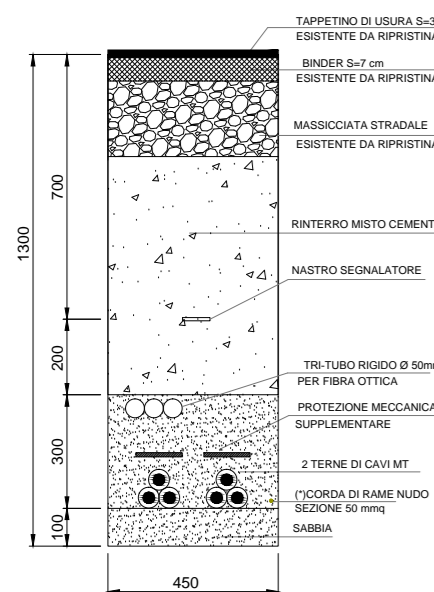
SEZIONE D-D CAVIDOTTO MT INTERRATO - 2 TERNE DI CAVI PERCORSO IN ASFALTO STRADA PROVINCIALE
