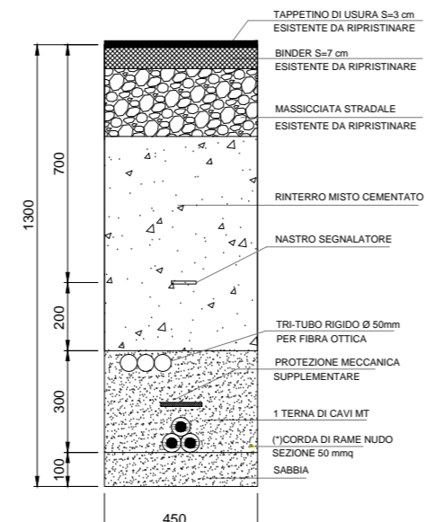
SEZIONE C-C CAVIDOTTO MT INTERRATO - 1 TERNA DI CAVI PERCORSO IN ASFALTO STRADA PROVINCIALE
