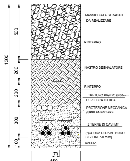
SEZIONE B-B CAVIDOTTO MT INTERRATO - 2 TERNE DI CAVI PERCORSO STRADA DI CANTIERE scala 1:20
