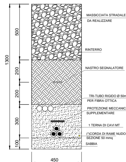
SEZIONE A-A CAVIDOTTO MT INTERRATO - 1 TERNA DI CAVI PERCORSO STRADA DI CANTIERE scala 1:20
