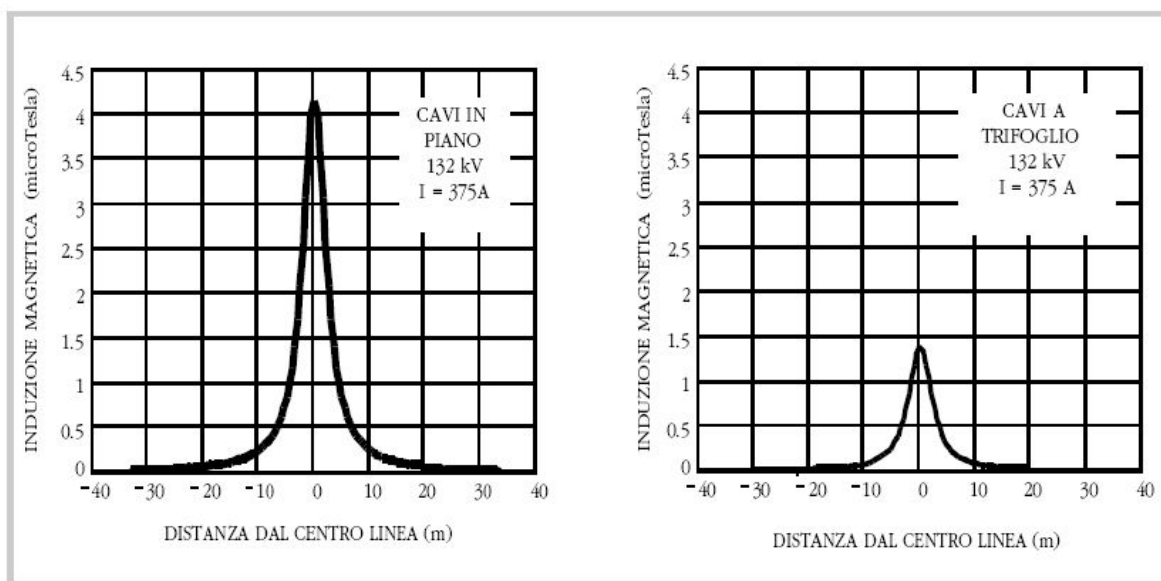
Fig. 7.6 Profili laterali dell'induzione magnetica relativa ai due tipici sistemi in cavo interrato riportati in Fig 7.5
