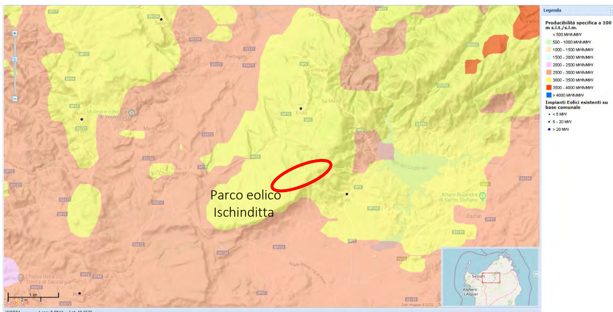
Figura 6 - Tavola 2 Producibilità media annua dall'Atlante Eolico Interattivo http://atlanteolico.rse-web.it/viewer.htm
