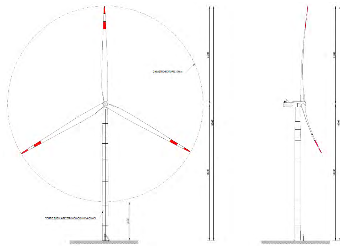
Figura 7 – Schema geometrico degli aerogeneratori in progetto V150.
