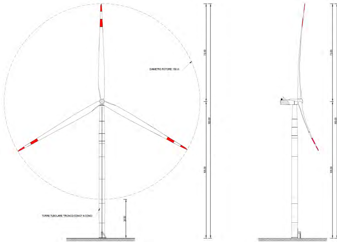
Figura 4 – Schema geometrico degli aerogeneratori in progetto V150.
