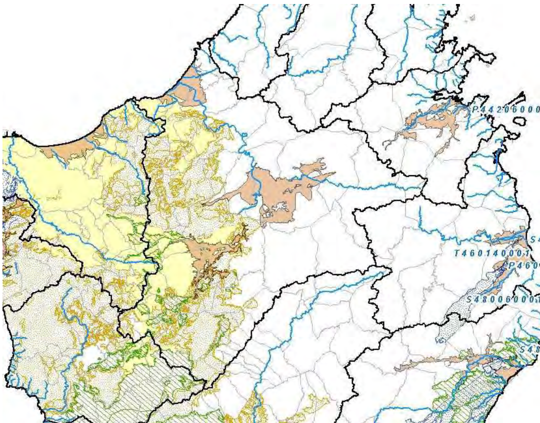
Figura 7: Complessi acquiferi presenti nella U.I.O. del Coghinas
