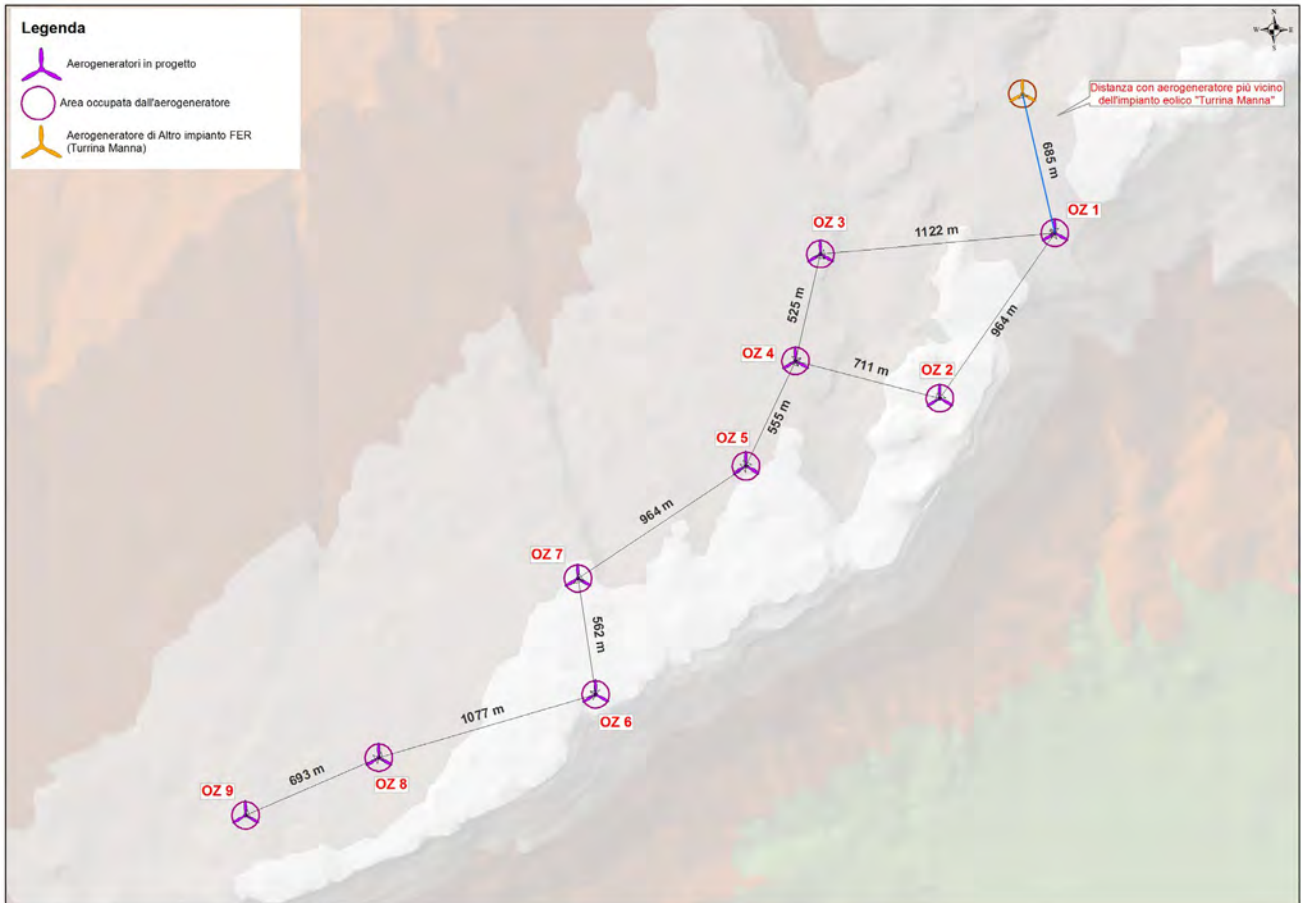
Figura 35 - Planimetria semplificativa delle interdistanze tra gli aerogeneratori in progetto e gli aerogeneratori dell'impianto eolico ENEL di "Sa Turrina Manna - Tula(SS)"
