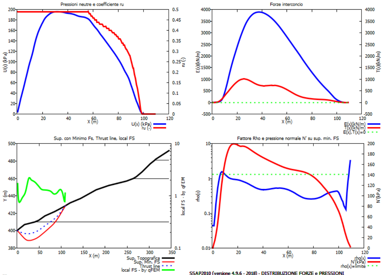
SSAP2010 (versione 4.9.6 - 2018) - DISTRIBUZIONE FORZE e PRESSIONI
