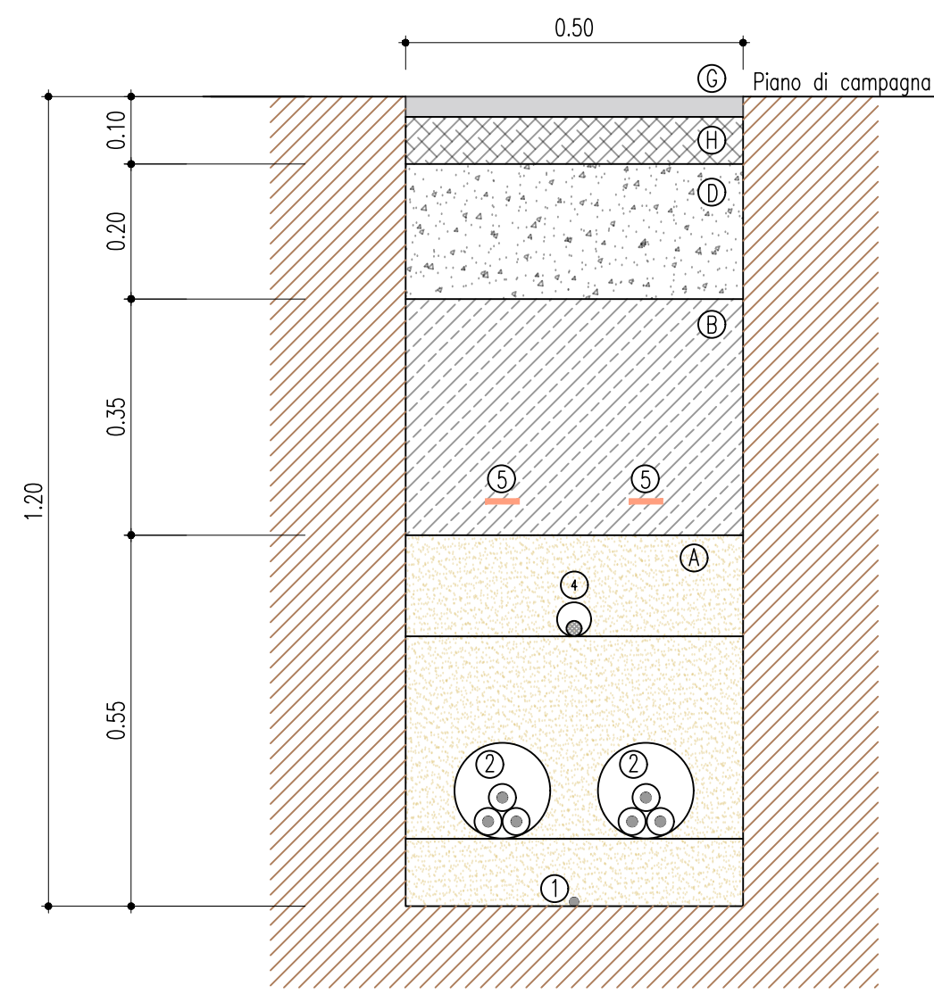
SEZIONE TIPO 2B - SU STRADE ASFALTATE
