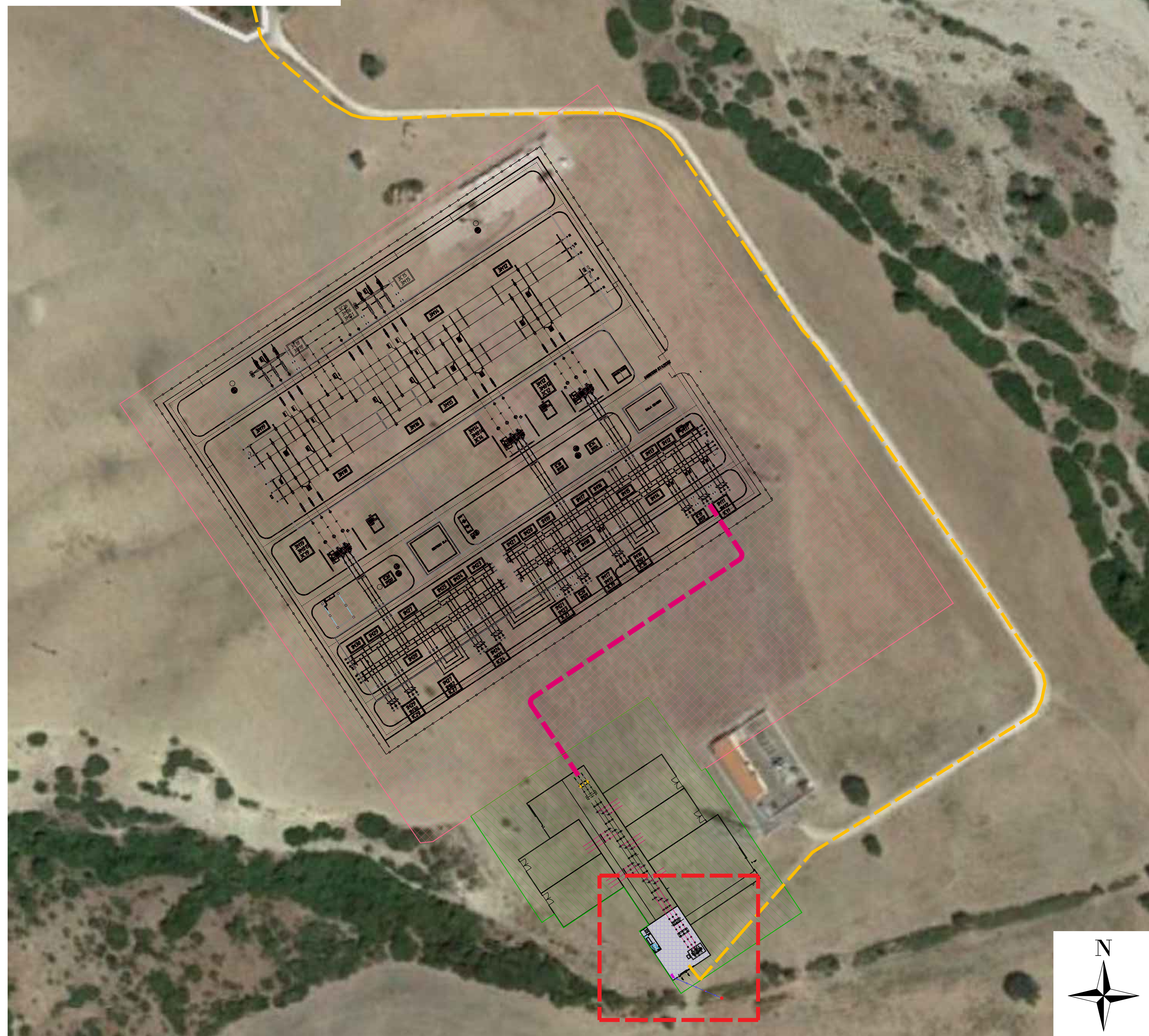
PLANIMETRIA DELLA STAZIONE ELETTRICA (SCALA 1:1.000)
