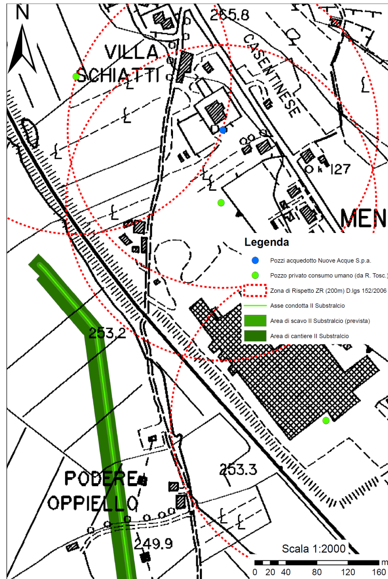
Figura 4 – Posizione dei pozzi privati per consumo umano, dei pozzi dell'acquedotto gestiti da Nuove Acque S.p.a. e relativa Zona di Rispetto di 200 m, in relazione alle aree di scavo e di occupazione del cantiere necessarie alla realizzazione della condotta.
