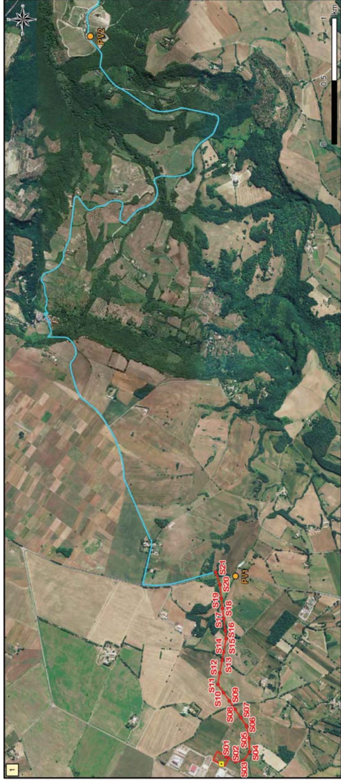
Tracciato Elettrodotto su ORTOFOTO con punti di ripresa dei fotoinserimenti
