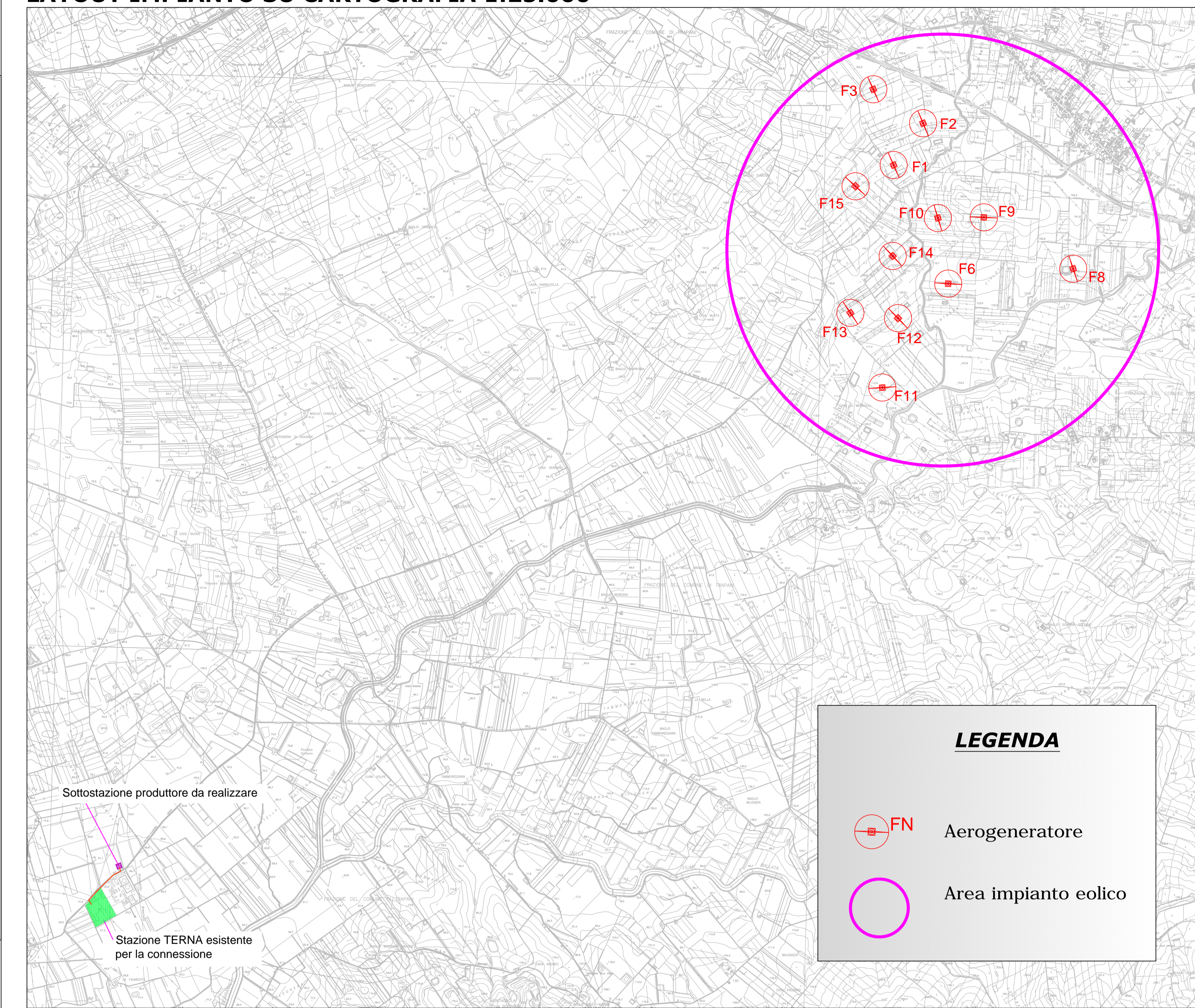
LAYOUT IMPIANTO SU CARTOGRAFIA 1:25.000
