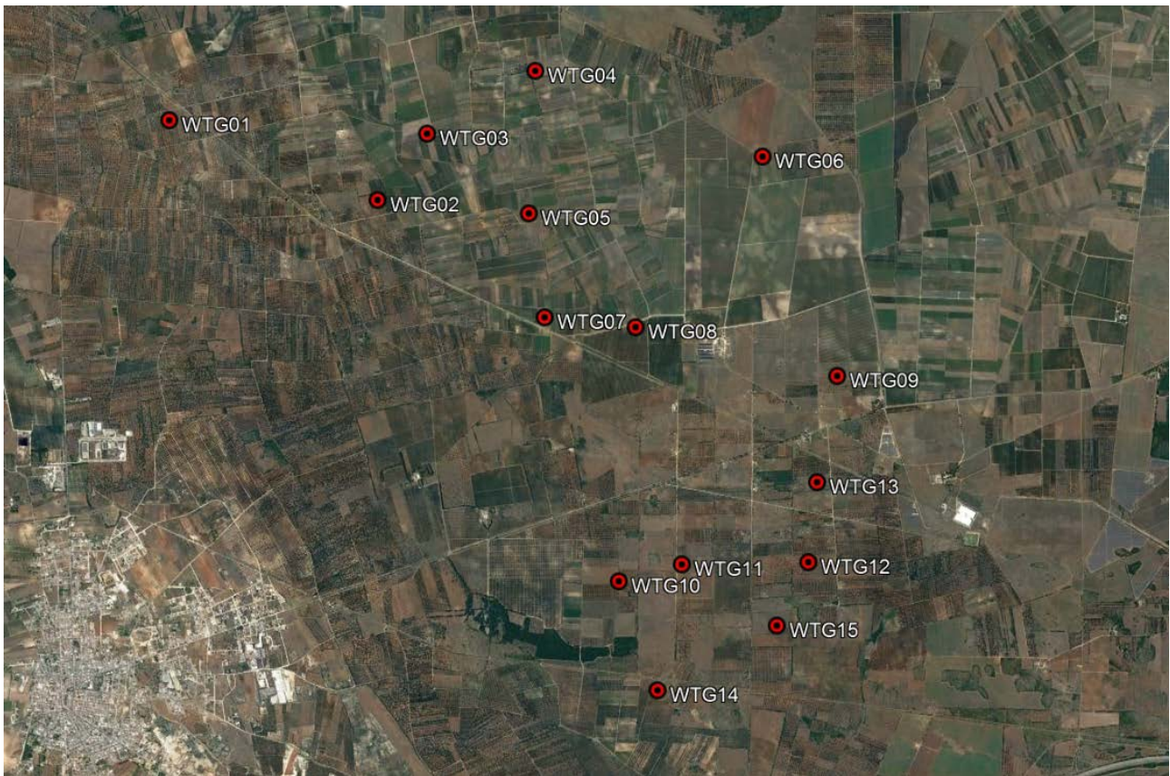
Fig. 1 - Layout del parco eolico su ortofoto
