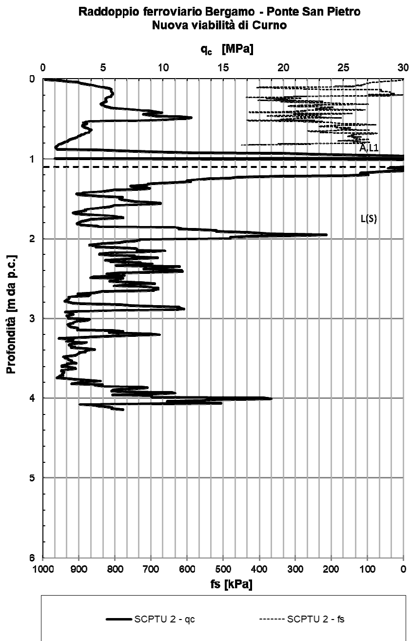
Figura 6: q_c da SCPTU-03
