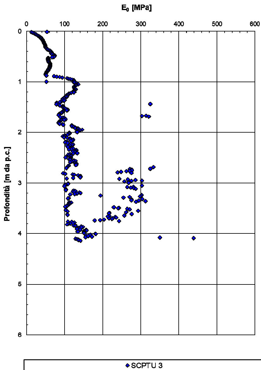
Figura 17: Modulo di Young iniziale da SCPTU-03
