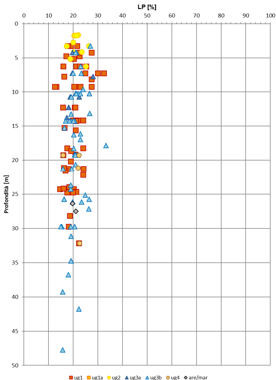
Figura 42: Limite plastico
