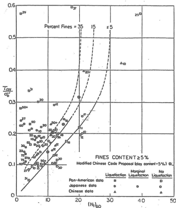
Figura 49: Relazione tra sforzo di taglio ciclico a liquefazione e N_{1(60)} – sisma di riferimento Magnitudo = 7.5 (Seed et al., 1985).
