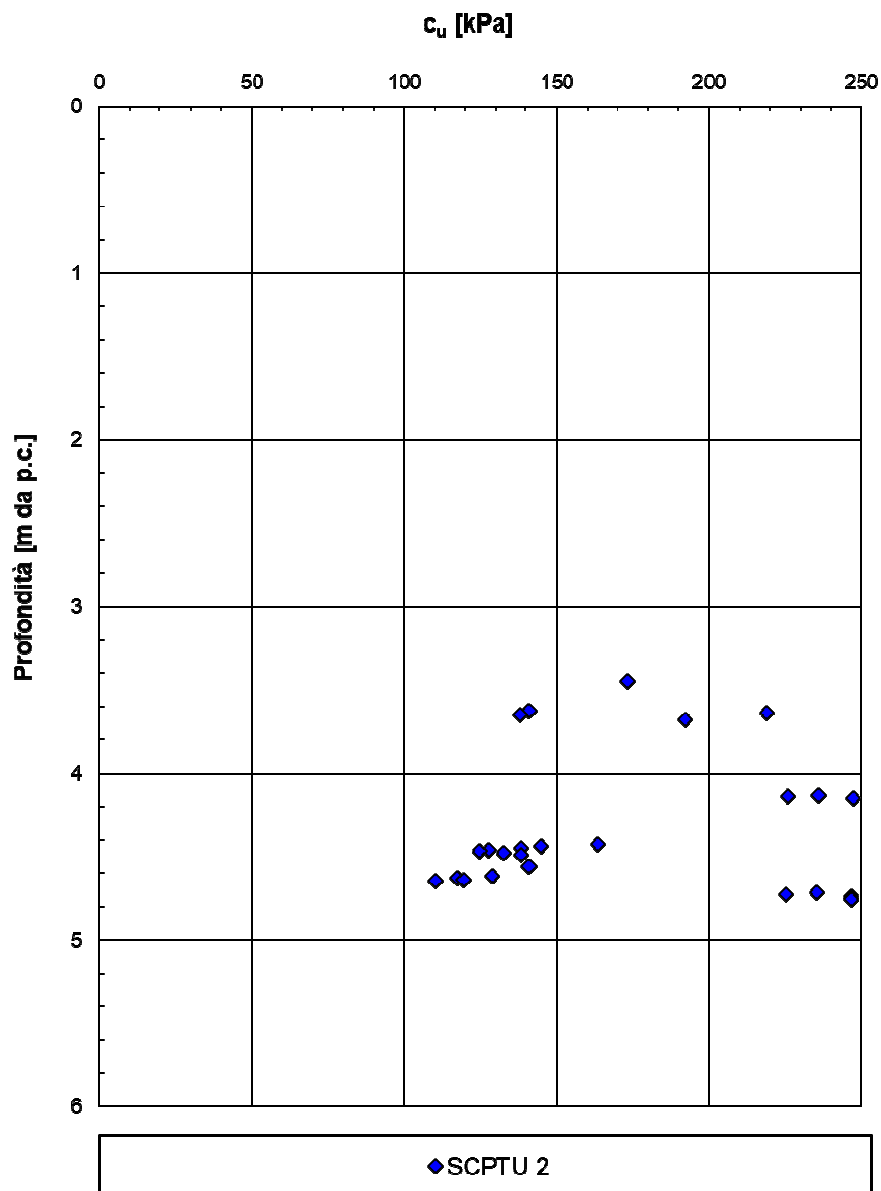
Figura 26:: Coesione non drenata da SCPTU-02
