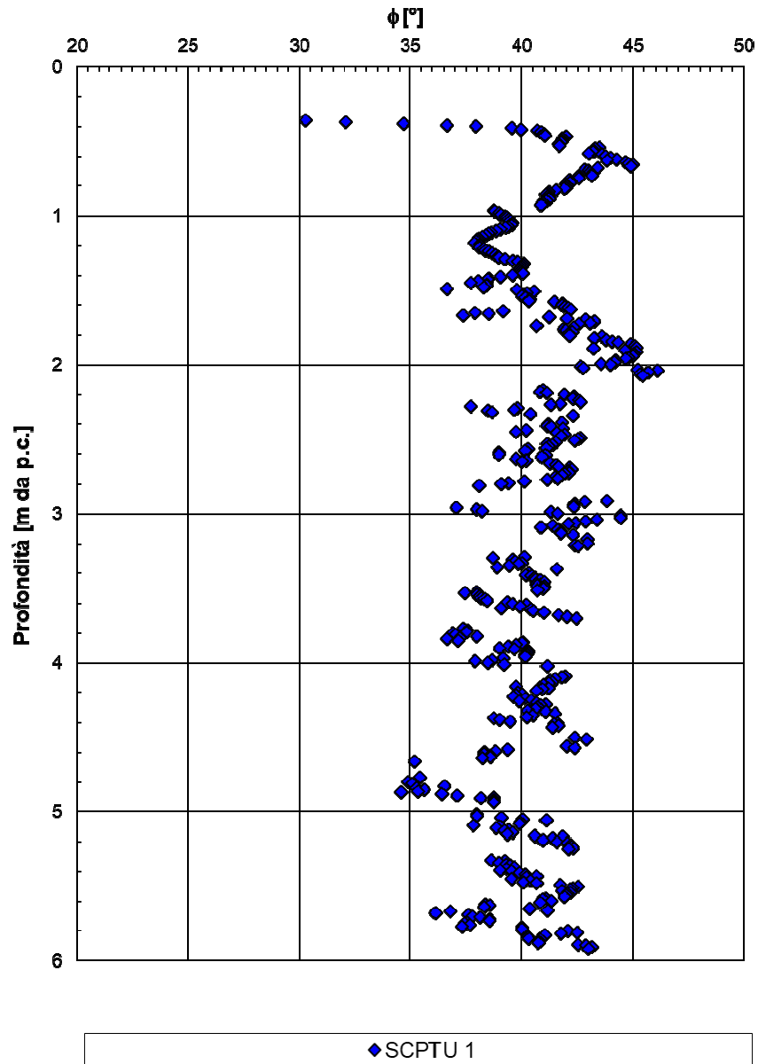
Figura 33: Angolo di resistenza al taglio da da SCPTU-01
