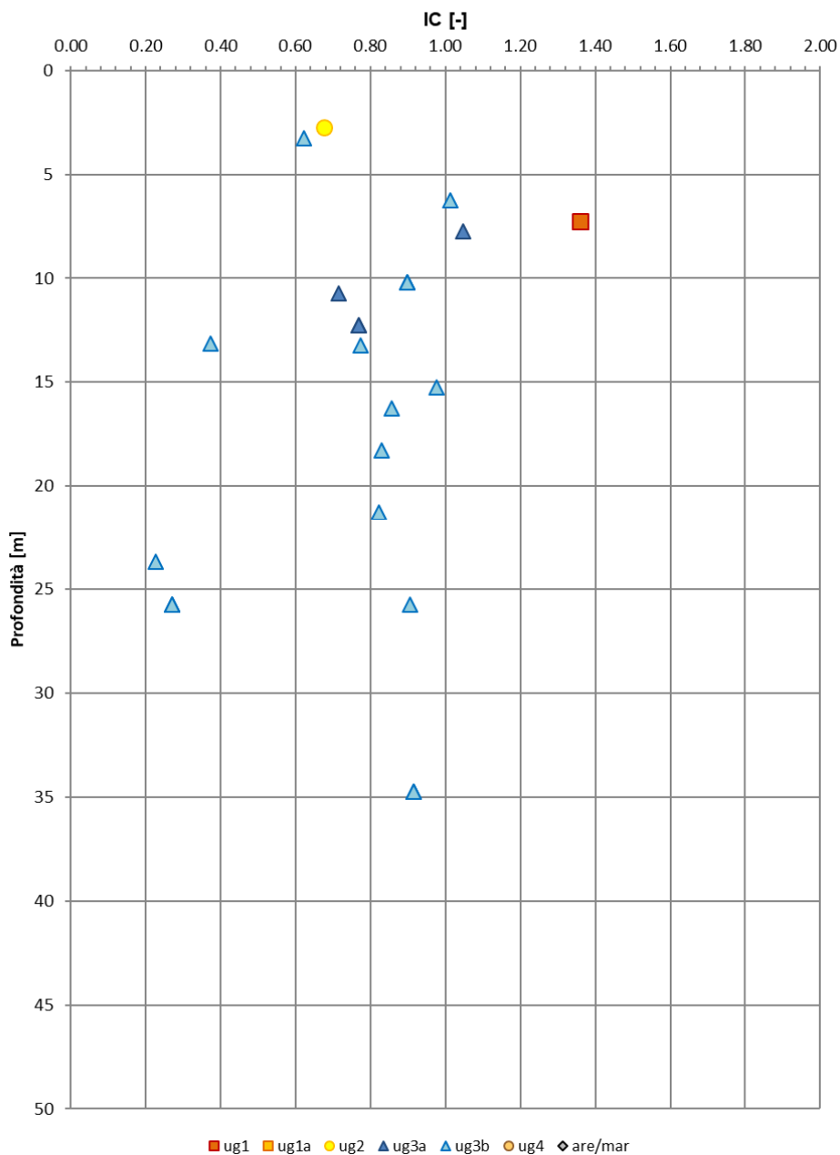
Figura 45: Indice di consistenza
