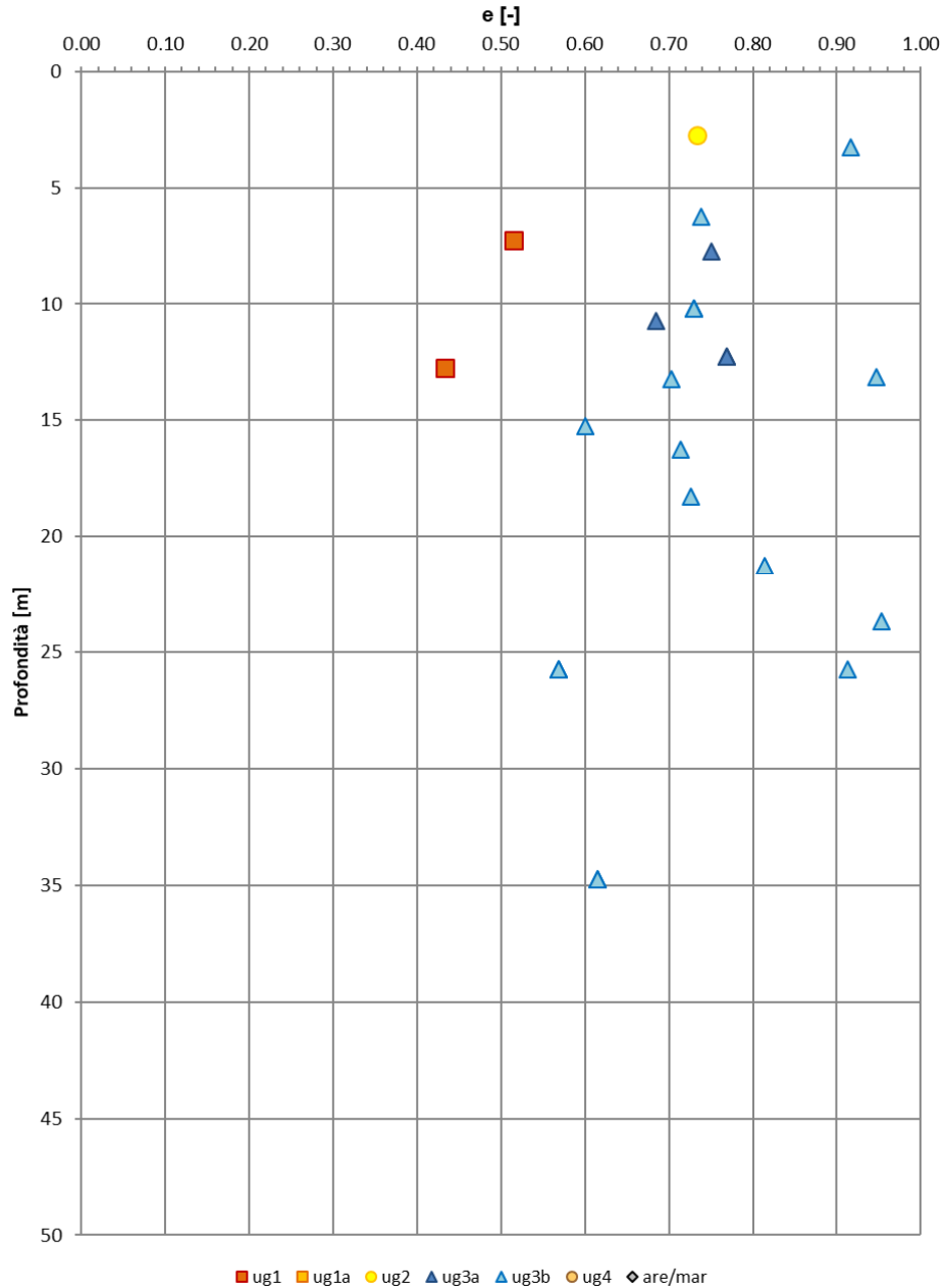
Figura 40: Indice dei vuoti iniziale
