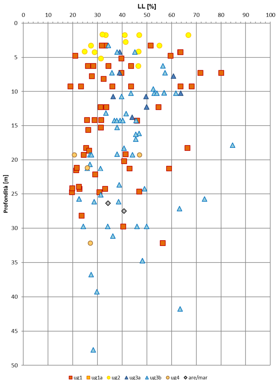
Figura 41: Limite liquido
