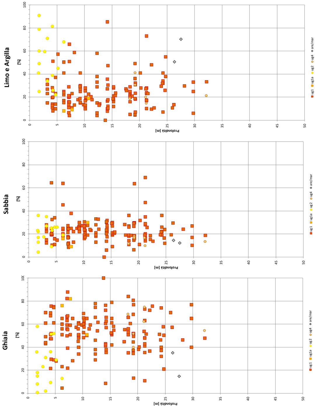
Figura 37: Composizione granulometrica Materiali granulari
