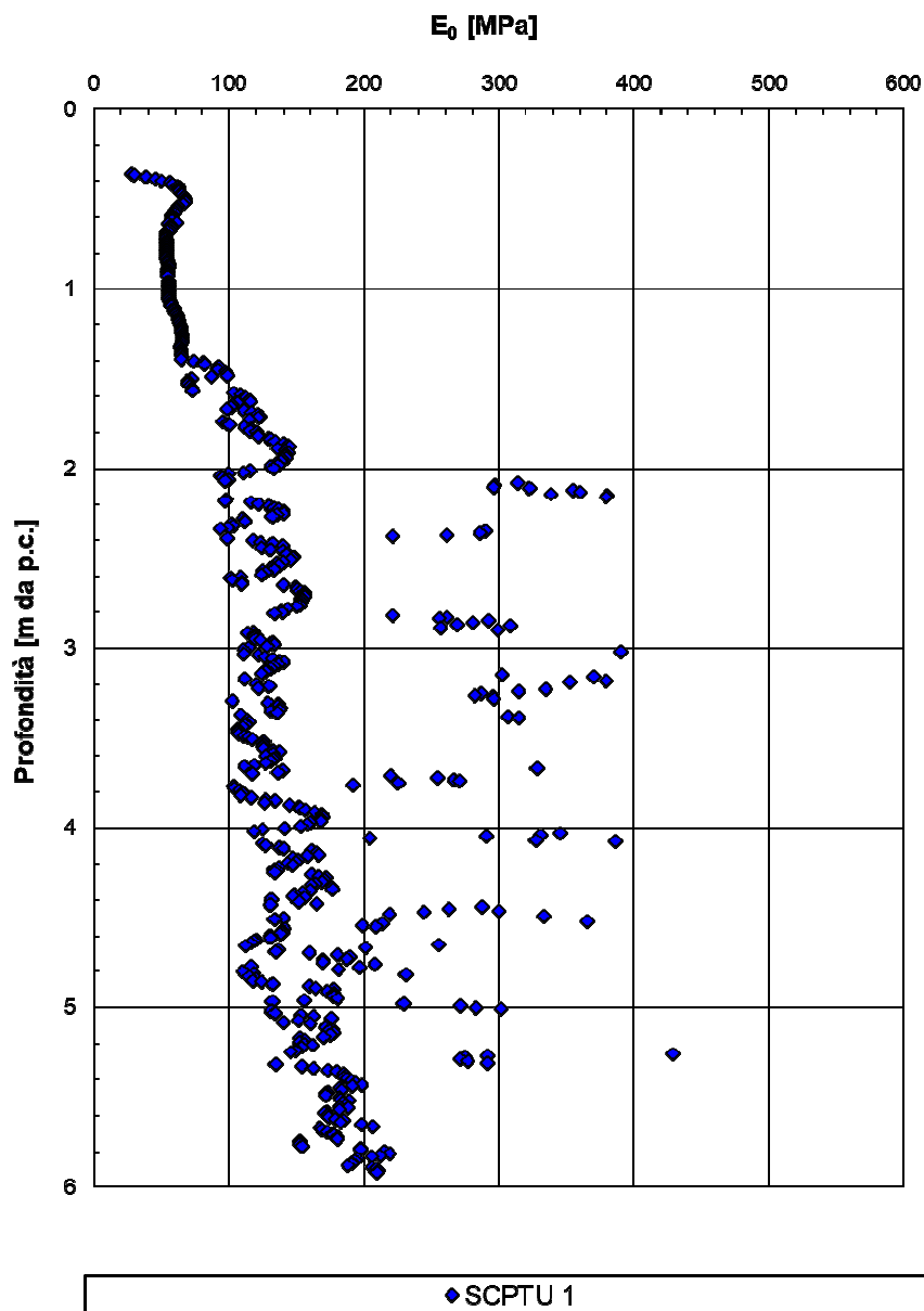
Figura 15: Modulo di Young iniziale da SCPTU-01
