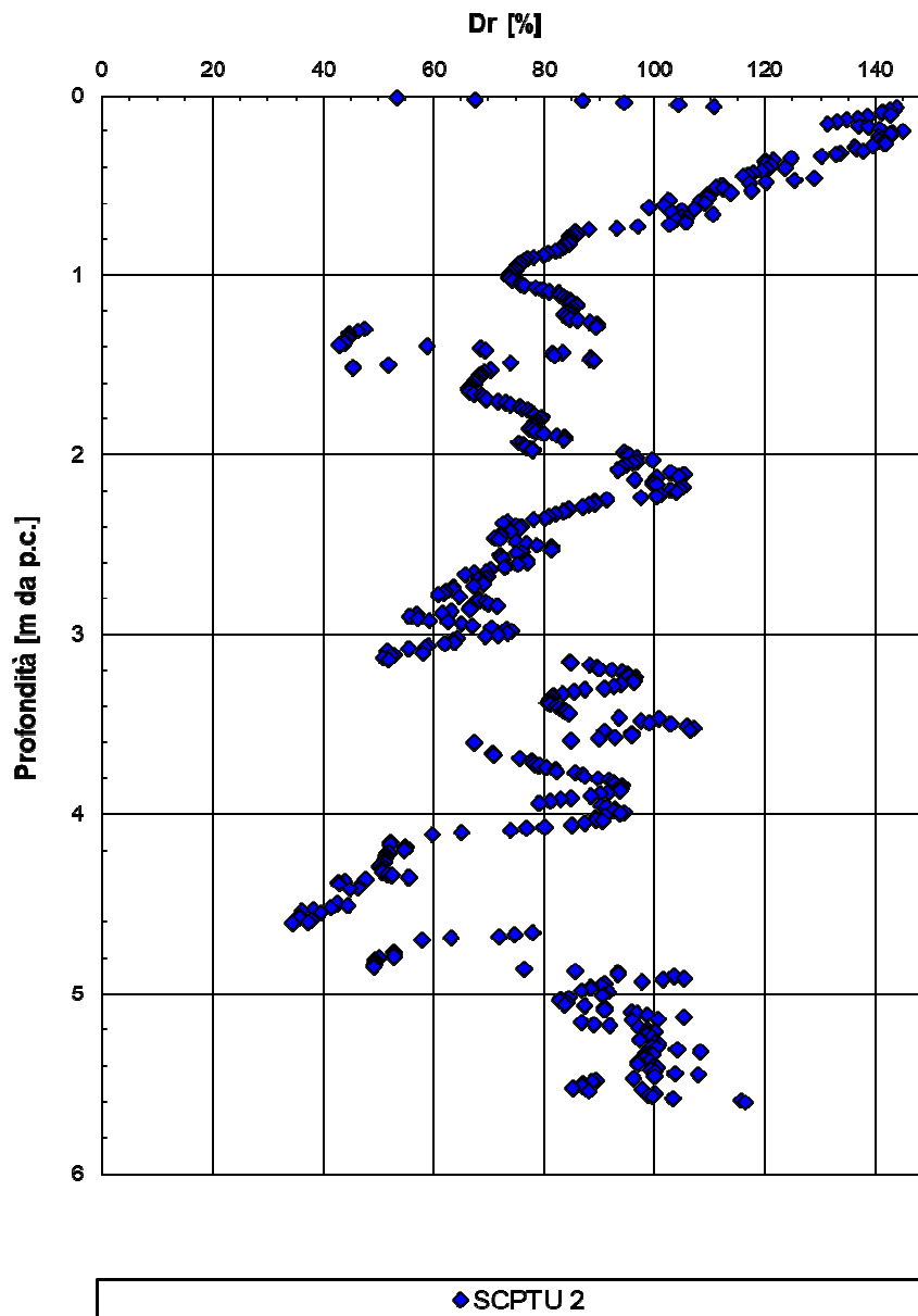
Figura 30: Densità relativa da SCPTU-02
