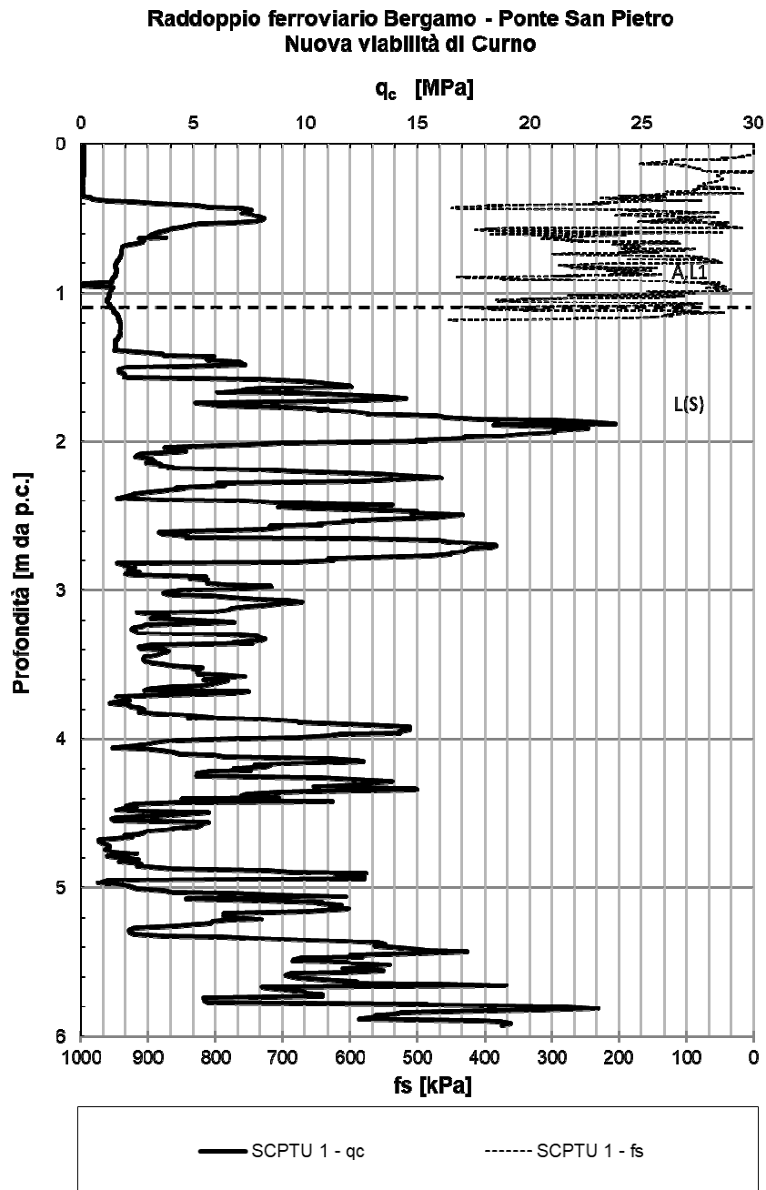
Figura 4: q_c da SCPTU-01
