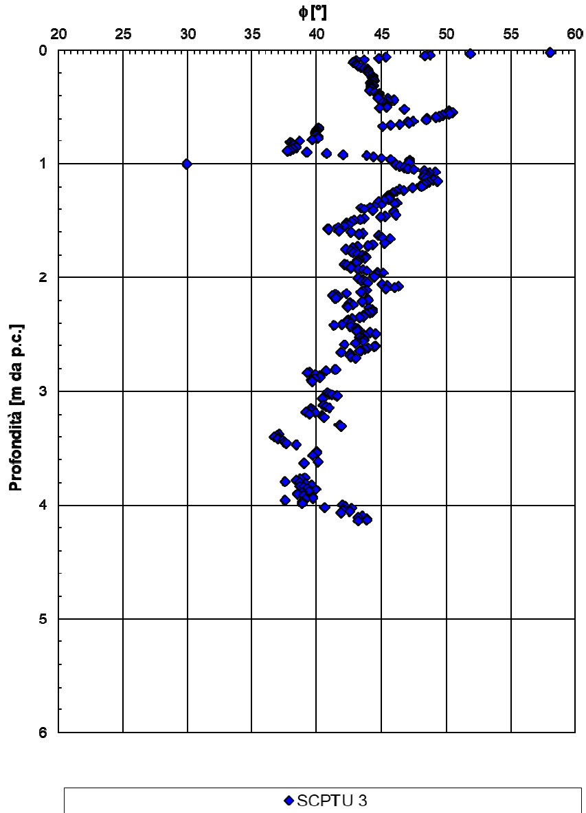
Figura 35: Angolo di resistenza al taglio da SCPTU-03
