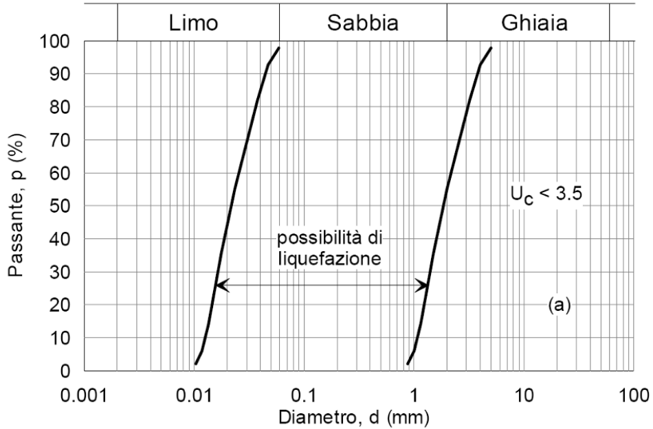
Figura 47: Dominio di suscettibilità alla liquefazione dei terreni ( U_c < 3.5 )
