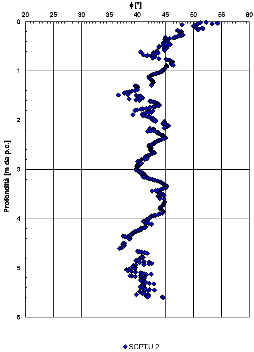
Figura 34: Angolo di resistenza al taglio da SCPTU-02
