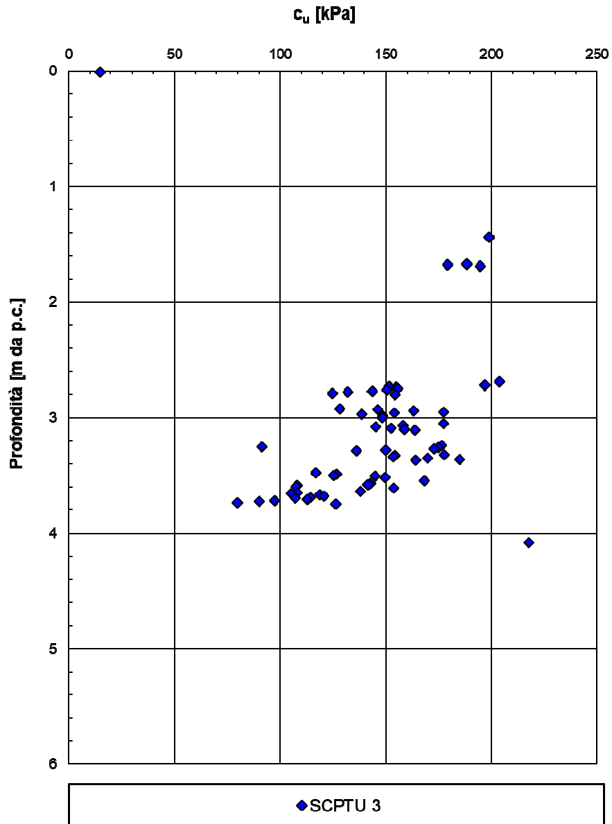
Figura 27:: Coesione non drenata da SCPTU-03
