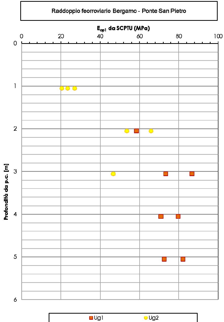
Figura 23: Modulo di Young operativo da Vs di SCPTU
