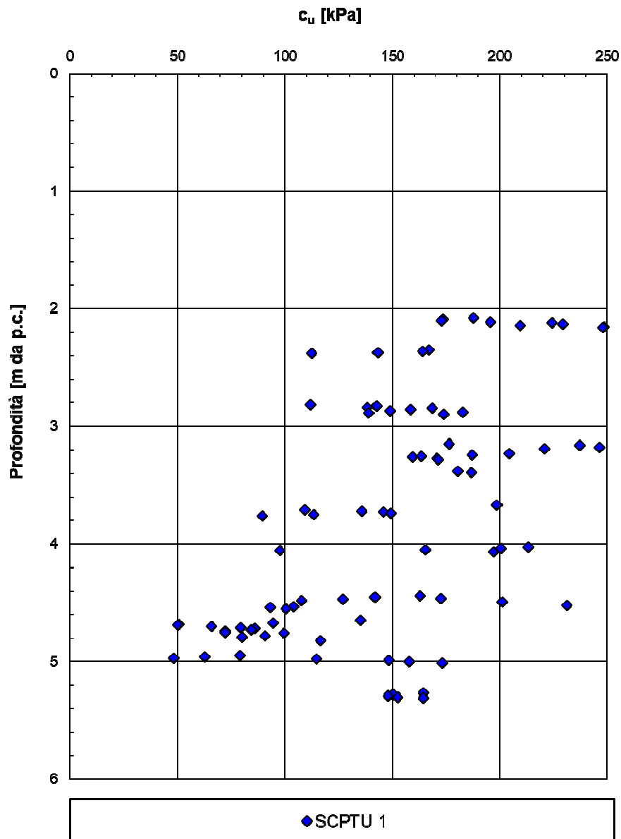
Figura 25:: Coesione non drenata da SCPTU-01
