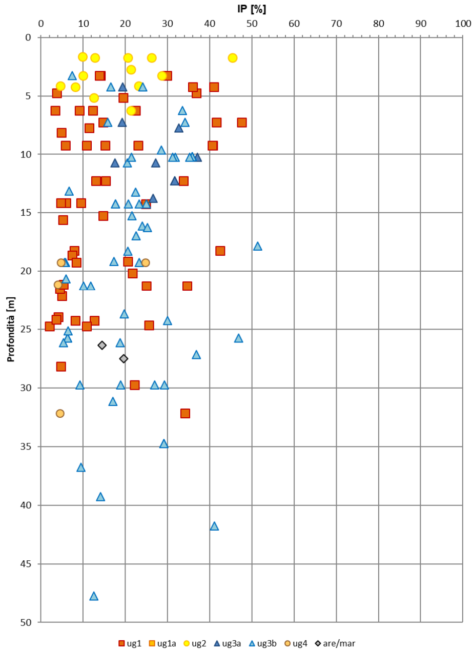
Figura 43: Indice di plasticità
