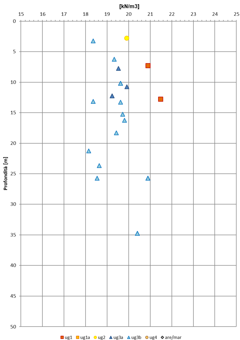
Figura 36: Pesi dell' unità di volume
