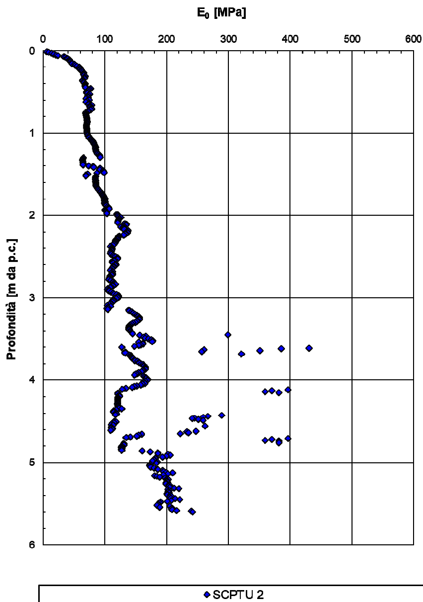
Figura 16: Modulo di Young iniziale da SCPTU-02
