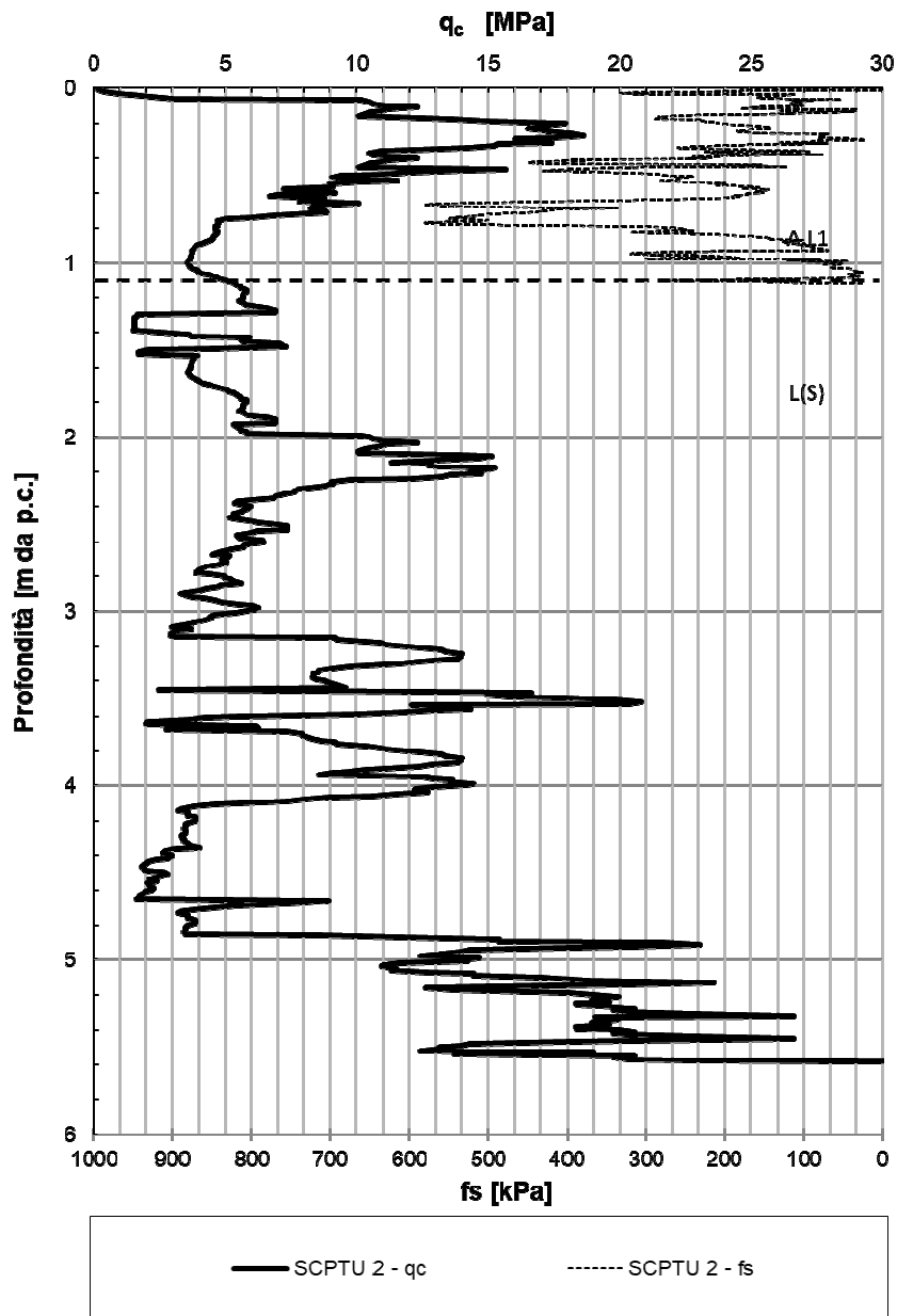
Figura 5: q_c da SCPTU-02
