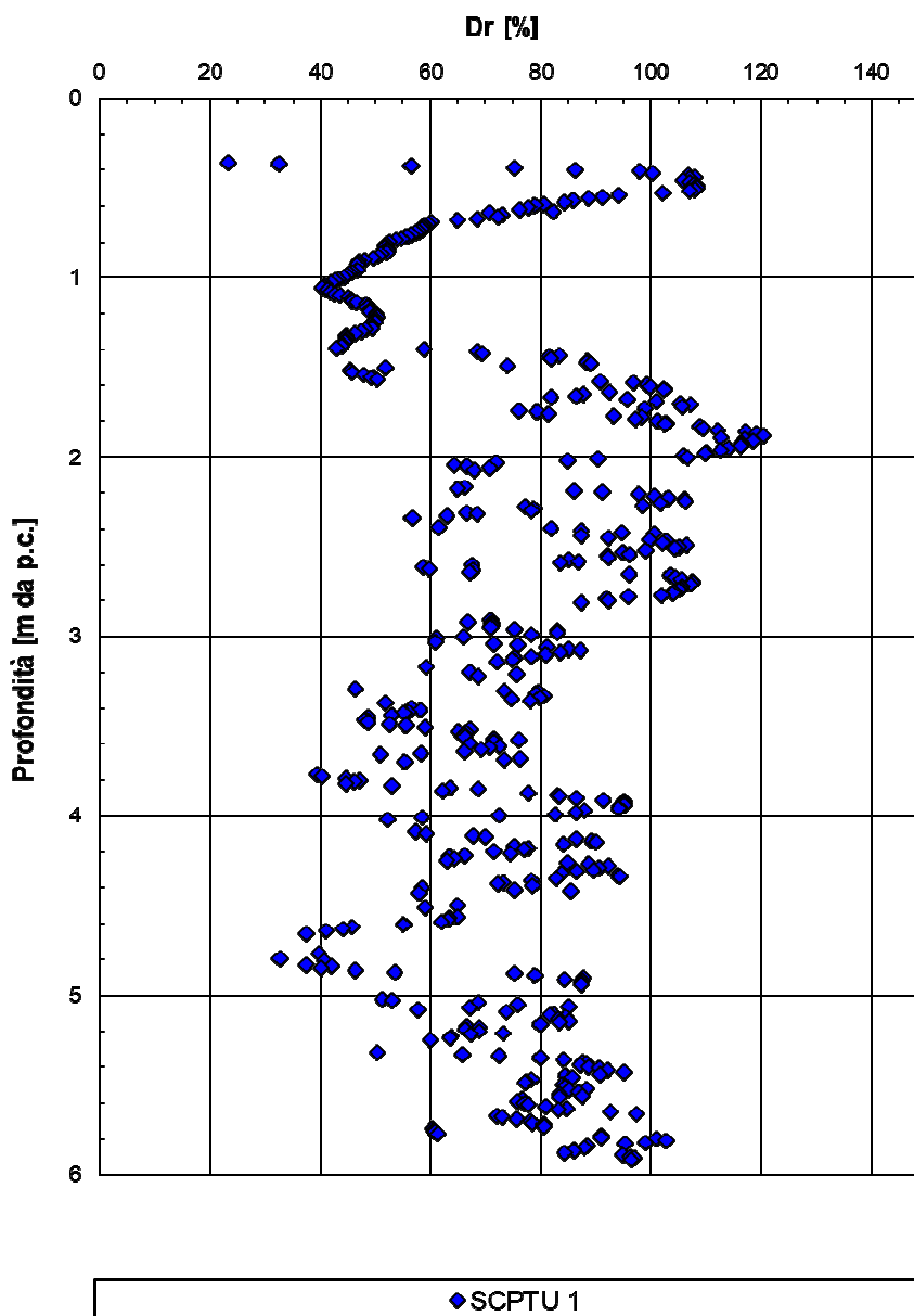
Figura 29: Densità relativa da SCPTU-01
