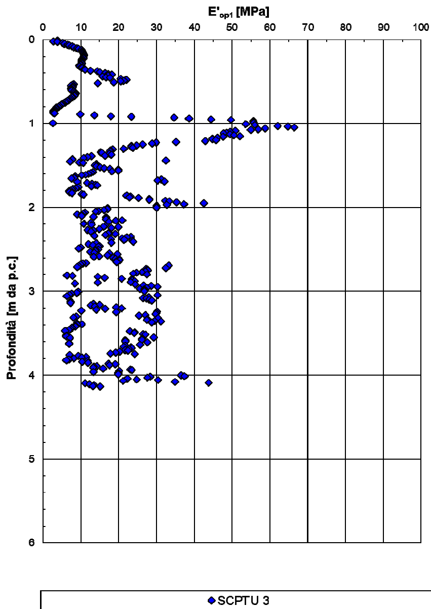
Figura 22: Modulo di Young operativo da SCPTU-03
