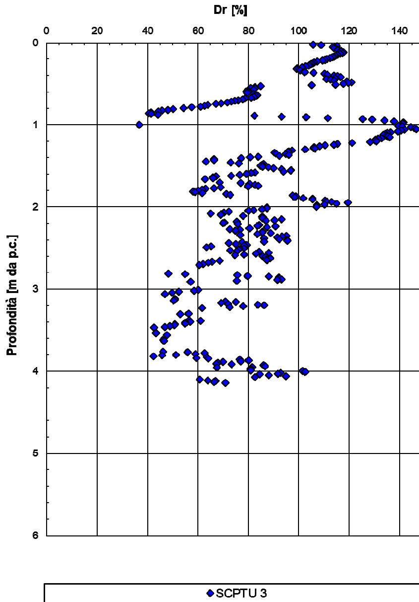
Figura 31: Densità relativa da SCPTU-03
