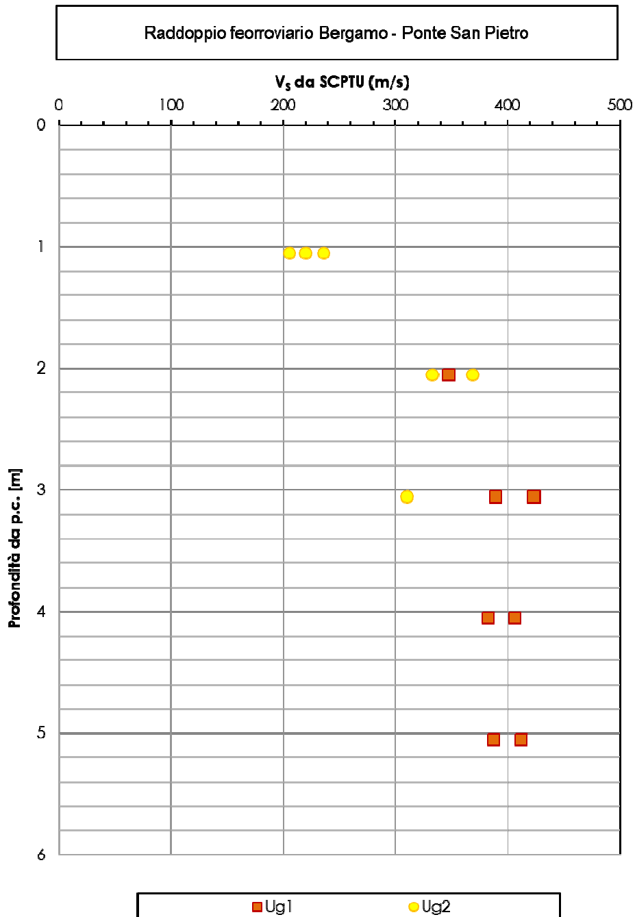
Figura 10: Vs da SCPTU
