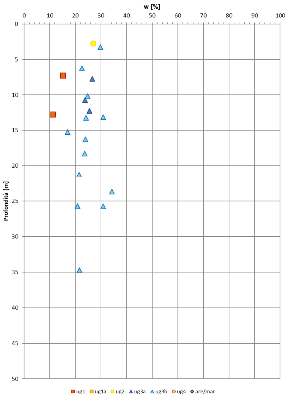
Figura 39: Contenuto naturale d'acqua
