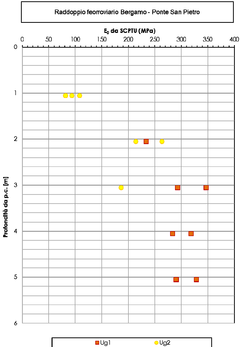
Figura 18: Modulo di Young iniziale da Vs di SCPTU
