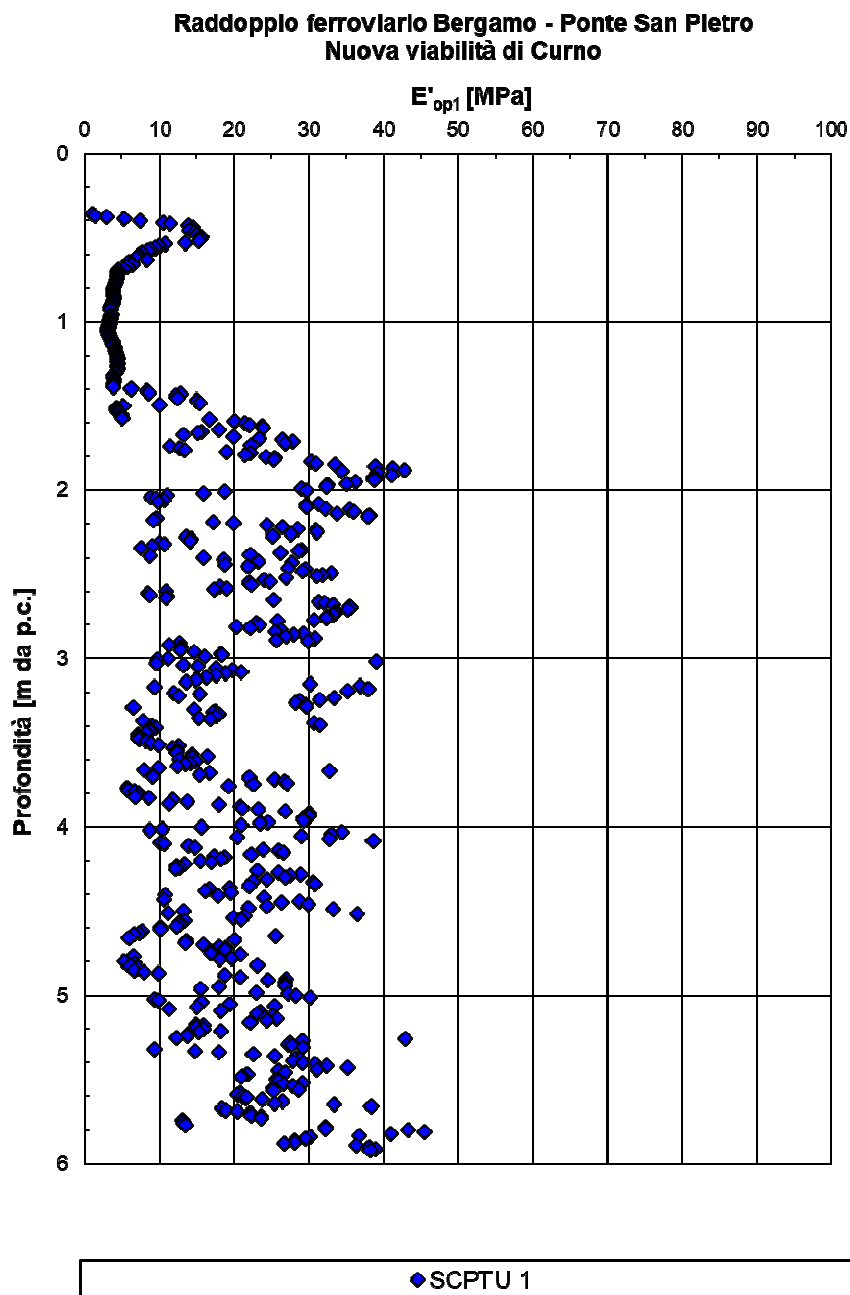
Figura 20: Modulo di Young operativo da SCPTU-01
