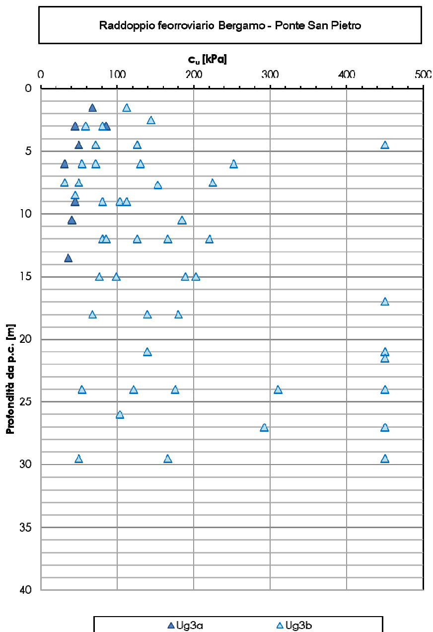
Figura 24.: Coesione non drenata da SPT
