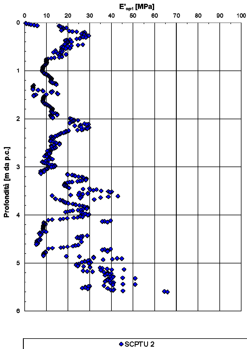
Figura 21: Modulo di Young operativo da SCPTU-02
