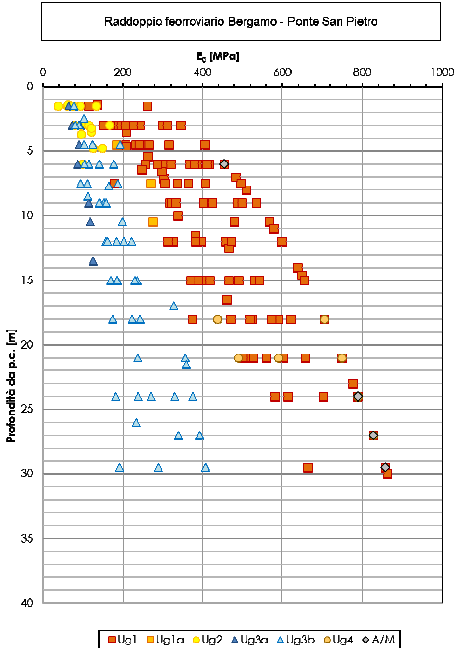
Figura 14: Modulo di Young iniziale da SPT
