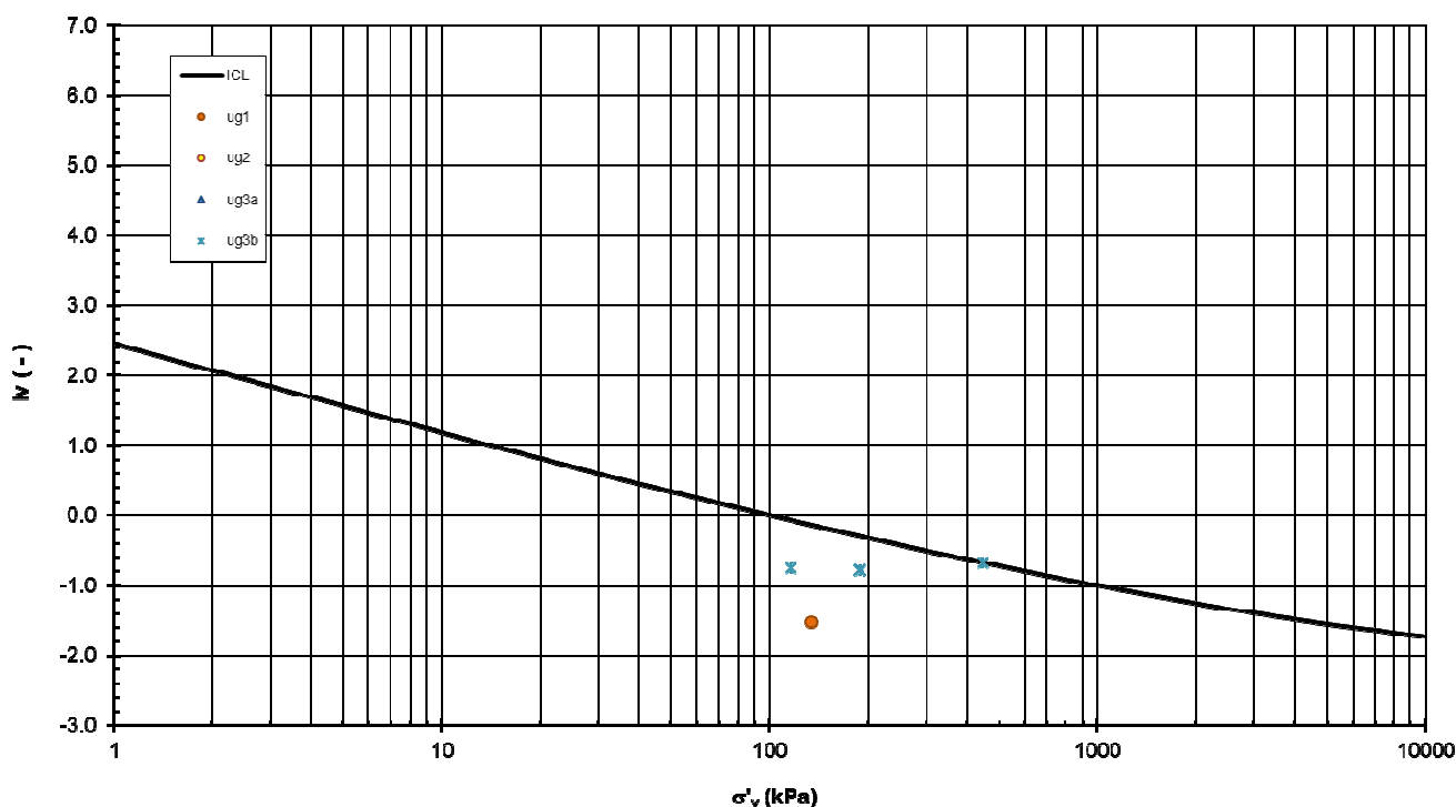
Figura 46: Curva di compressione intrinseca e indice dei vuoti in sito (Burland, 1990)
