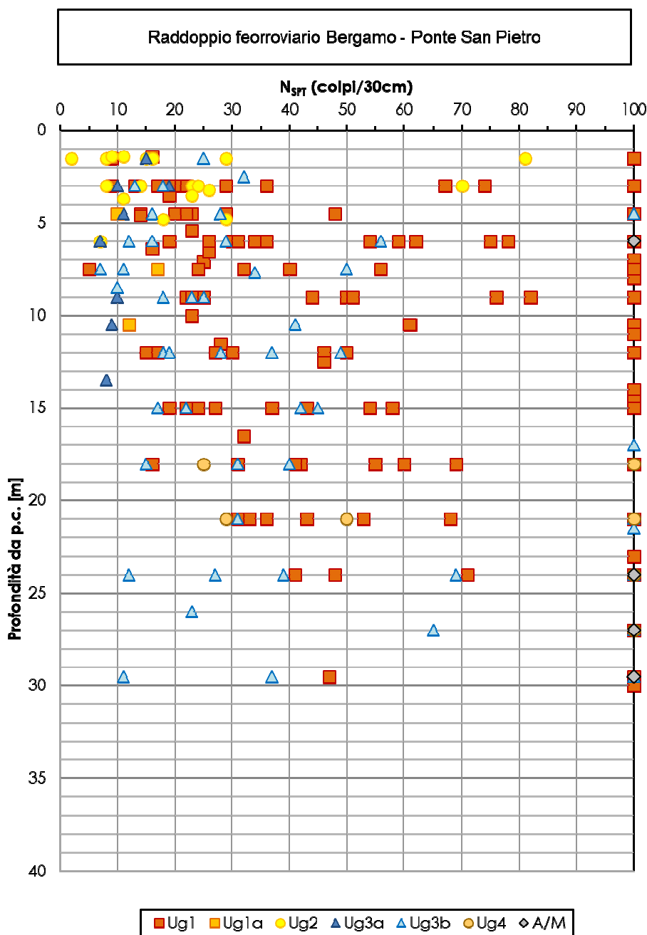
Figura 7: N spt
