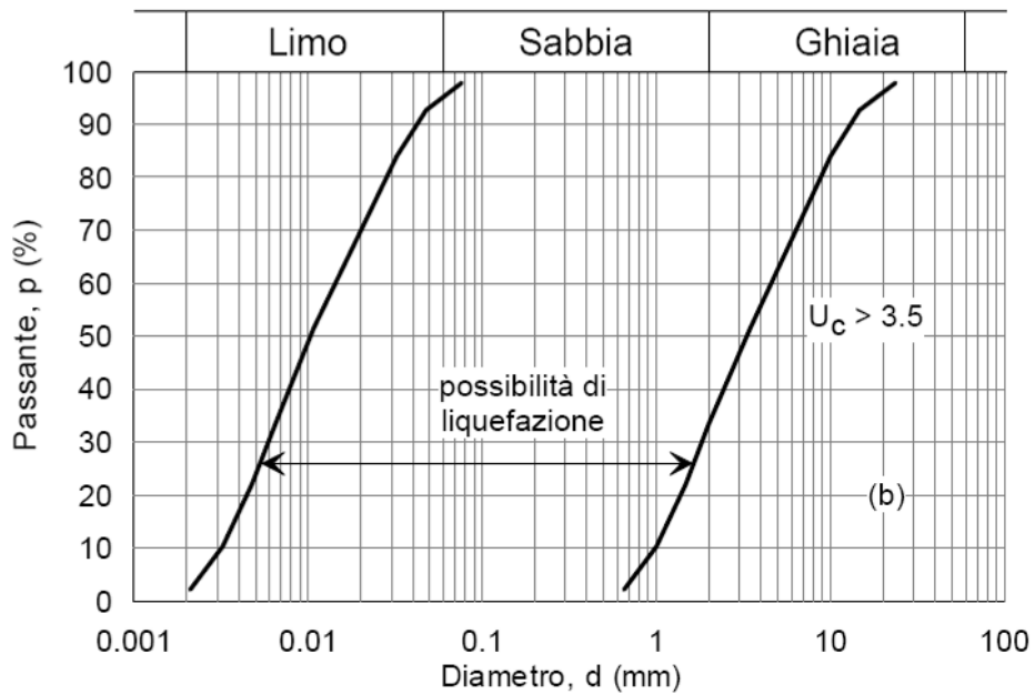
Figura 48: Dominio di suscettibilità alla liquefazione dei terreni ( U_c > 3.5 )
