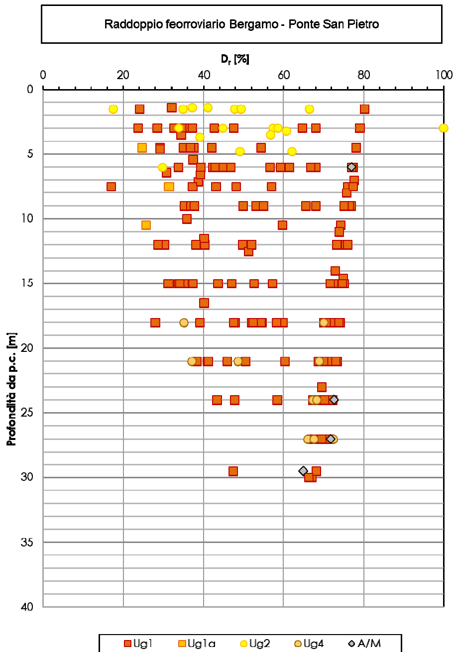
Figura 28: Densità relativa da SPT
