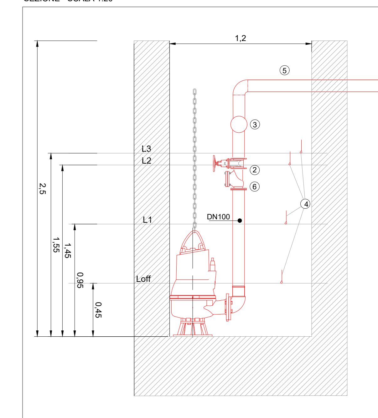
SEZIONE - SCALA 1:20
