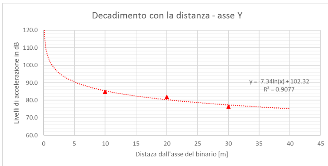
Figura 4-2 Curva di attenuazione del Leq_{te} in funzione della distanza dal binario, ricavata dai rilievi lungo l'asse Y, in corrispondenza della Terna 1 (10metri), della Terna 2 (20 metri) e della Terna 3 (30 metri) e relativa al totale dei transiti ferroviari rilevati durante il periodo di osservazione.
