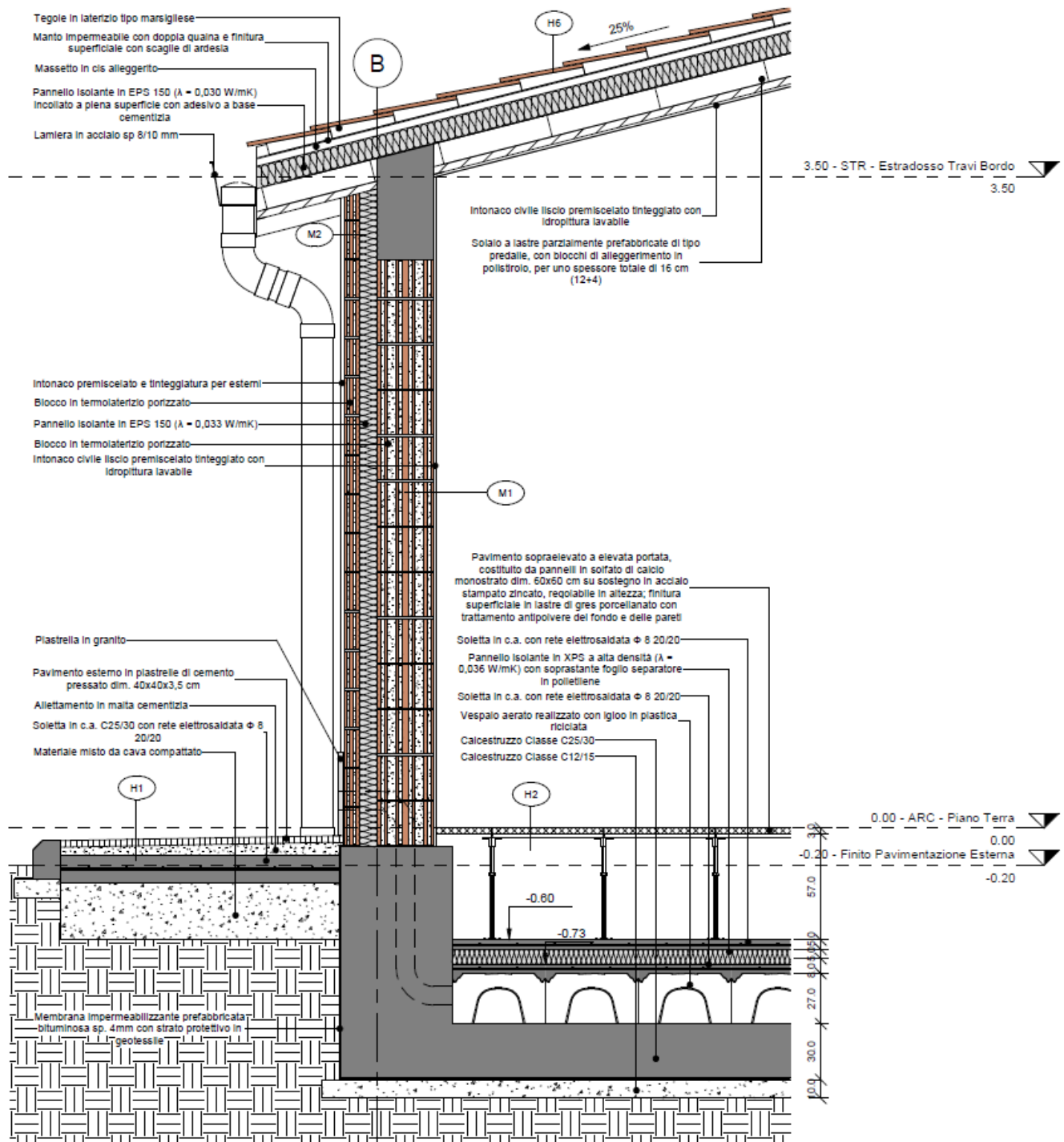
Figura 9 - Dettagli Costruttivi – Nodo di copertura e di piano
