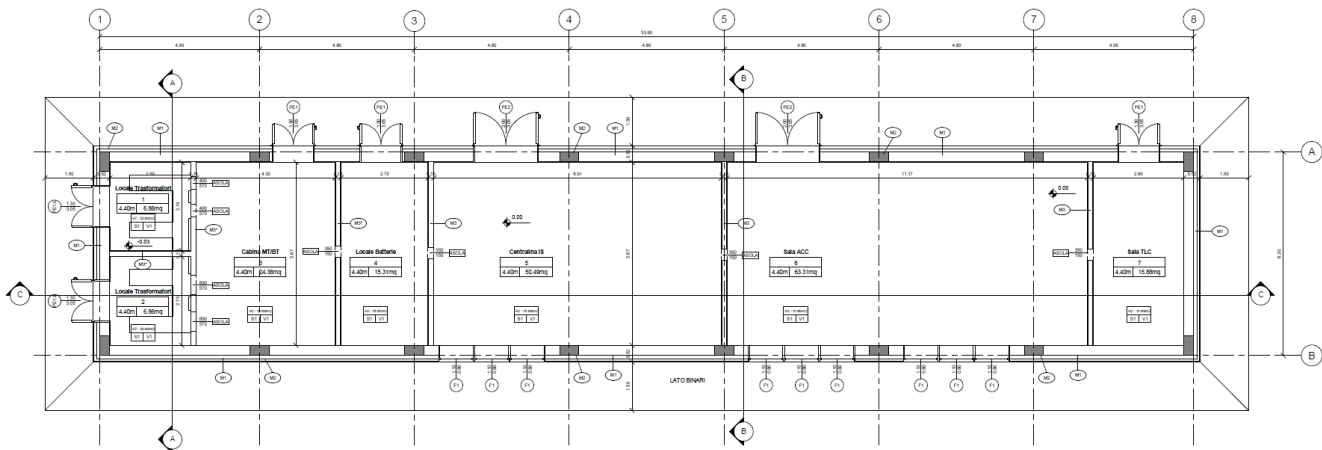
Figura 6 - Pianta Piano Terra
