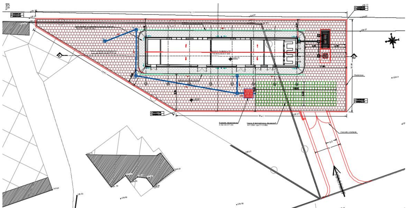
Figura 13 - Drenaggio piazzale
