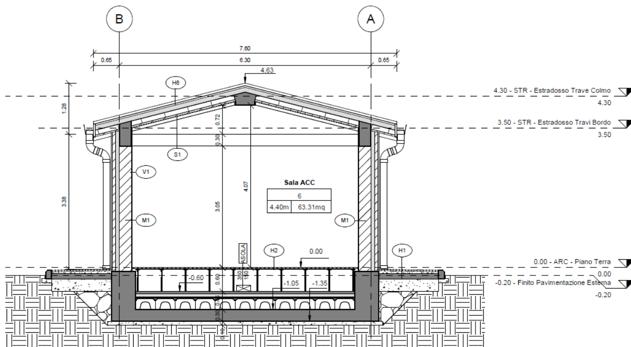
Figura 7 - Sezione Trasversale del fabbricato
