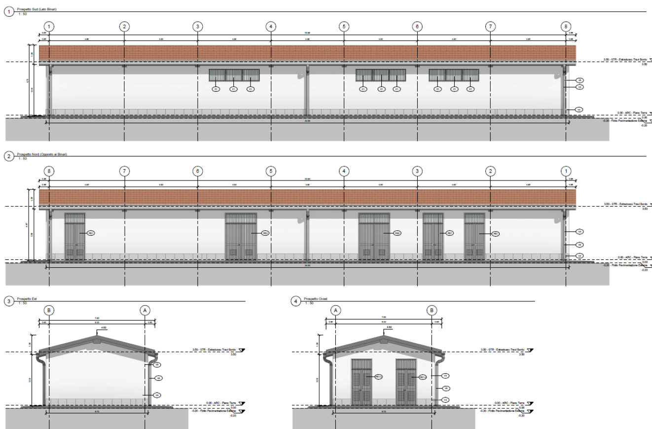
Figura 10 - Prospetti del fabbricato
