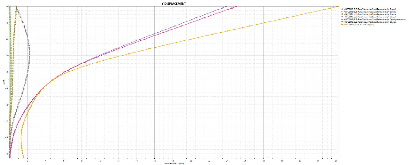
Figura 18: Spostamenti nominali della paratia nelle principali fasi
