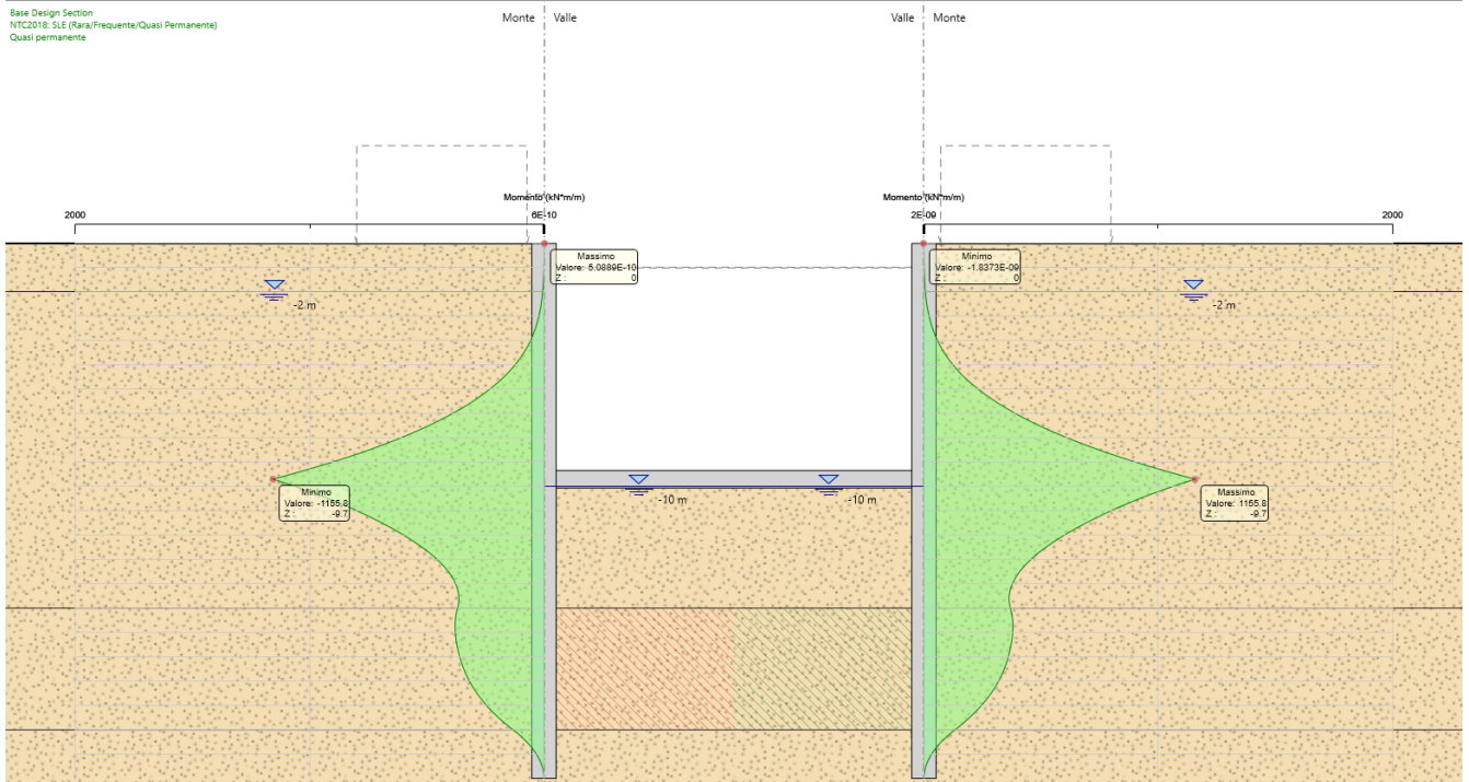
Figura 15: Diagramma dei momenti agli SLE r (in fase di esercizio)
