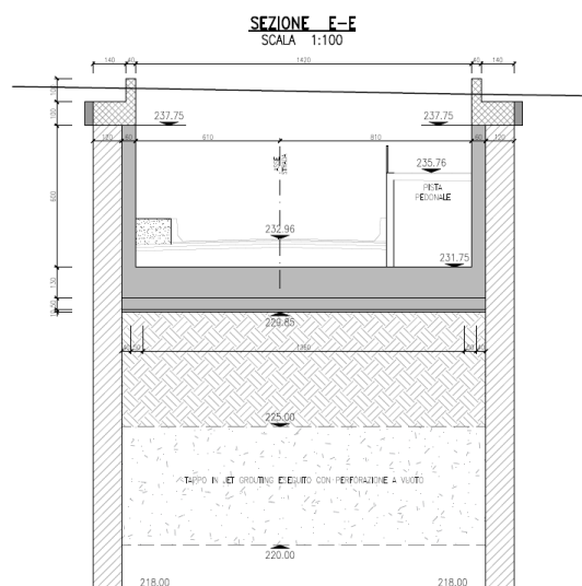
Figura 1: Sezione trasversale tipo con arredo
