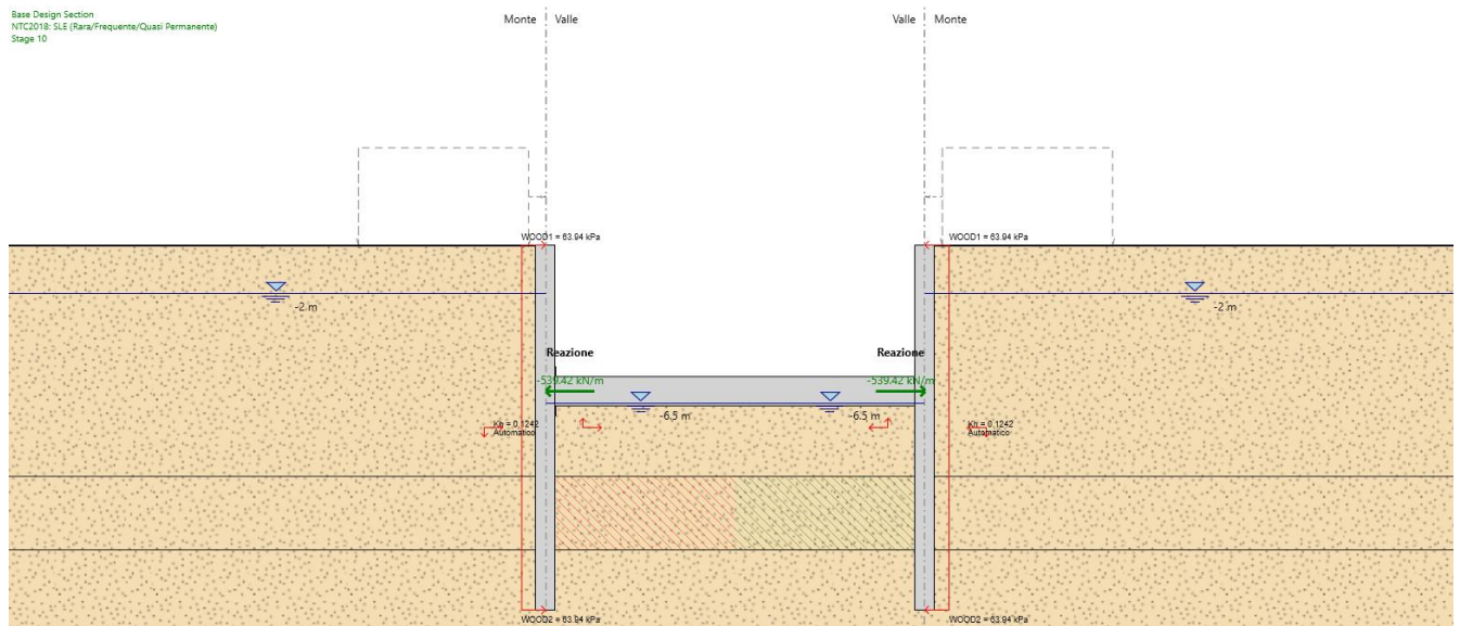
Figura 29: Involuppo delle reazioni vincolari allo SLU/SLV (tutte le fasi)
