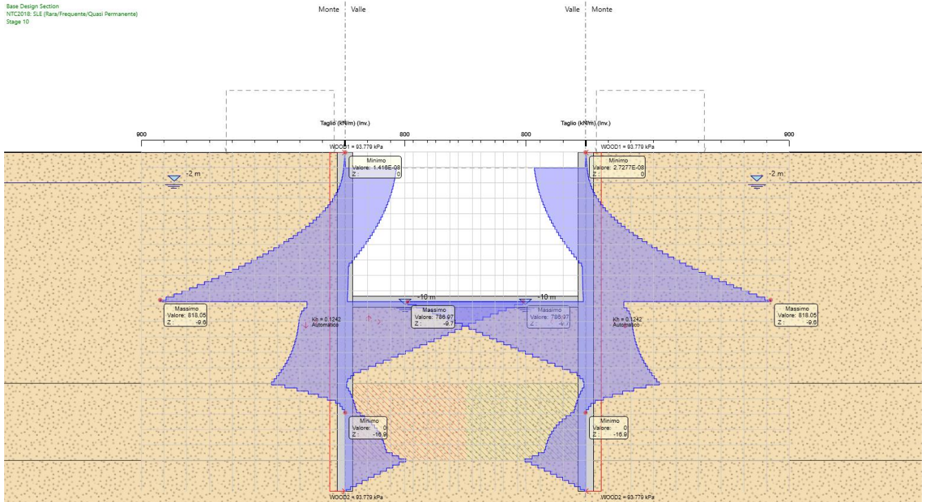
Figura 14: Involuppo del taglio agli SLU/SLV (per tutti gli stage)
