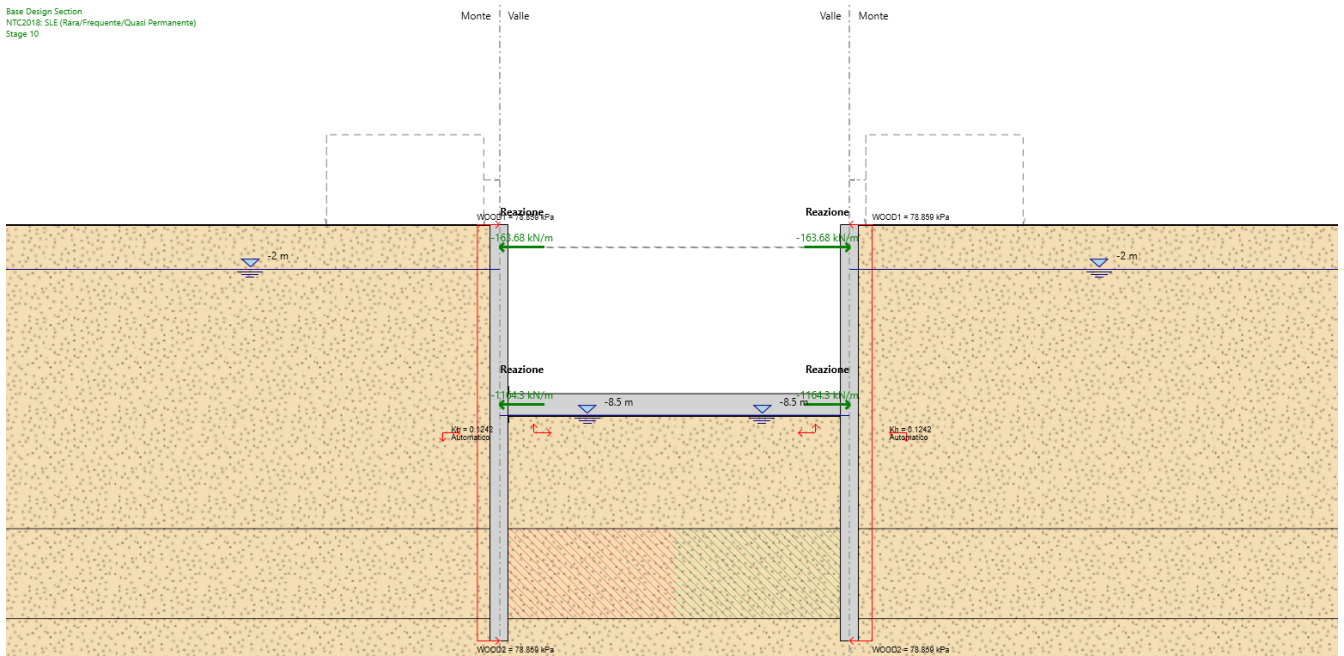
Figura 23: Involuppo delle reazioni vincolari allo SLU/SLV (tutte le fasi)
