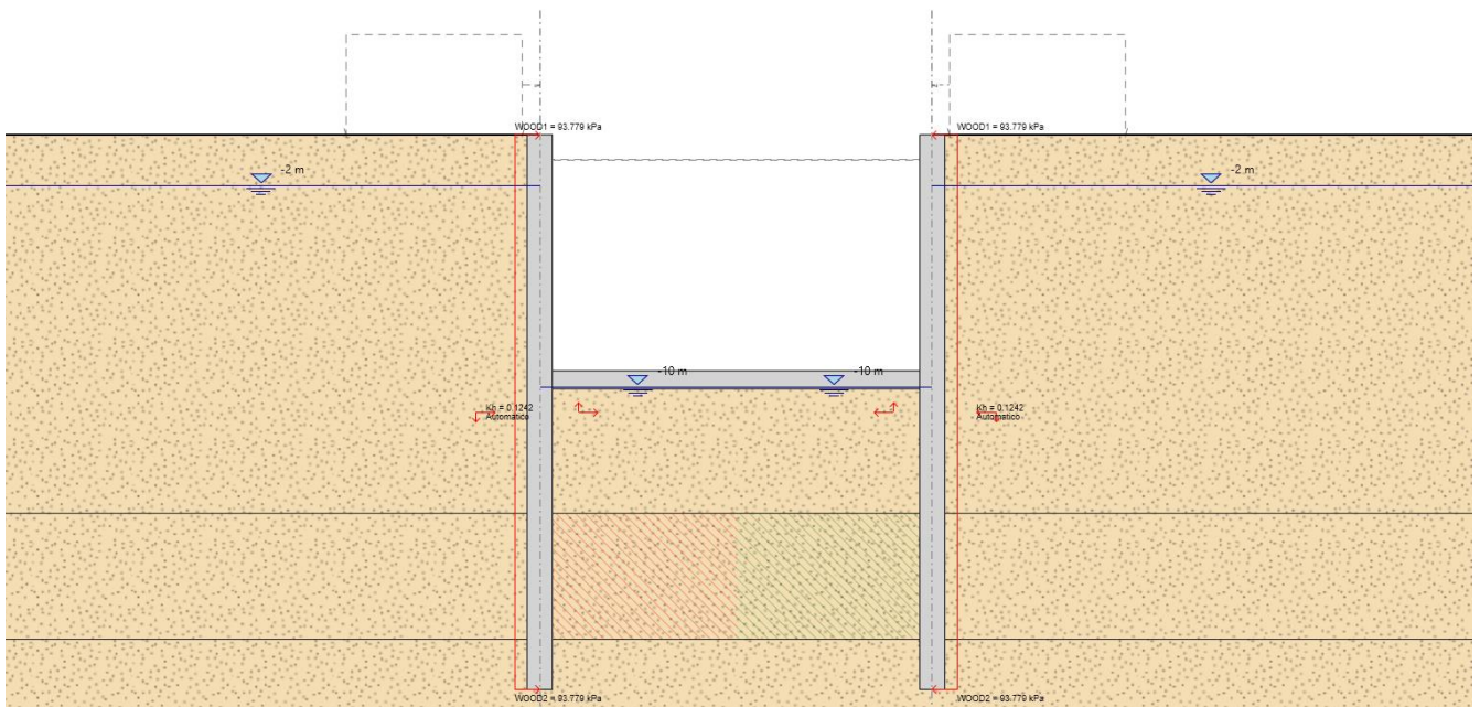
Figura 10: Fasi realizzative: Fase 6
