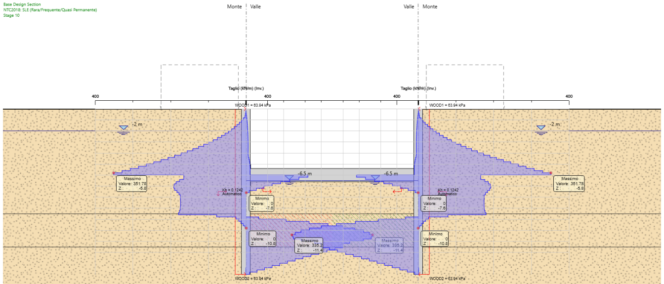
Figura 26: Involuppo del taglio agli SLU/SLV (per tutti gli stage)
