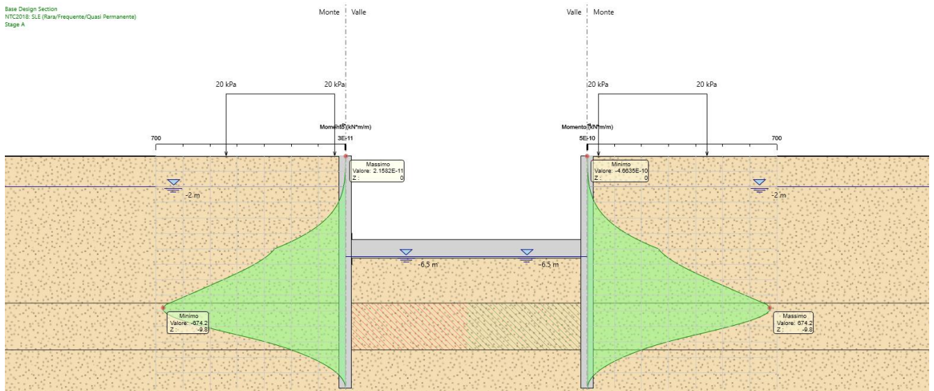
Figura 27: Diagramma dei momenti agli SLE r (in fase di esercizio)
