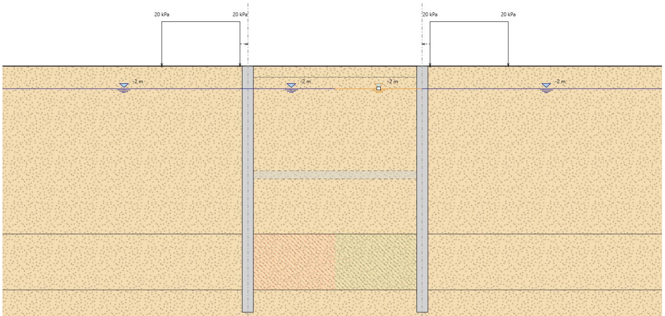
Figura 5: Fasi realizzative: Fase 1
