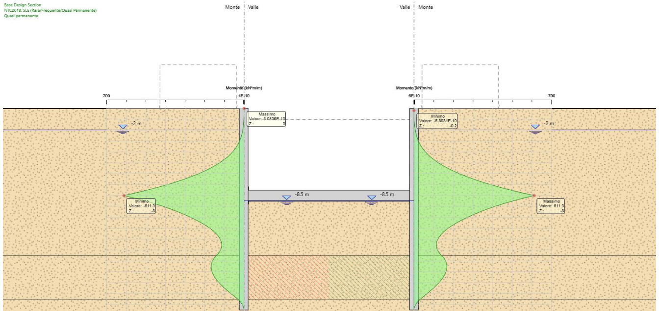
Figura 22: Diagramma dei momenti agli SLE qp (in fase di esercizio)
