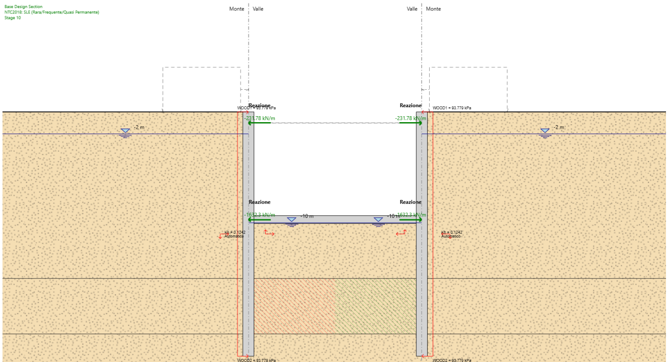
Figura 16: Diagramma dei momenti agli SLE qp (in fase di esercizio)
