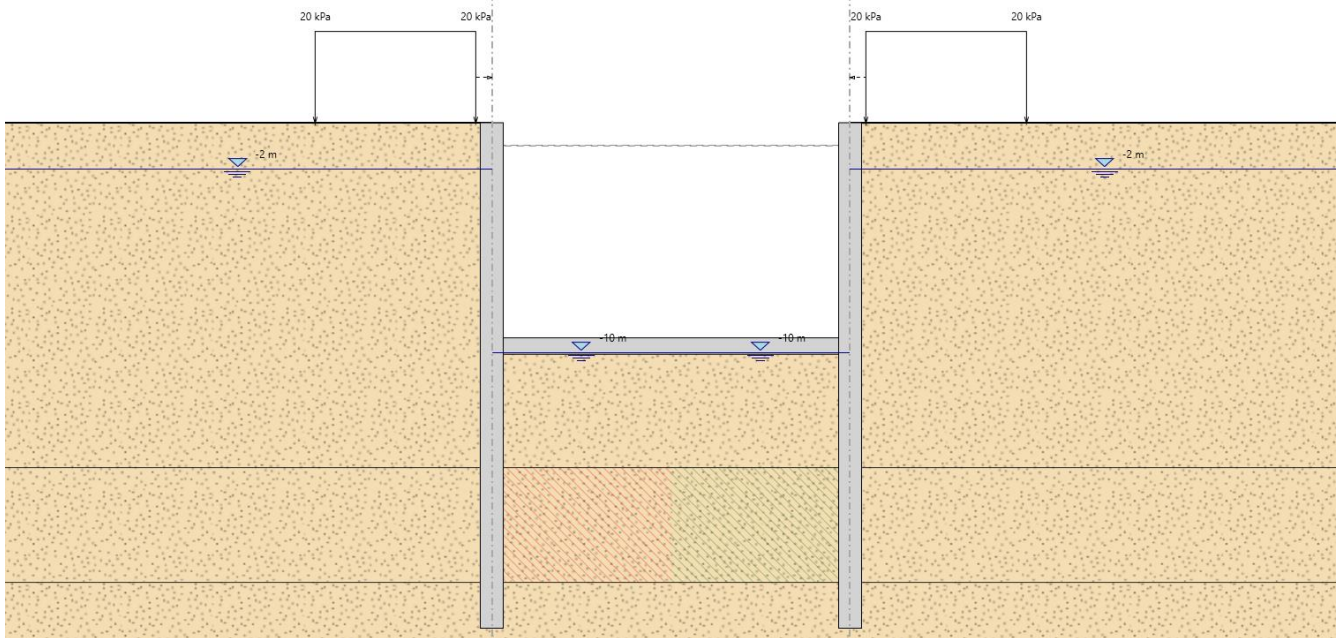
Figura 10: Fasi realizzative: Fase 6
