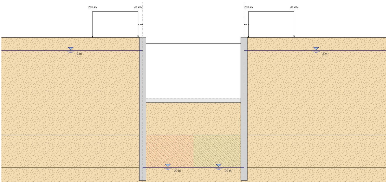
Figura 8: Fasi realizzative: Fase 4
