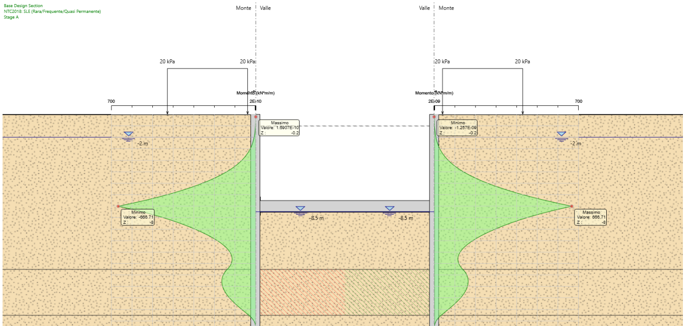
Figura 21: Diagramma dei momenti agli SLE r (in fase di esercizio)
