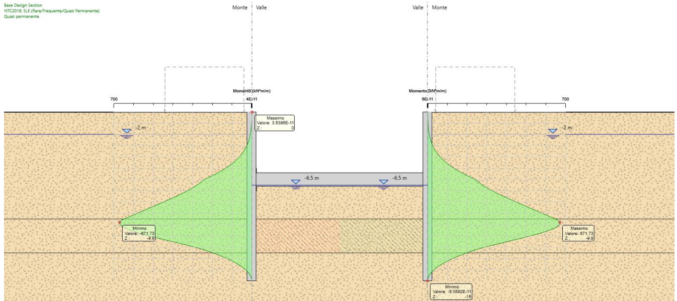
Figura 28: Diagramma dei momenti agli SLE qp (in fase di esercizio)
