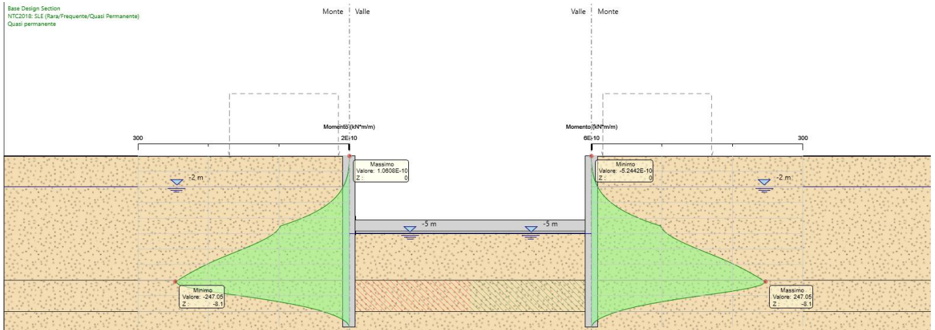
Figura 34: Diagramma dei momenti agli SLE qp (in fase di esercizio)
