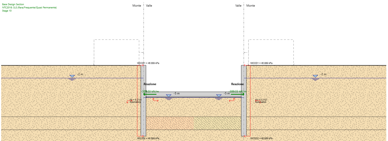
Figura 35: Involuppo delle reazioni vincolari allo SLU/SLV (tutte le fasi)
