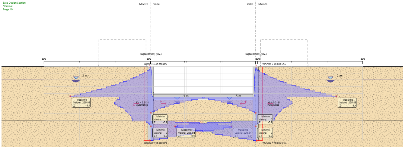
Figura 32: Involuppo del taglio agli SLU/SLV (per tutti gli stage)
