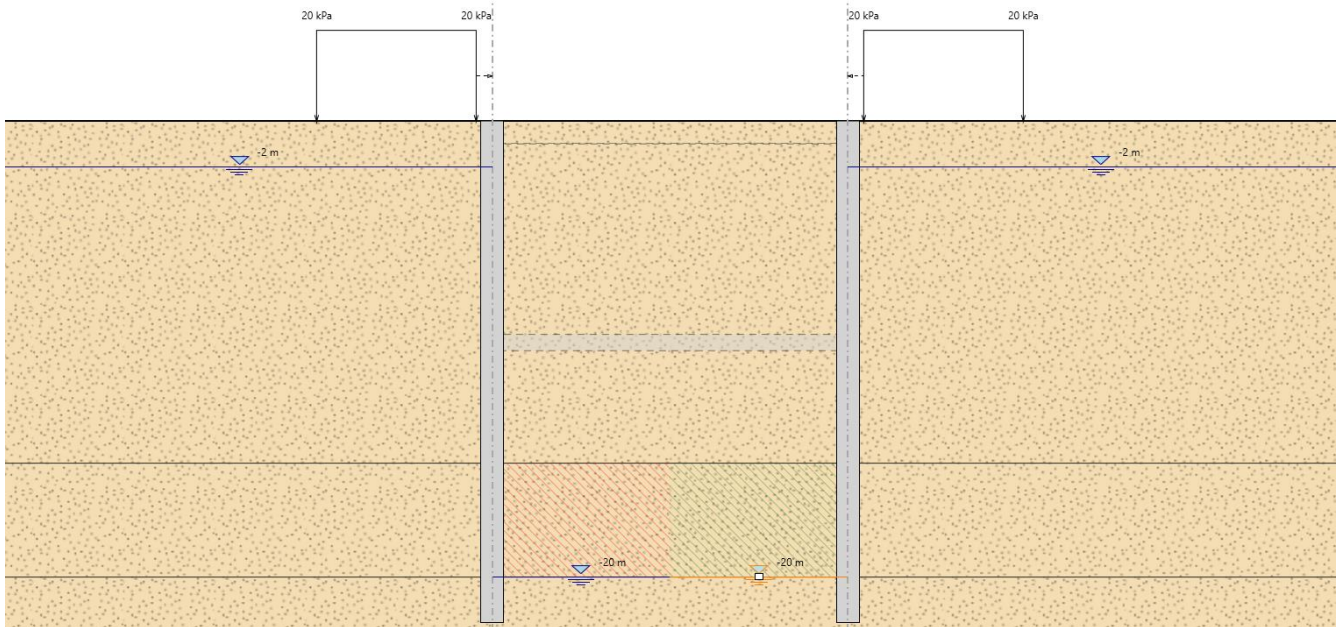
Figura 6: Fasi realizzative: Fase 2
