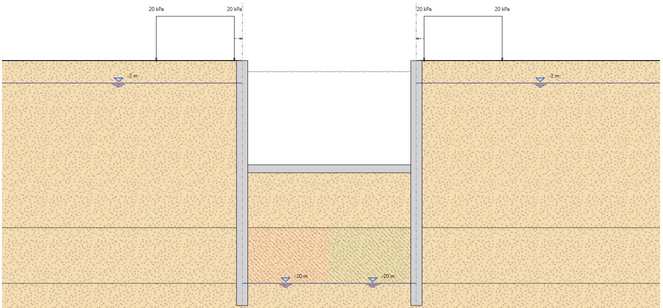
Figura 9: Fasi realizzative: Fase 5
