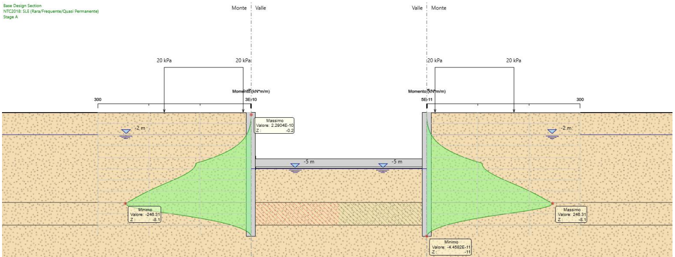
Figura 33: Diagramma dei momenti agli SLE r (in fase di esercizio)
