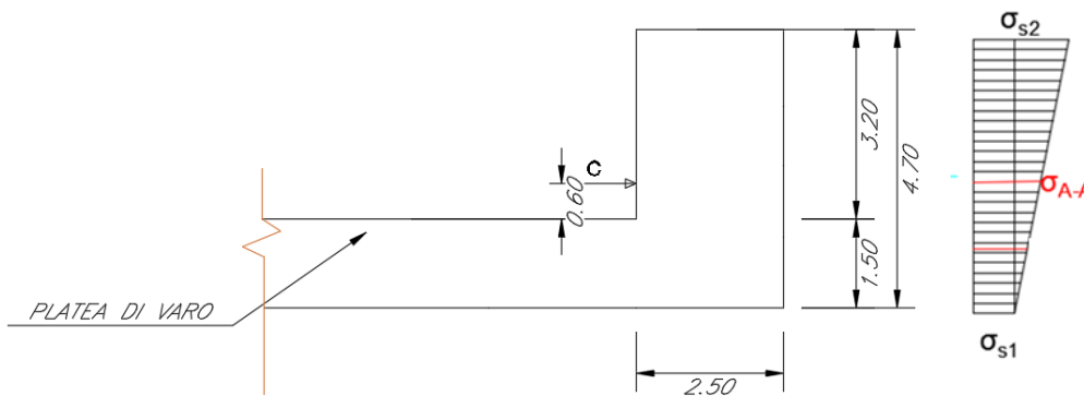
Figura 37 Schema di calcolo armature verticali
