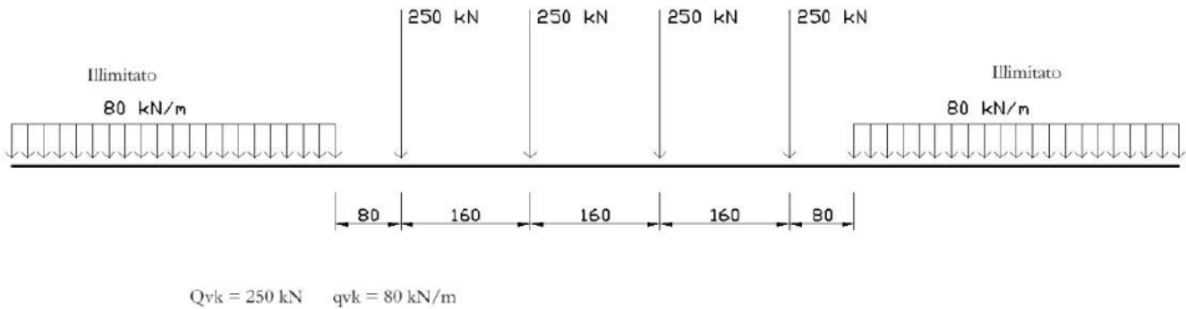
Figura 10: Treno di carico LM71
