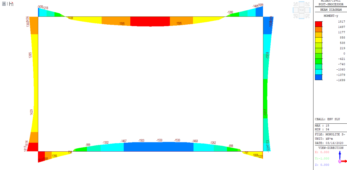
Figura 22: Involuppo M – SLU
