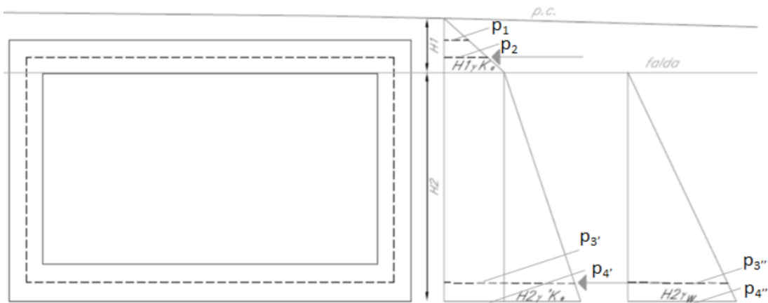
Figura 8: Spinte del terreno (si fa presente che il disegno è da prendere come esempio e spiega le azioni agenti, la quota di falda nel nostro caso è più bassa e sono presenti due strati aventi caratteristiche diverse lungo l'altezza del monolite)
