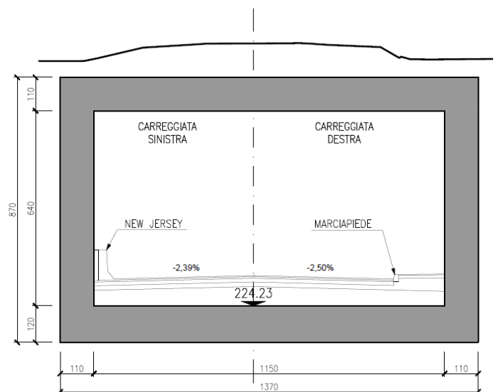
Figura 3: Geometria dell'opera
