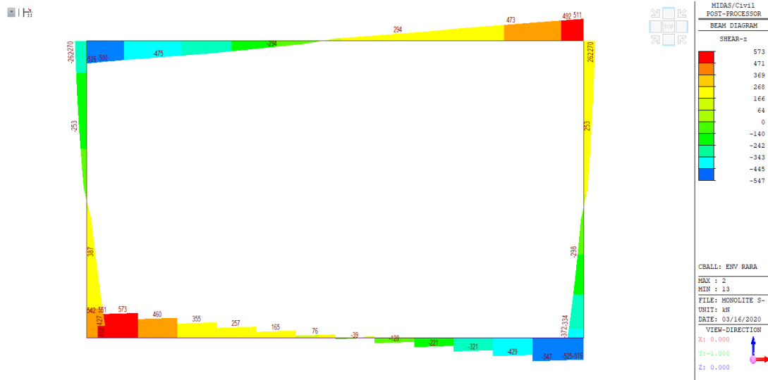
Figura 27: Involuppo V – SLE RARA
