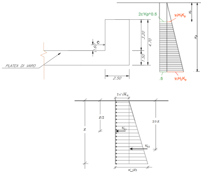
Figura 13.19 – Diagramma di spinta passiva in un terreno dotato di coesione e attrito
