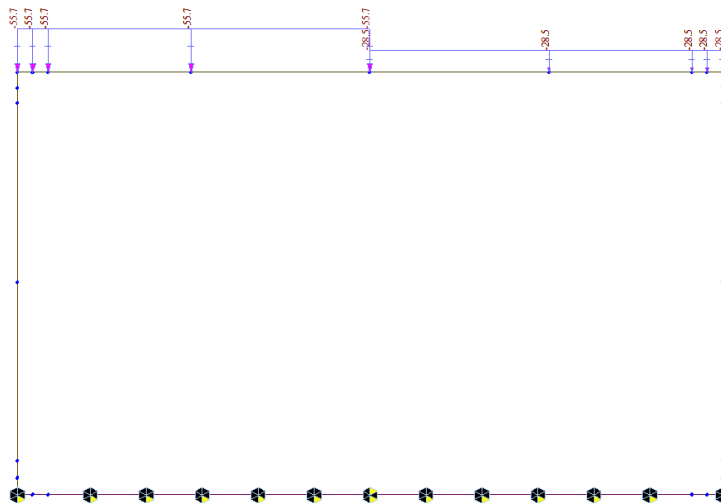
Figura 13: Carichi Treno LM71 condizione Taglio massimo ACC2
