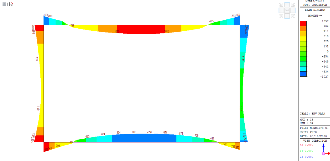
Figura 28: Inviluppo M – SLE RARA
