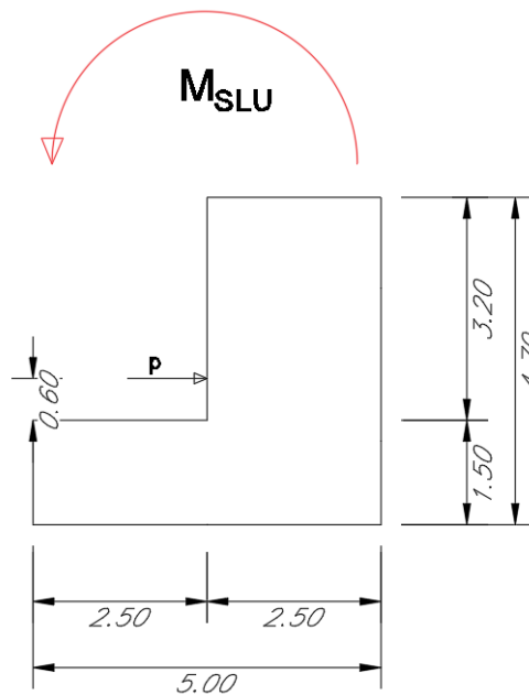
Figura 36 – Azione di momento agente sulla sezione a T
