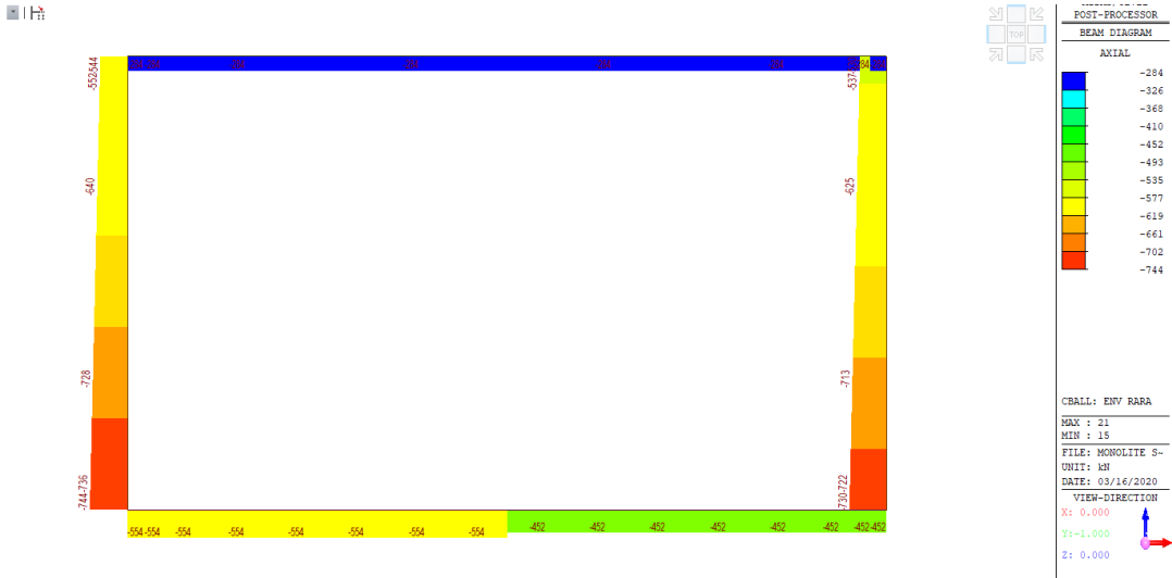
Figura 26: Involuppo N – SLE RARA
