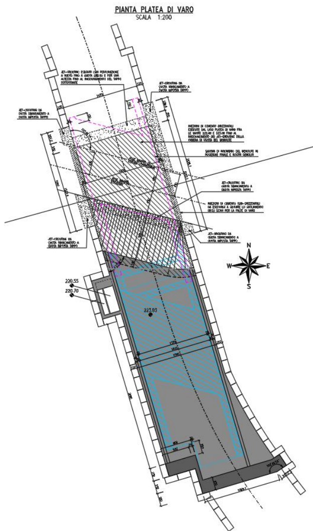
Figura 30 Pianta
