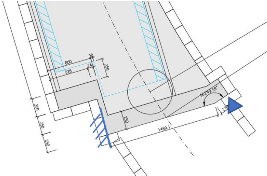
Figura 35 Trave reggispinta e condizioni di vincolo
