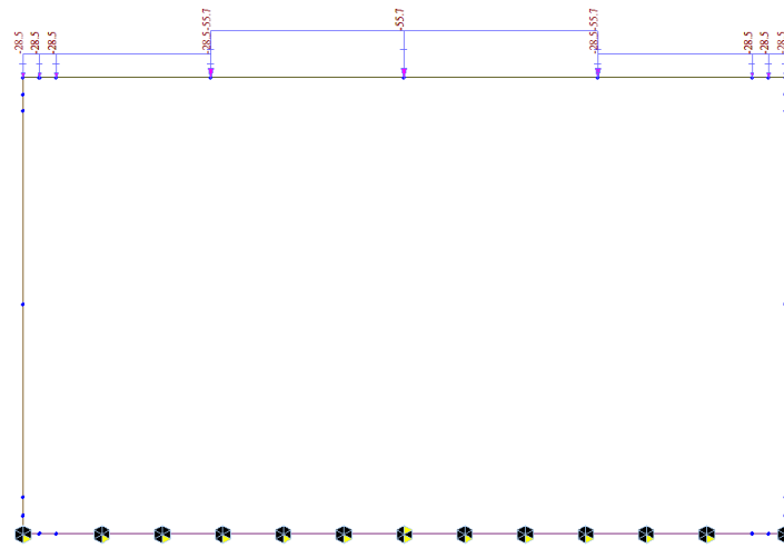
Figura 12: Carichi Treno LM71 condizione Momento massimo ACC1
