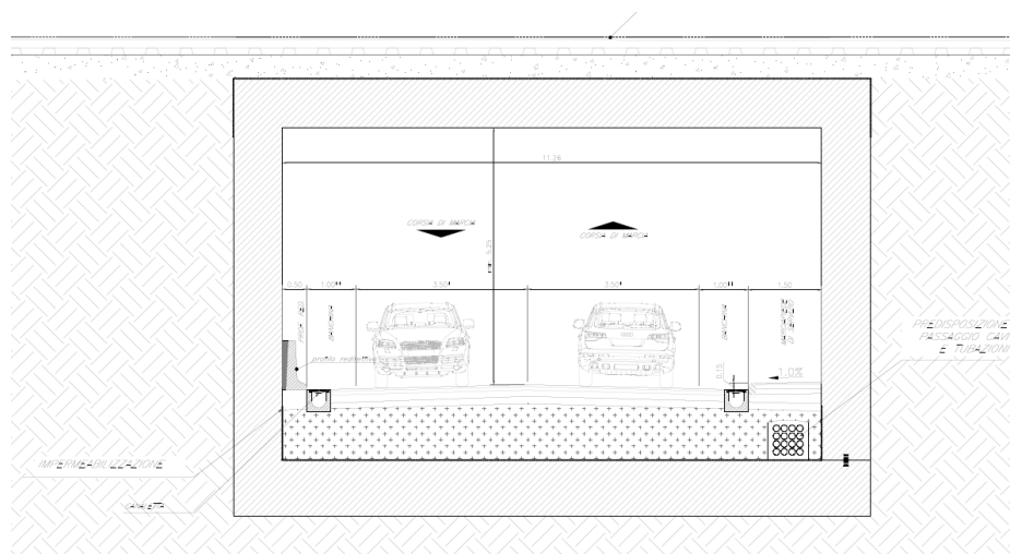
Figura 1: Sezione trasversaleschematica dello scatolare con dimensioni "di calcolo"
