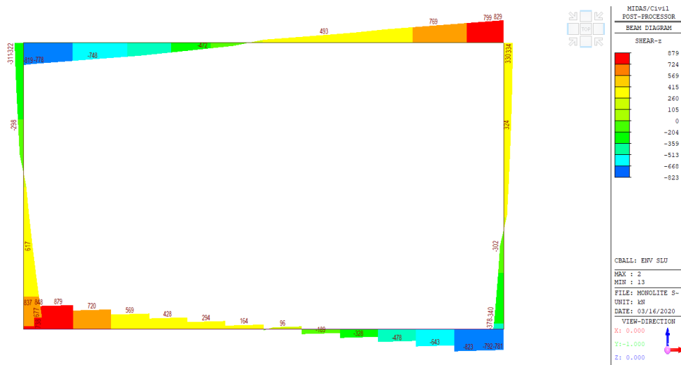
Figura 21: Inviluppo T - SLU
