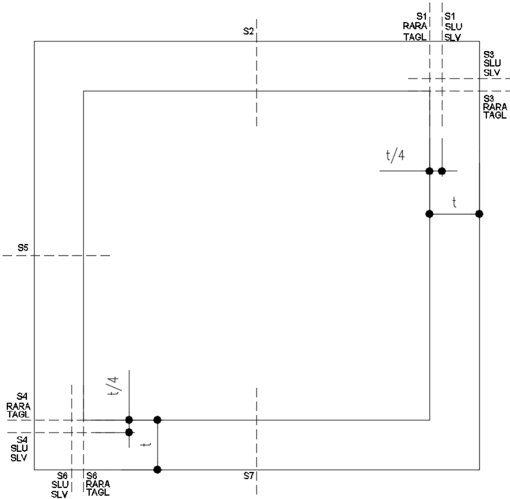
Figura 29: Sezioni di verifica
