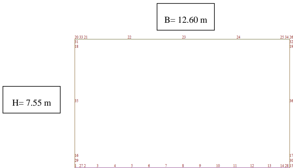
Figura 4: Numerazione dei nodi nel modello strutturale
