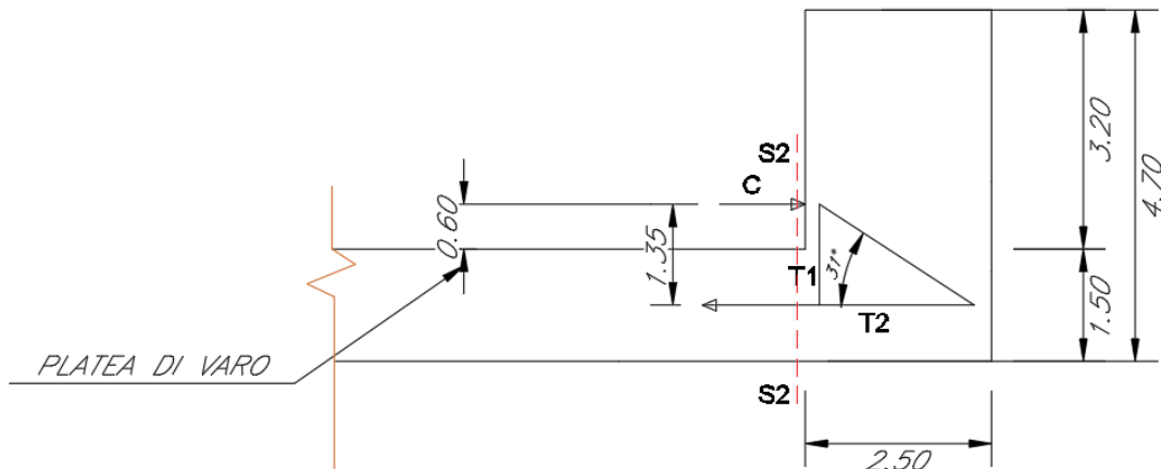
Figura 32 Sollecitazioni agenti all'interno del muro reggispinta in corrispondenza della sezione S2 nella platea di varo.
