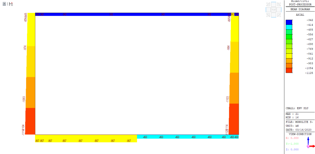
Figura 20: Inviluppo N – SLU
