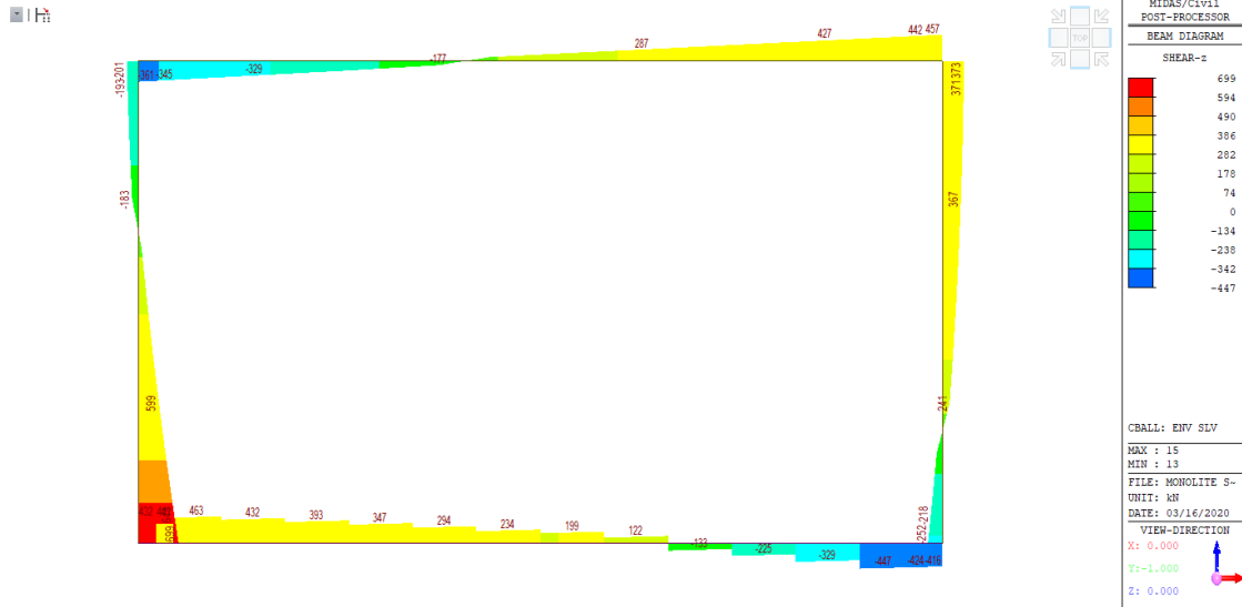
Figura 24: Inviluppo T - SLV
