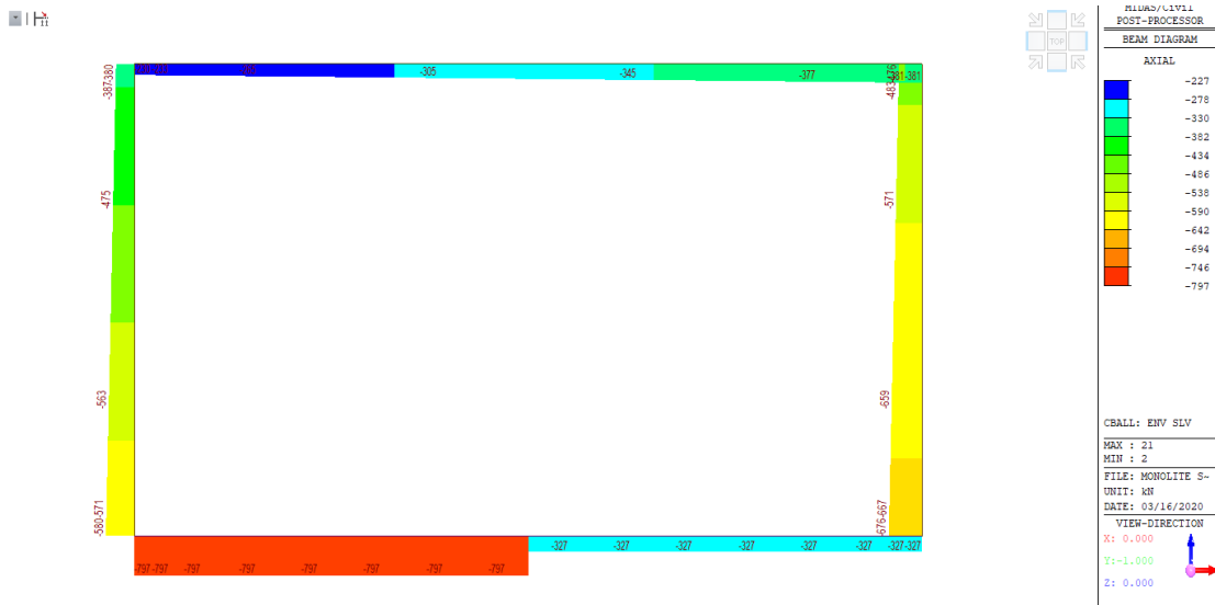
Figura 23: Involuppo N - SLV
