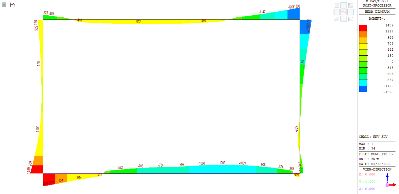
Figura 25: Inviluppo M - SLV
