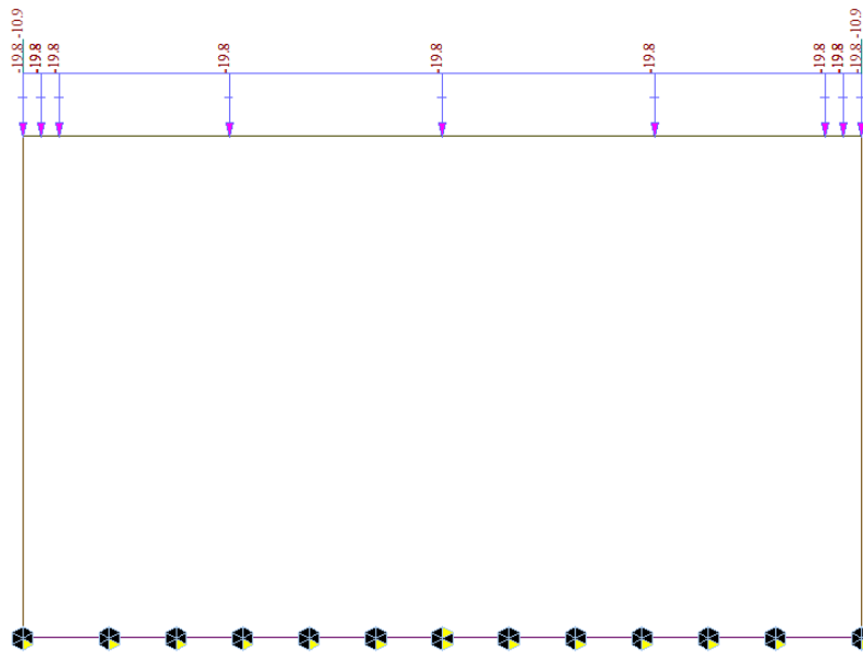
Figura 7: Carico permanente verticale ballast
