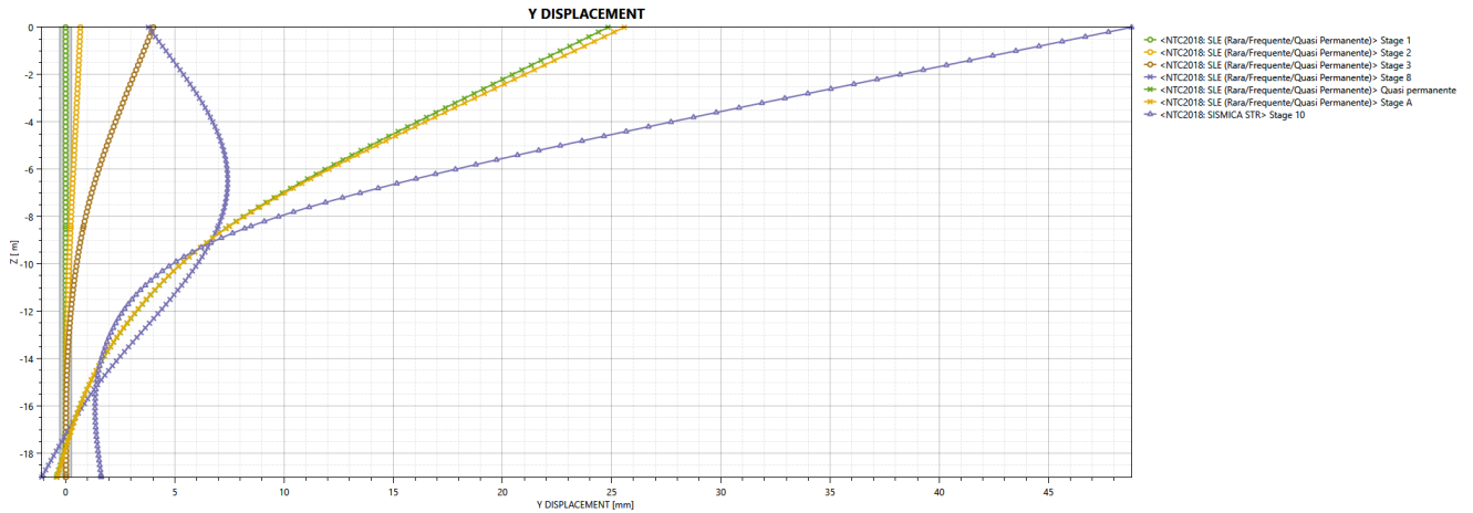
Figura 18: Spostamenti nominali della paratia nelle principali fasi
