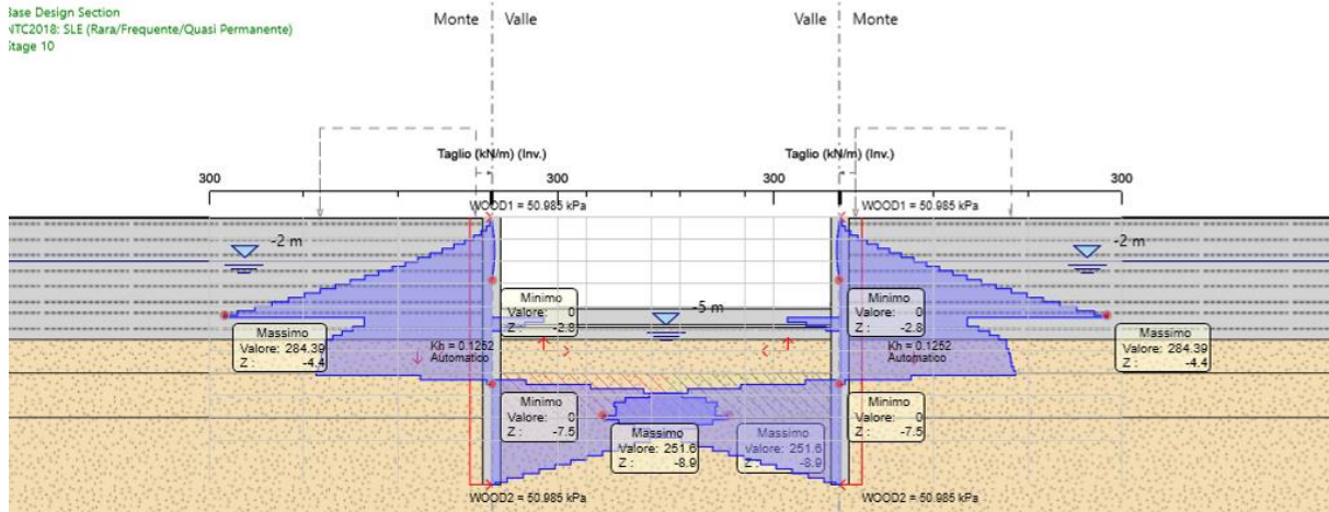
Figura 32: Inviluppo del taglio agli SLU/SLV (per tutti gli stage)
