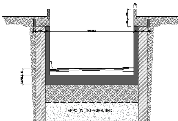
Figura 1: Sezione trasversale tipo con arredo
