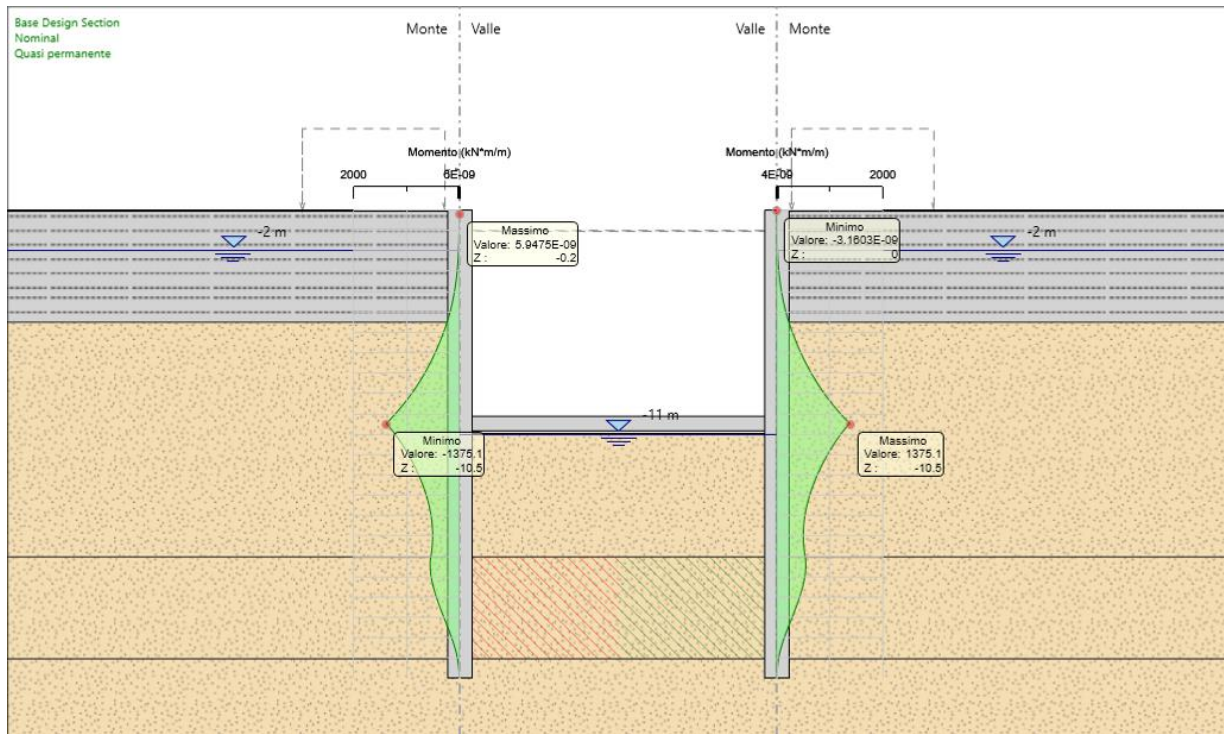
Figura 16: Diagramma dei momenti agli SLE qp (in fase di esercizio)
