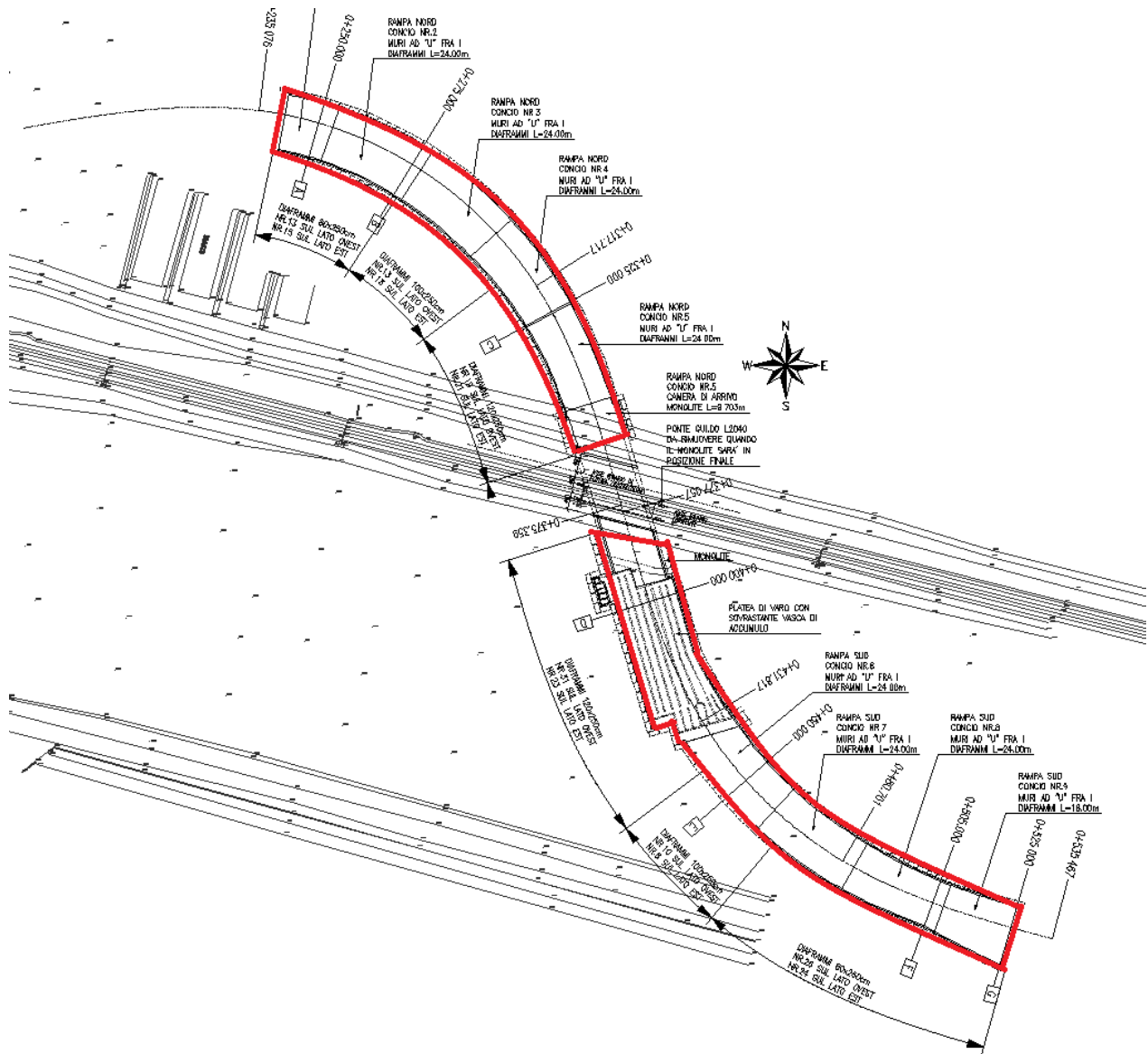
Figura 2: planimetria generale del sottopasso SL03 con il tratto interessato evidenziato
