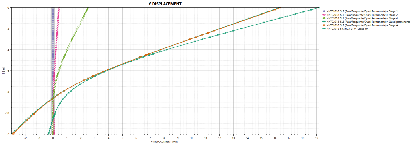
Figura 30: Spostamenti nominali della paratia nelle principali fasi
