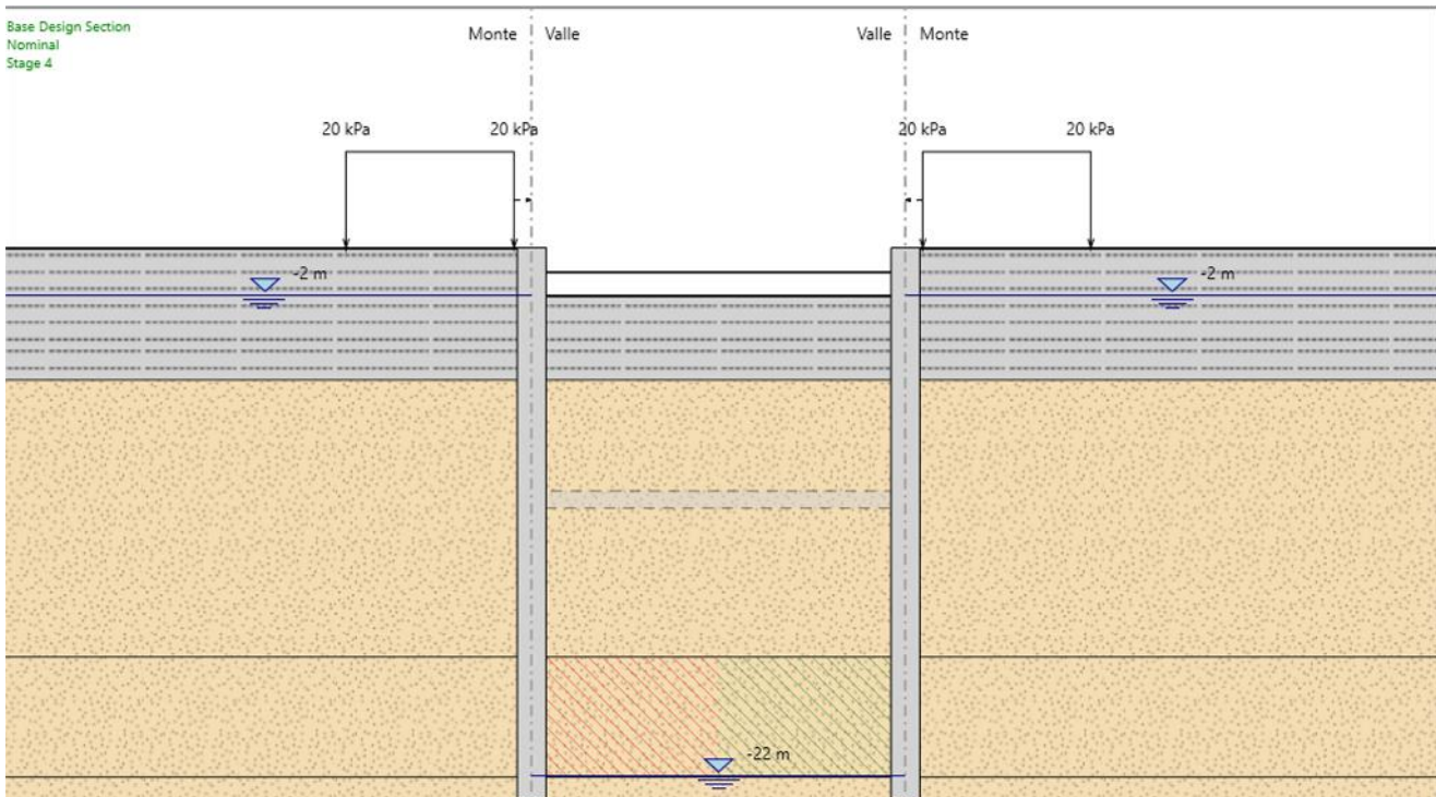
Figura 7: Fasi realizzative: Fase 3
