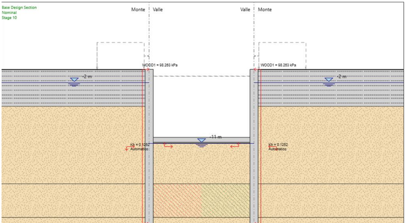
Figura 11: Fasi realizzative: Fase 7
