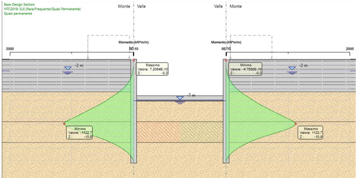
Figura 28: Diagramma dei momenti agli SLE qp (in fase di esercizio)
