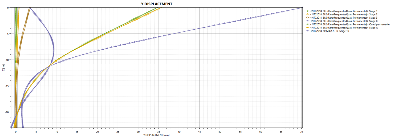
Figura 12: Spostamenti nominali della paratia nelle principali fasi
