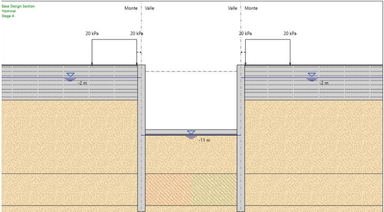
Figura 10: Fasi realizzative: Fase 6
