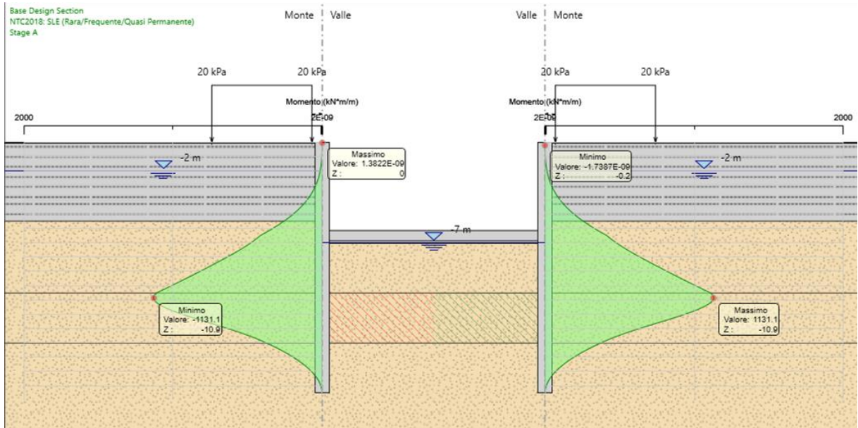
Figura 27: Diagramma dei momenti agli SLE r (in fase di esercizio)
