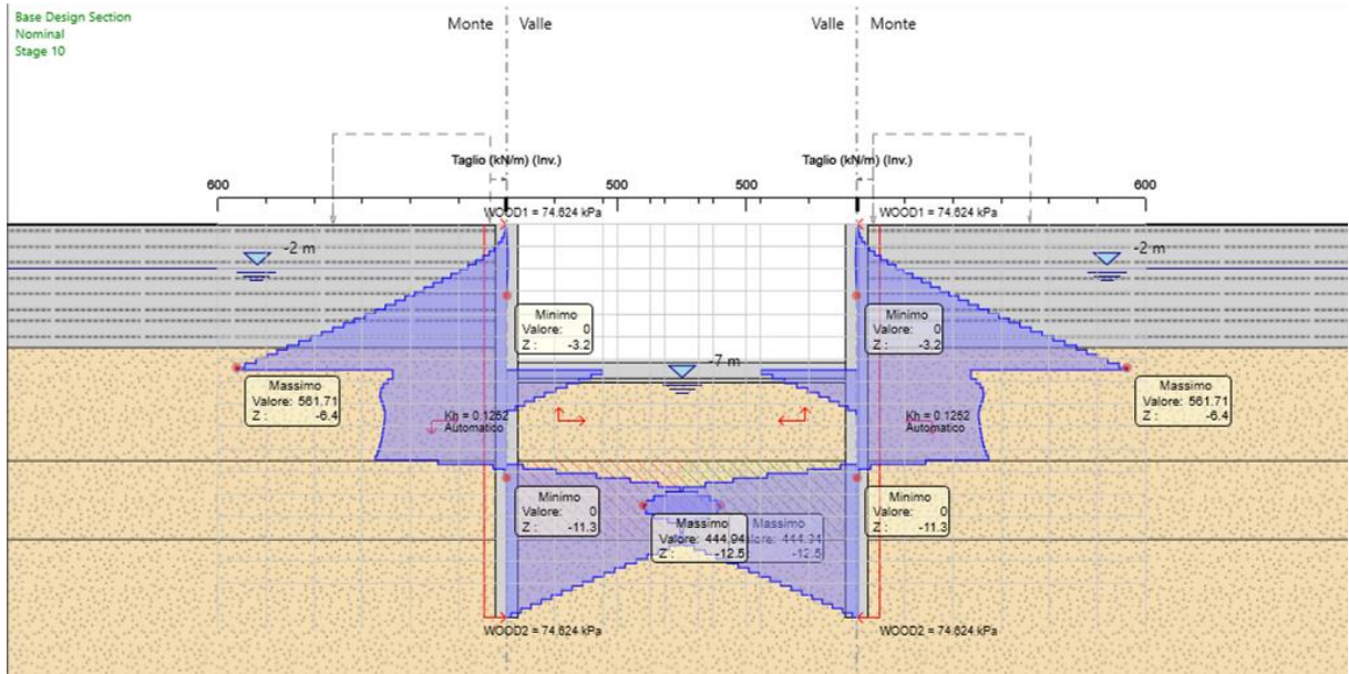
Figura 26: Involuppo del taglio agli SLU/SLV (per tutti gli stage)
