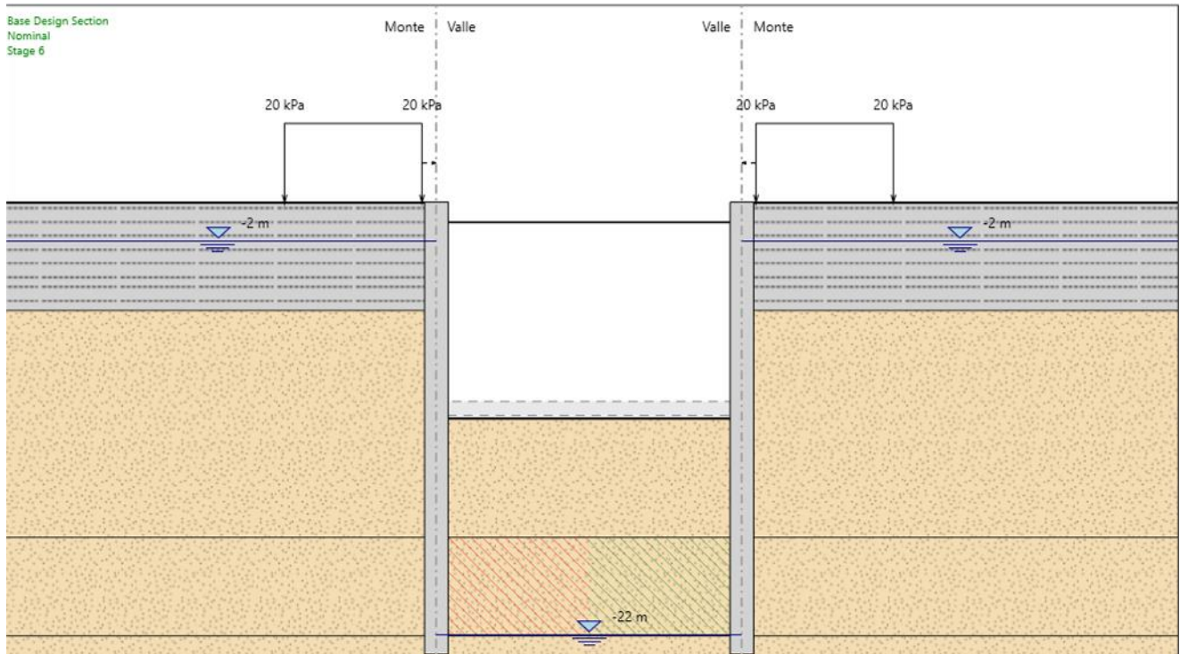
Figura 8: Fasi realizzative: Fase 4
