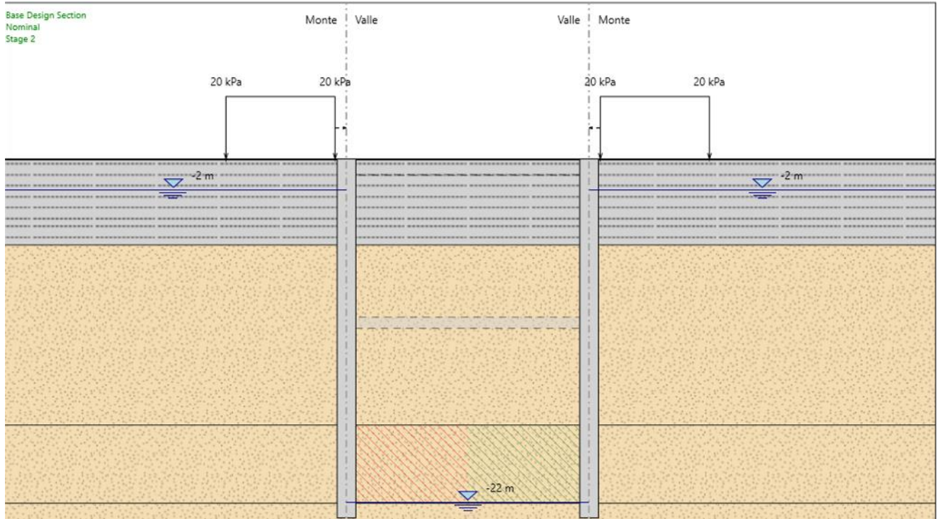
Figura 6: Fasi realizzative: Fase 2
