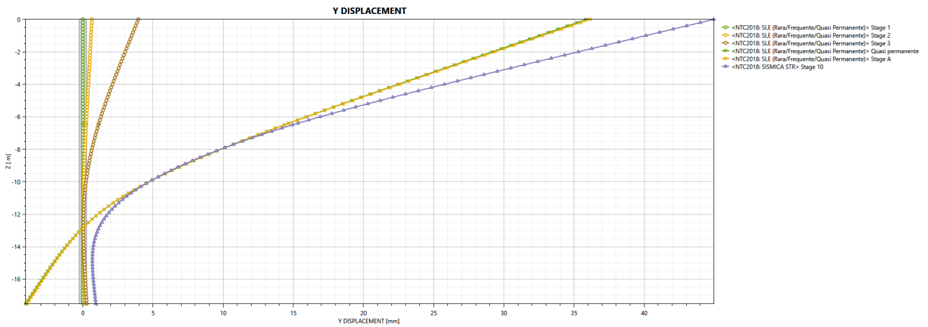
Figura 24: Spostamenti nominali della paratia nelle principali fasi
