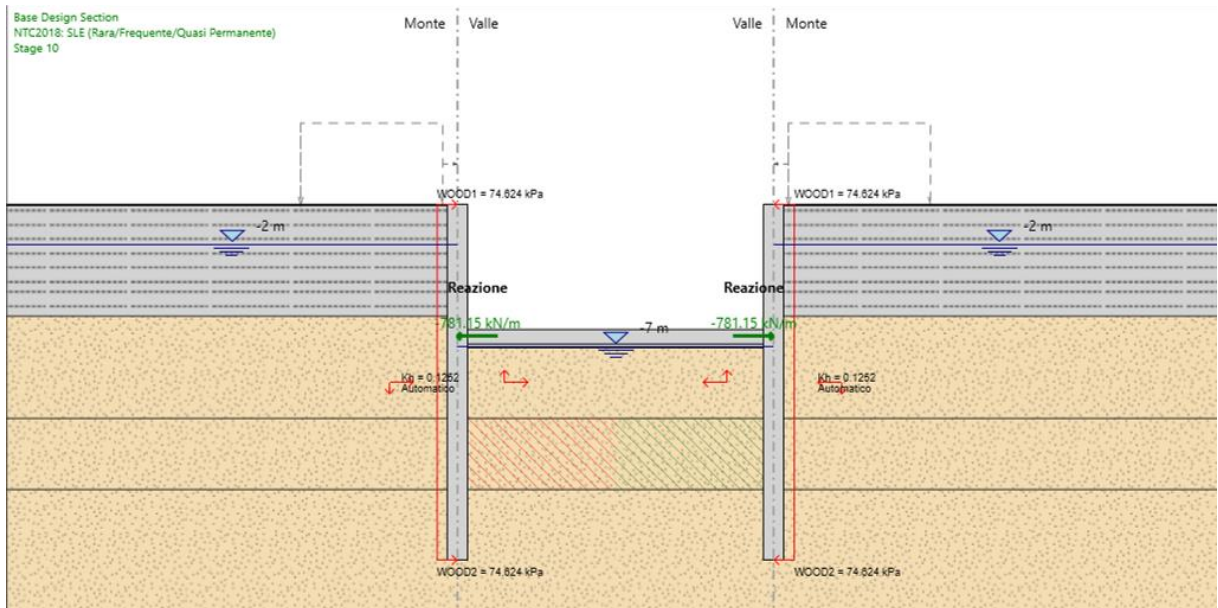
Figura 29: Involuppo delle reazioni vincolari allo SLU/SLV (tutte le fasi)
