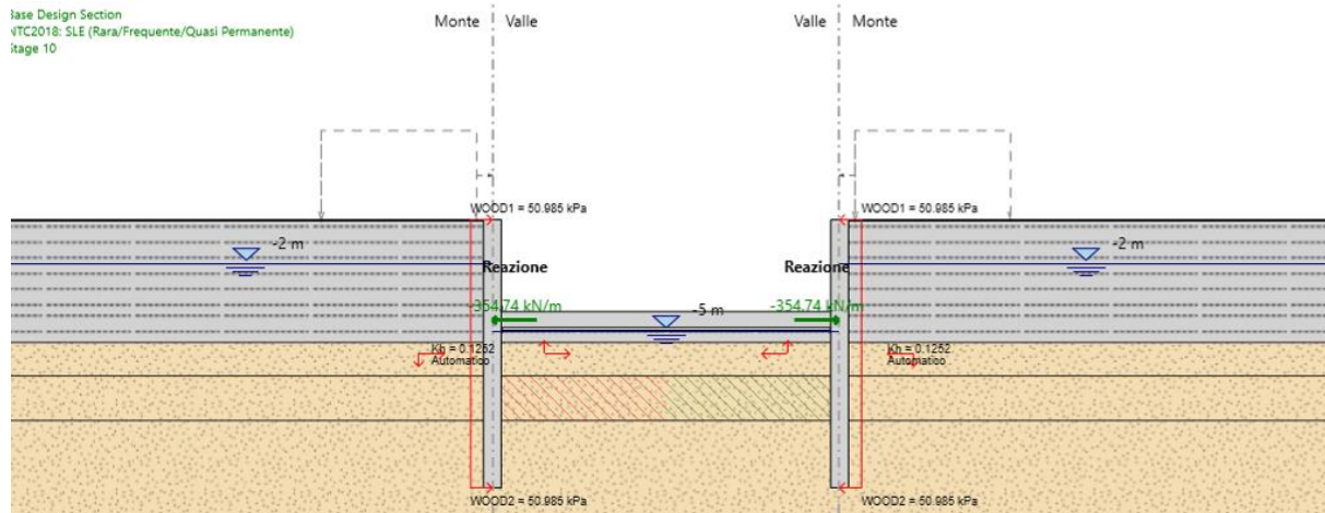
Figura 35: Involuppo delle reazioni vincolari allo SLU/SLV (tutte le fasi)
