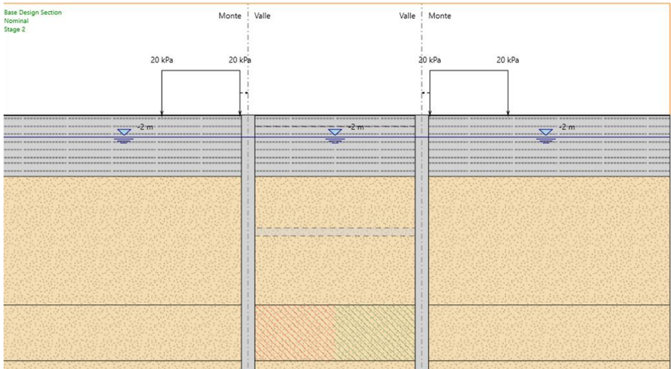
Figura 5: Fasi realizzative: Fase 1
