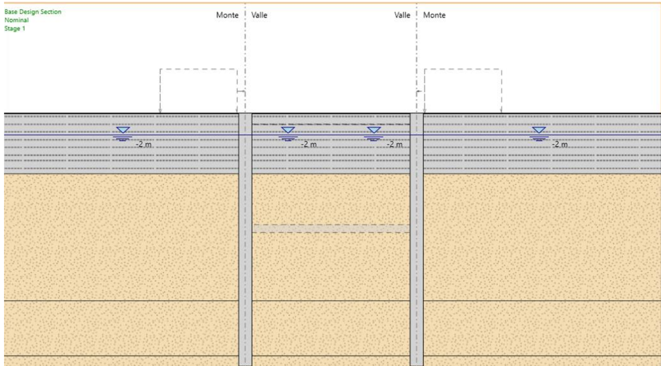
Figura 4: Fasi realizzative: Fase 0
