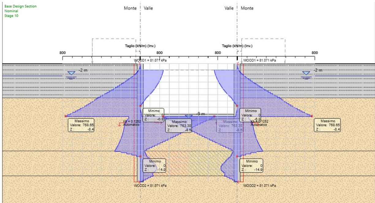
Figura 20: Involuppo del taglio agli SLU/SLV (per tutti gli stage)
