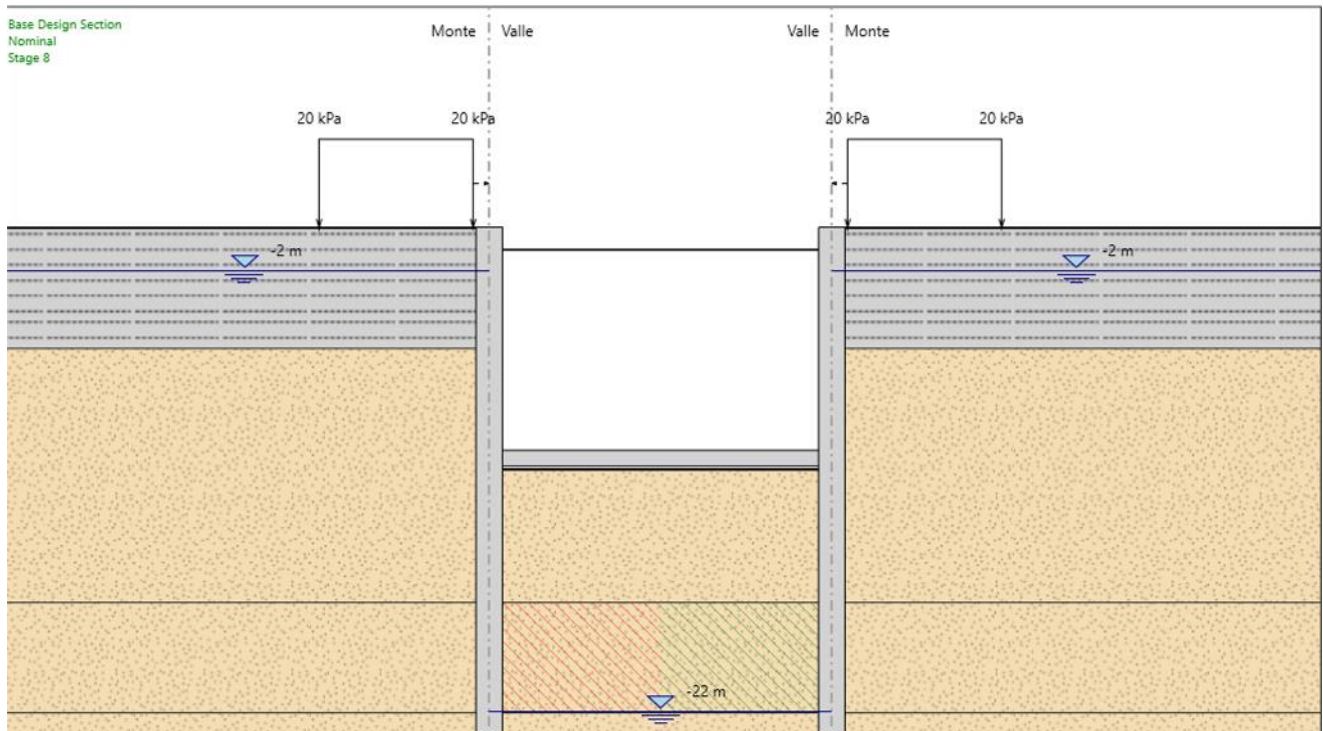
Figura 9: Fasi realizzative: Fase 5
