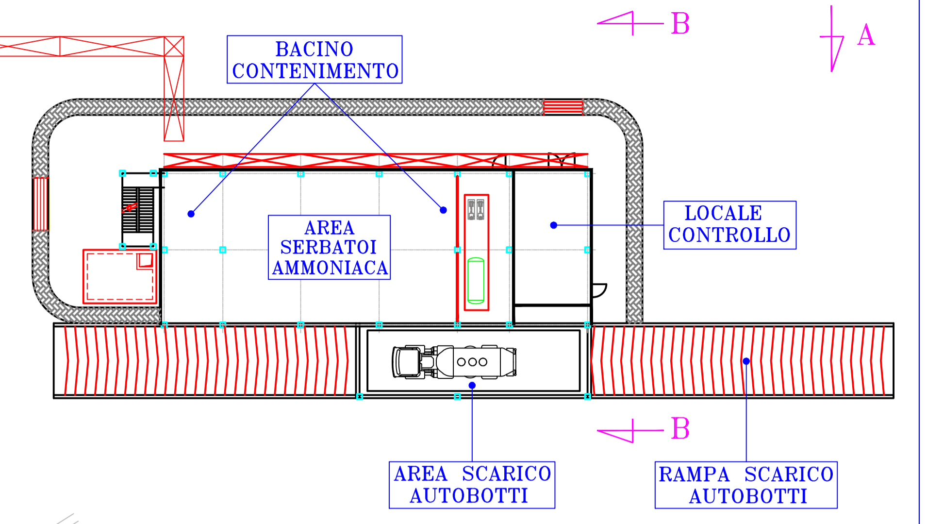
PIANTA EDIFICIO STOCCAGGIO AMMONIACA
