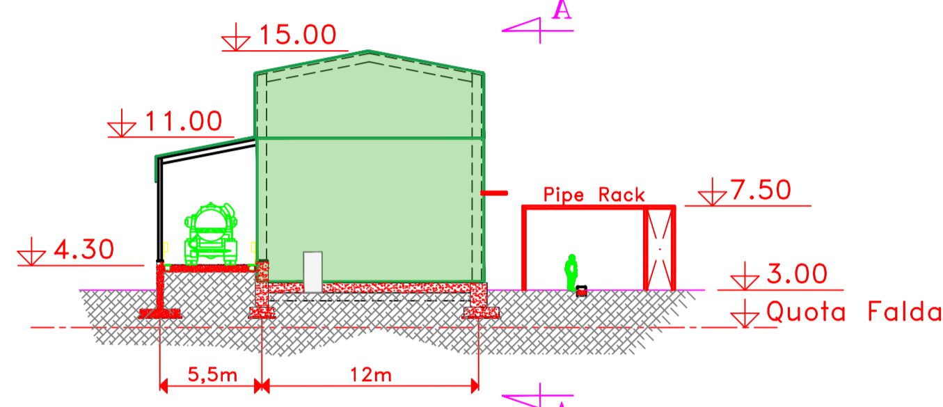
SEZIONE B-B
